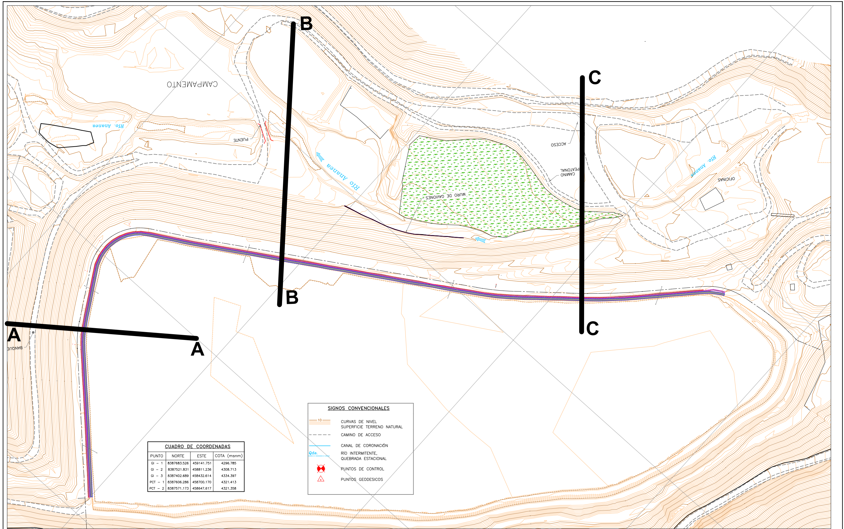
PLANTA Esc.: 1/1,000
