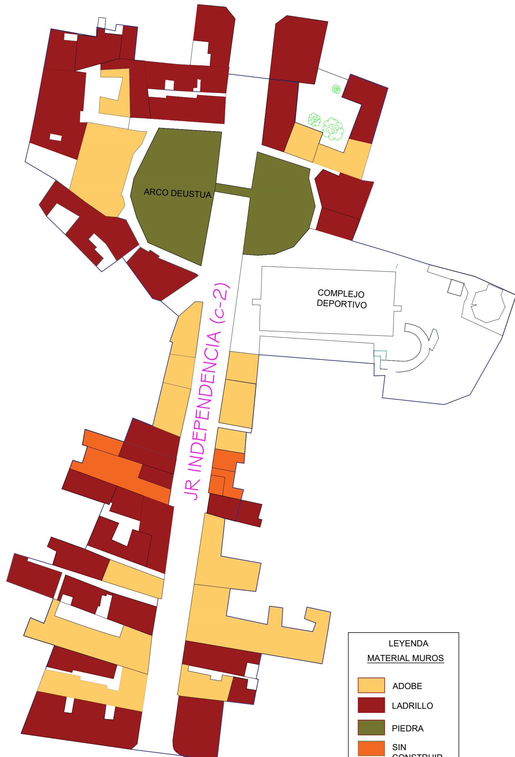
MATERIAL DE MUROS DE LAS EDIFICACIONES EN EL AMBIENTE URBANO MONUMENTAL ARCO DEUSTUA
