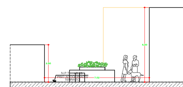
CORTE I-I Jr. 2 DE MAYO
