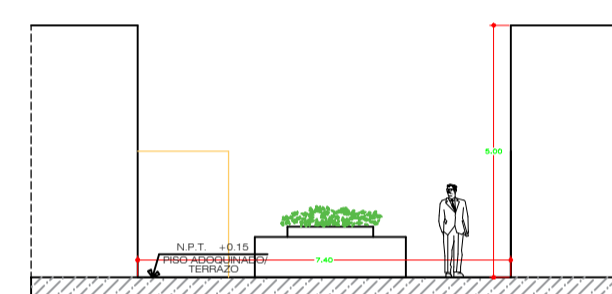
CORTE K-K Jr. 2 DE MAYO
