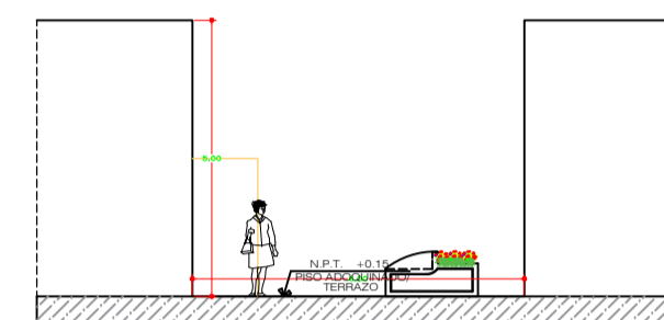
CORTE H-H Jr. 28 DE JULIO
