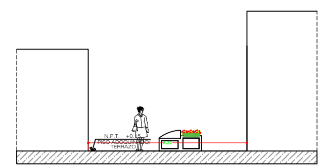
CORTE A-A CALLE PUNO
