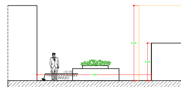
CORTE G-G Jr. 28 DE JULIO
