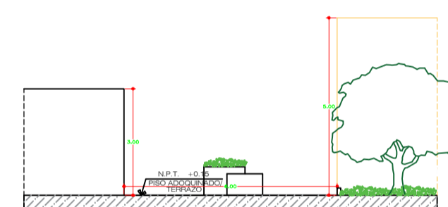
CORTE L-L JIRON CUSCO
