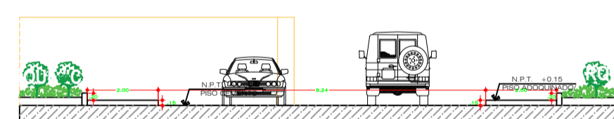
CORTE N-N CALLE SAN ROMAN
