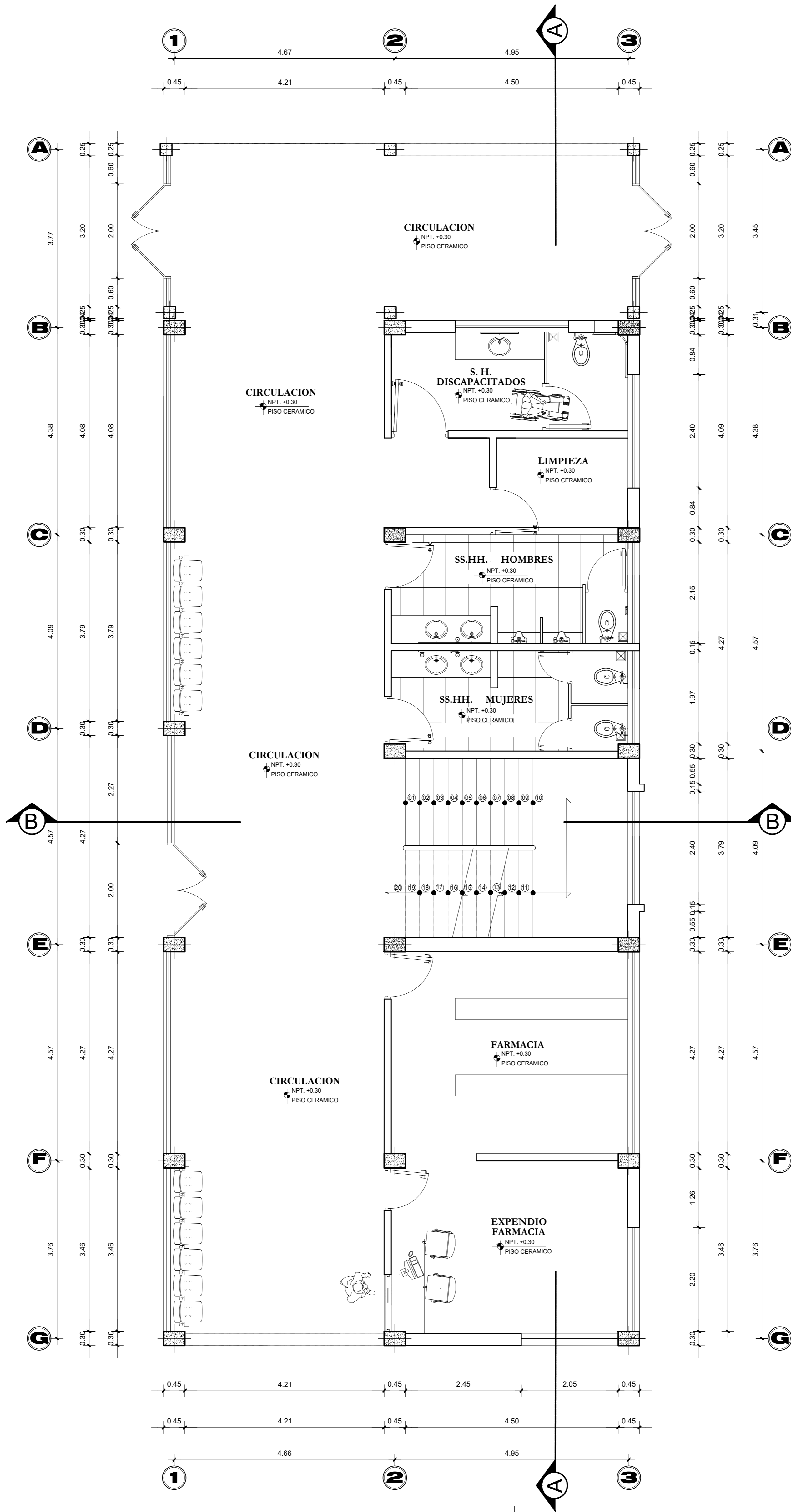
1° NIVEL UNIDAD DE ADMINISTRACION Escala 1:50
