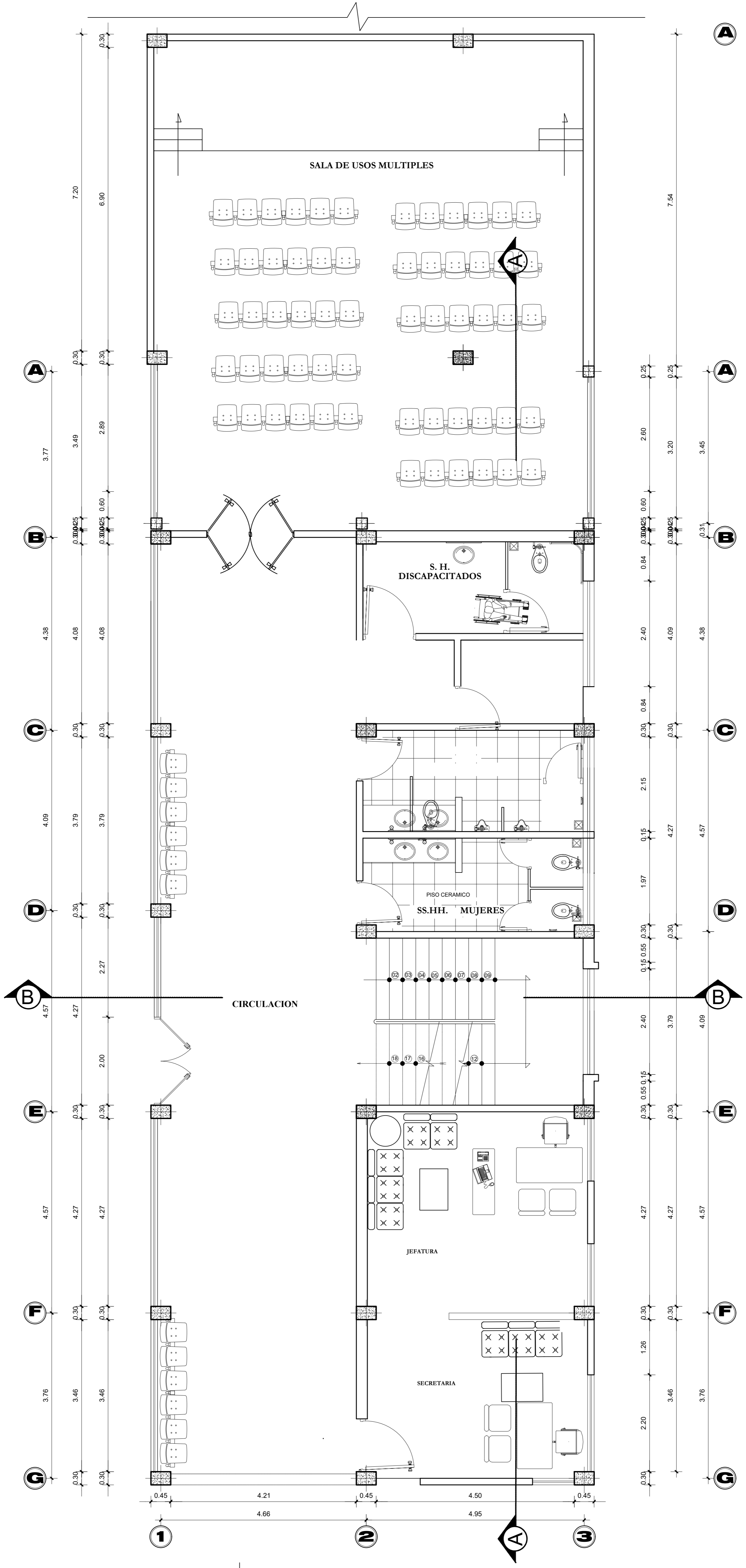
2° NIVEL UNIDAD DE ADMINISTRACION Escala 1:50
