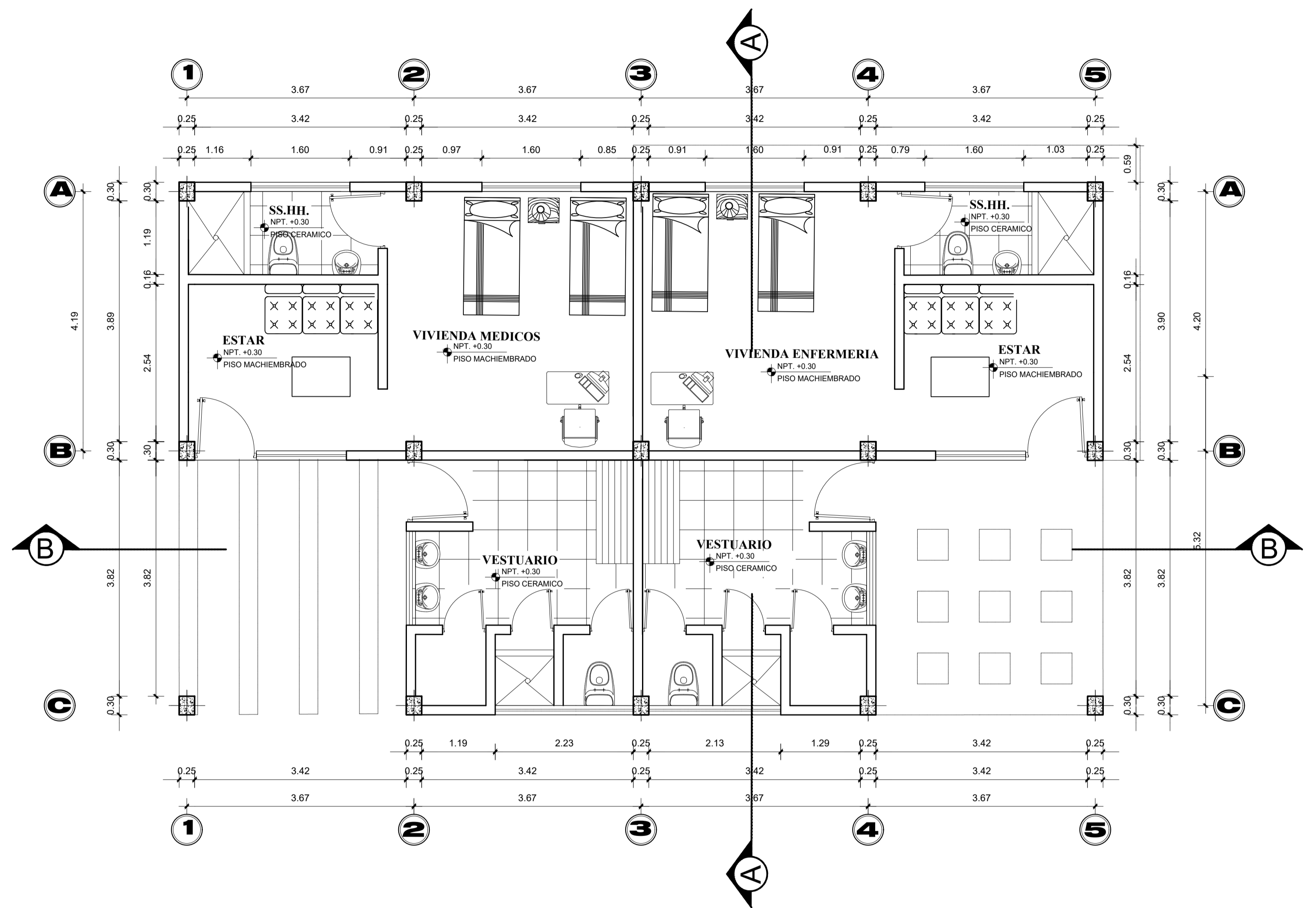
PLANTA-UNIDAD DE VIVIENDA Escala 1:50
