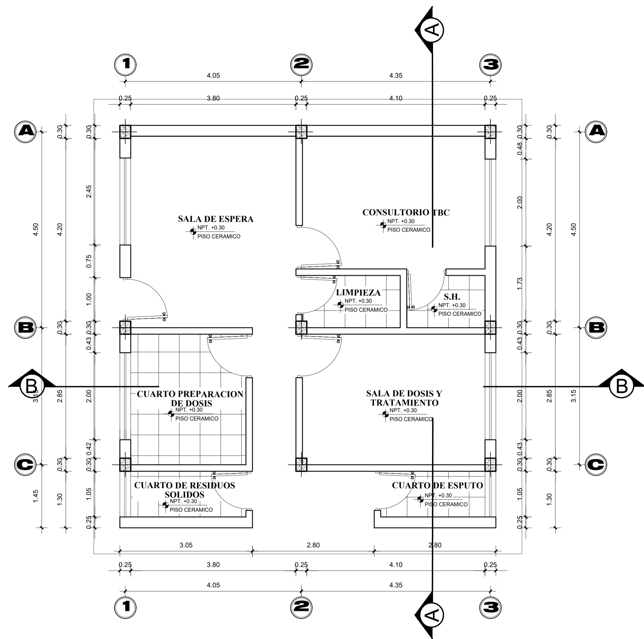
PLANTA-UNIDAD DE TBC Escala 1:50
