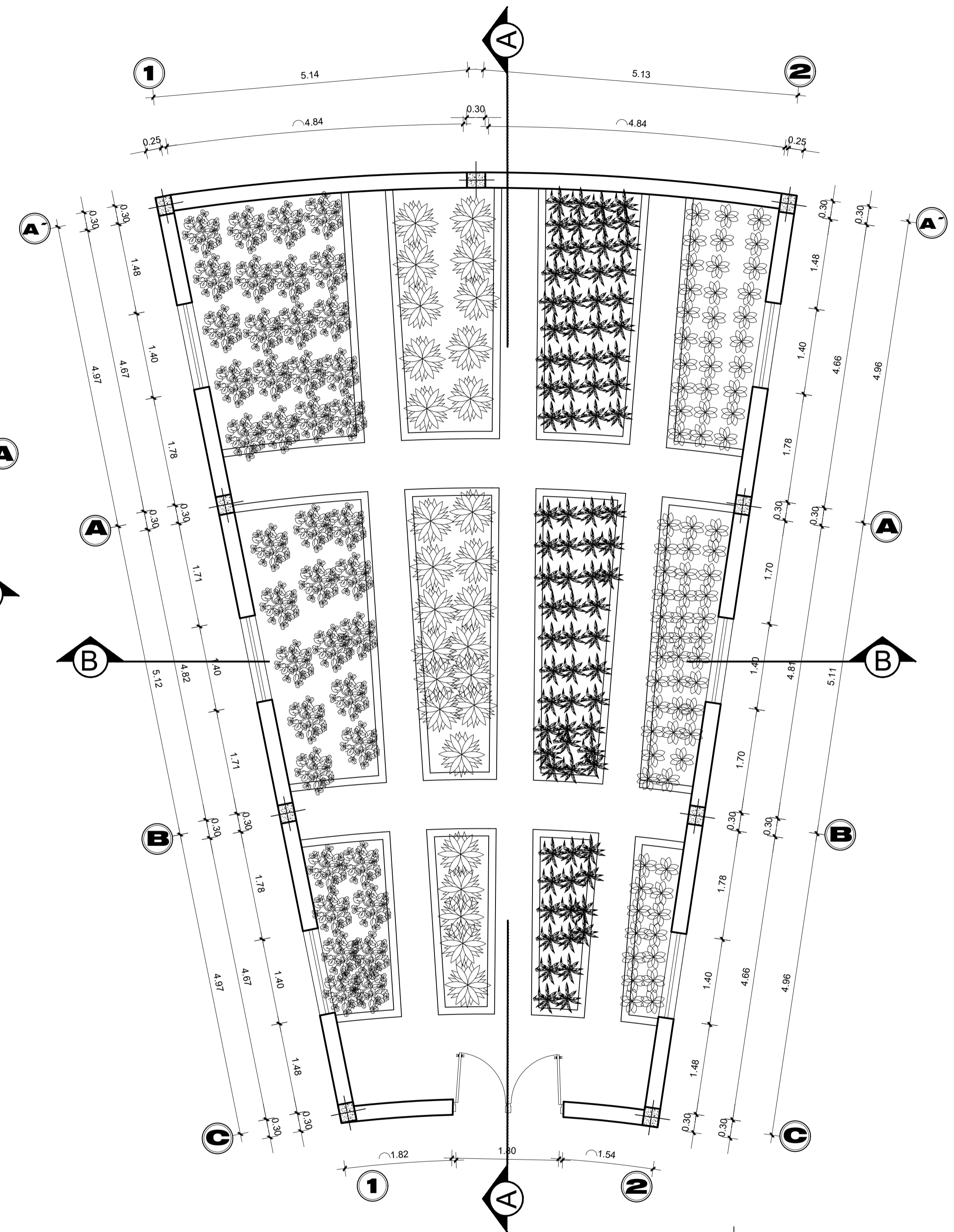
PLANTA-VIVIERO ORNAMENTAL
