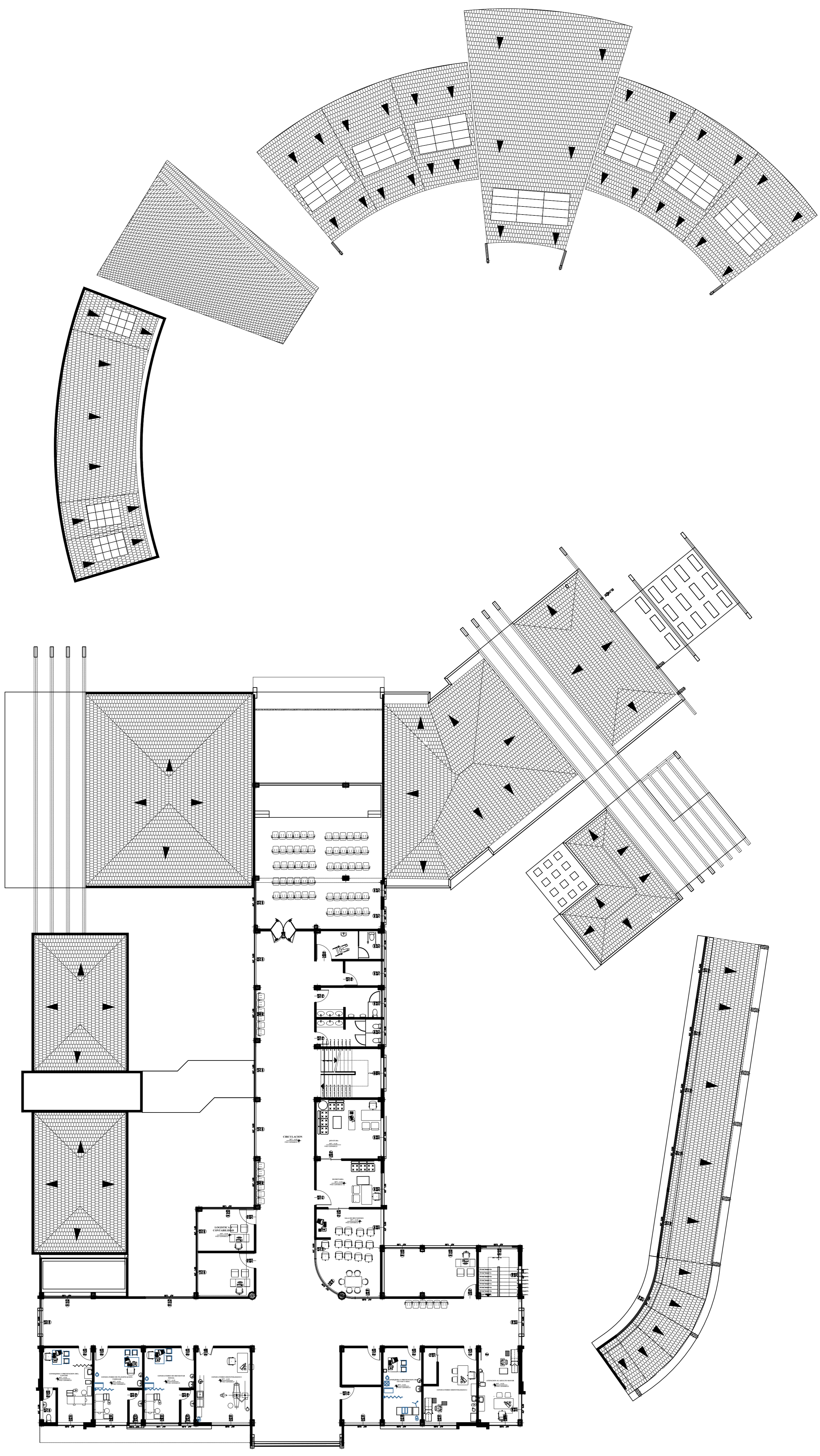
PLANTA GENERAL 2° NIVEL Escala 1:50
