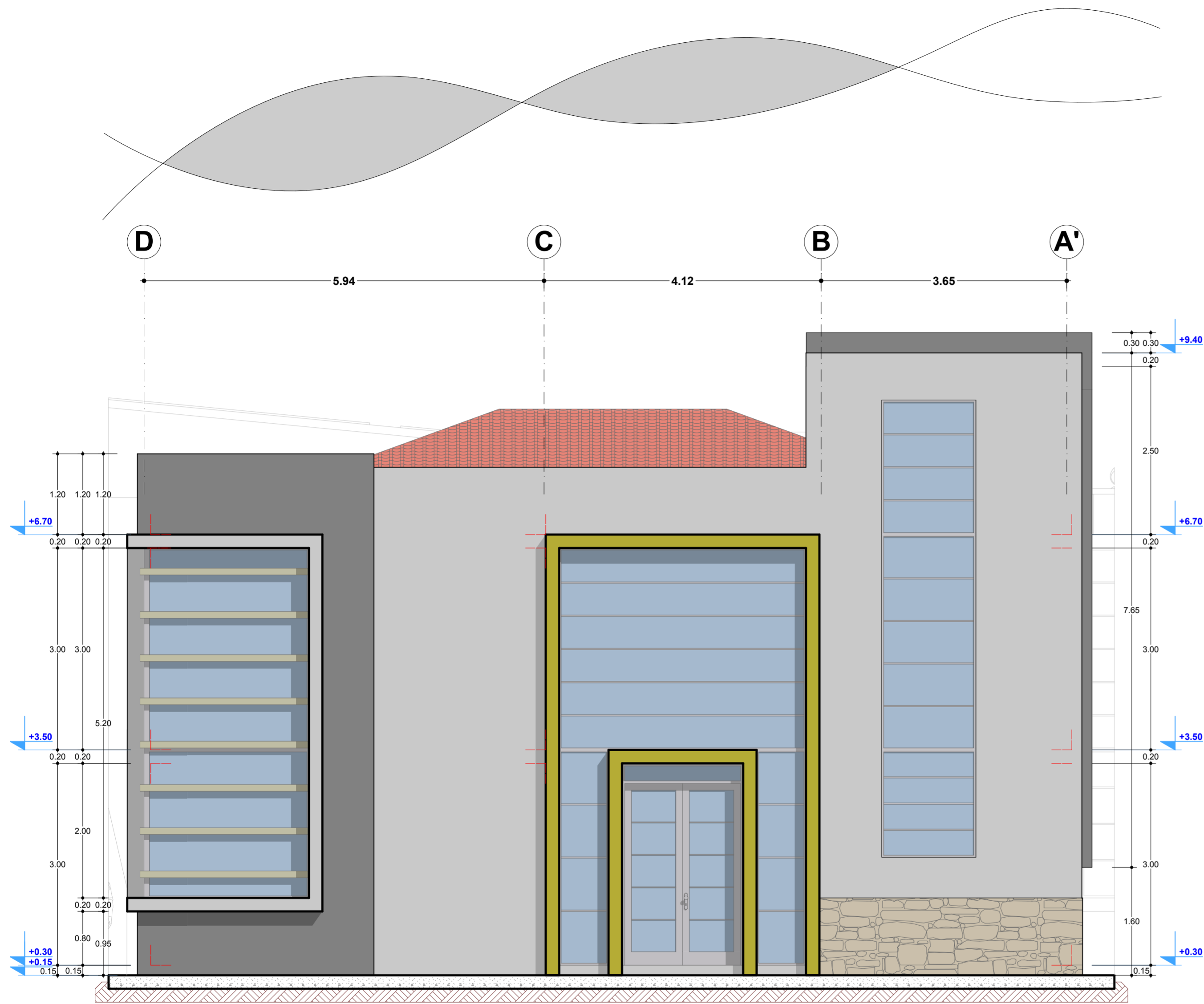
ELEVACION 02
