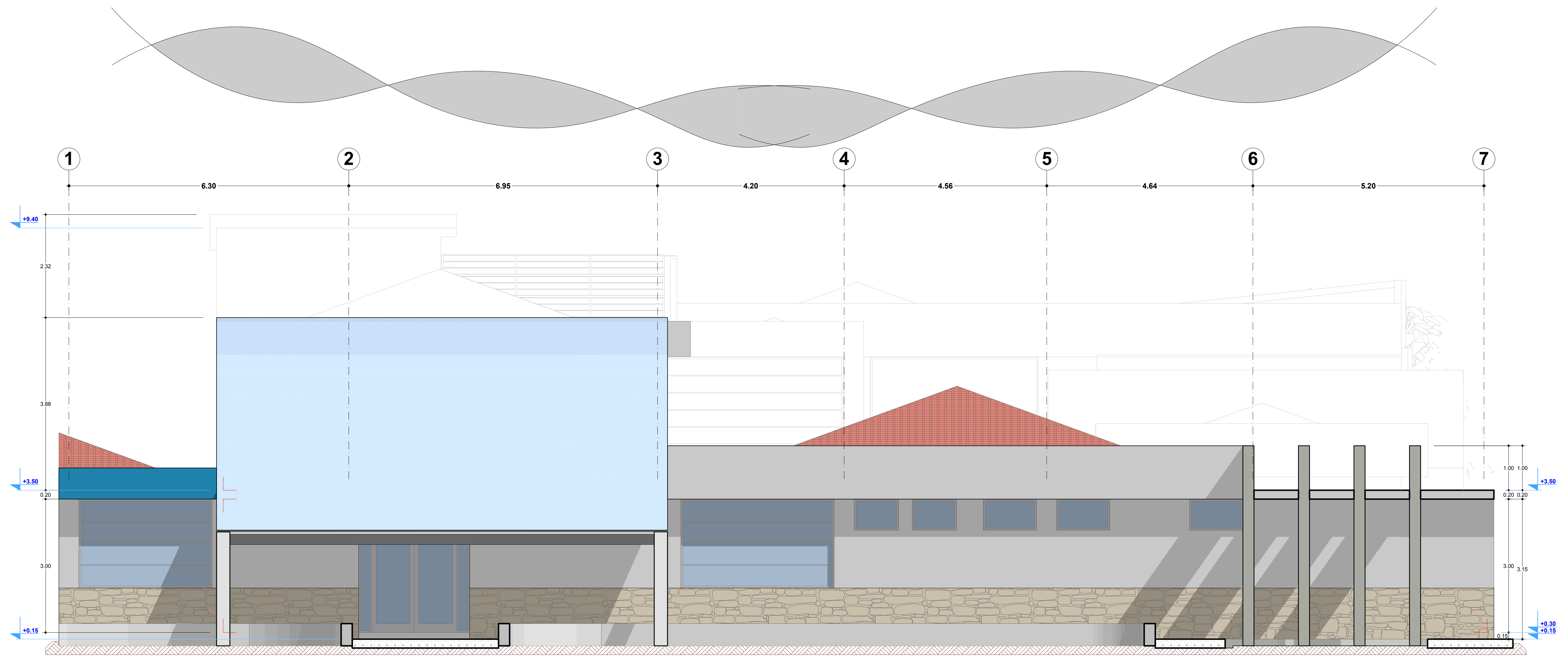
ELEVACION 04
