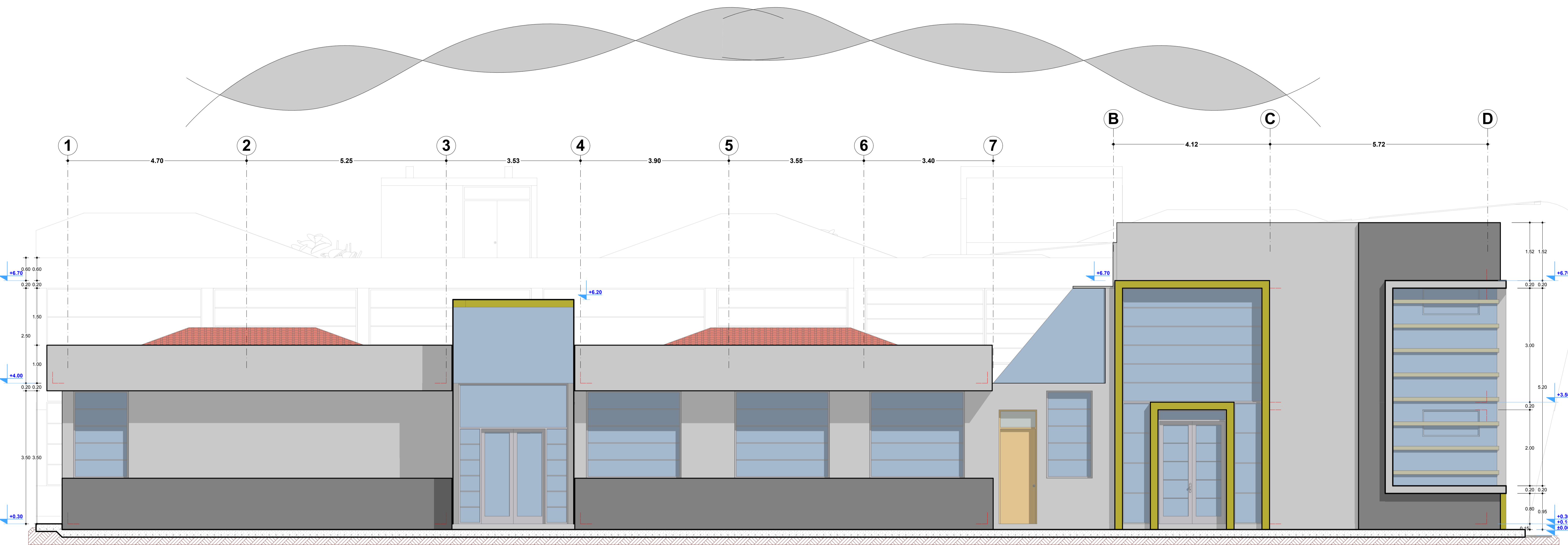
ELEVACION 05
