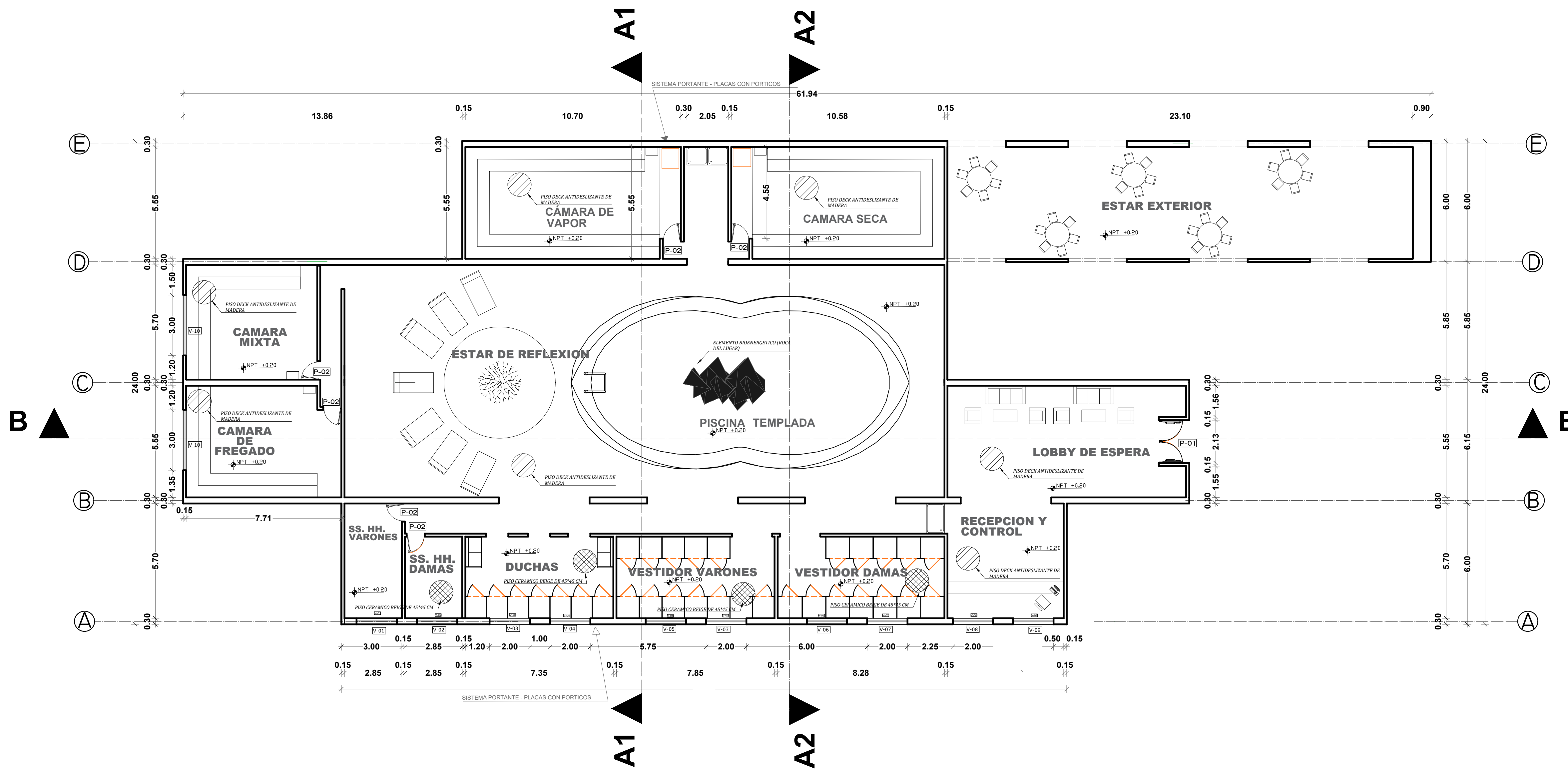
PISCINA Y SAUNA DE MEDITACIÓN. DISTRIBUCIÓN
