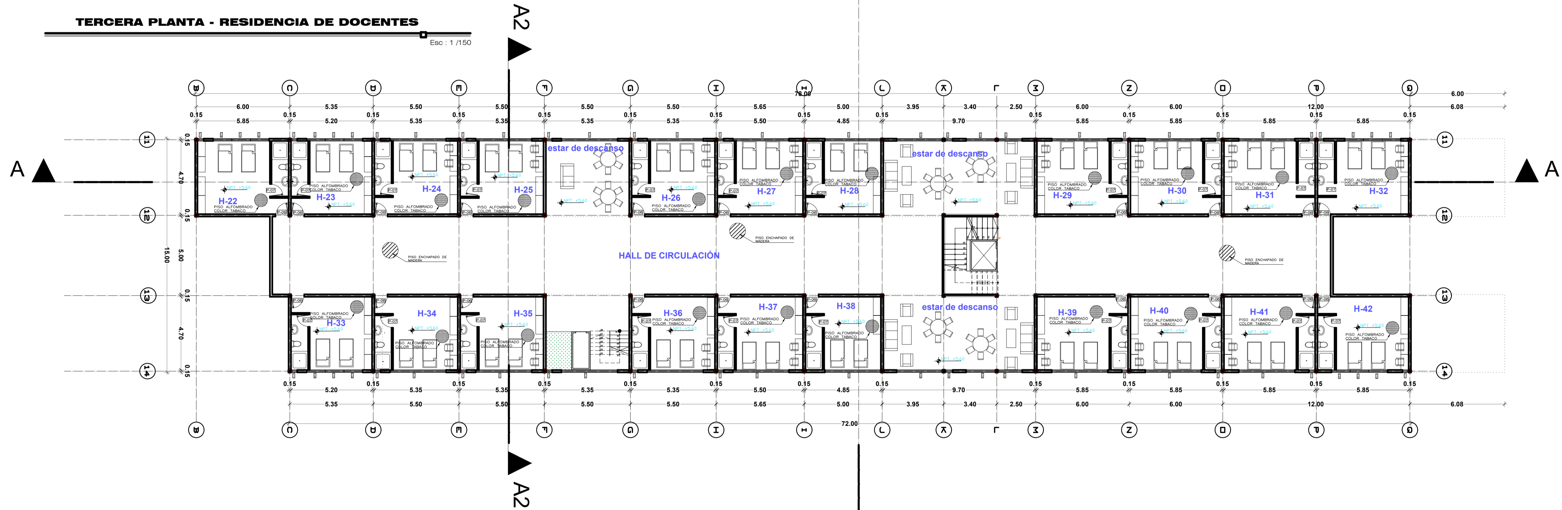
TERCERA PLANTA - RESIDENCIA DE ALUMNOS Y DOCENTES
