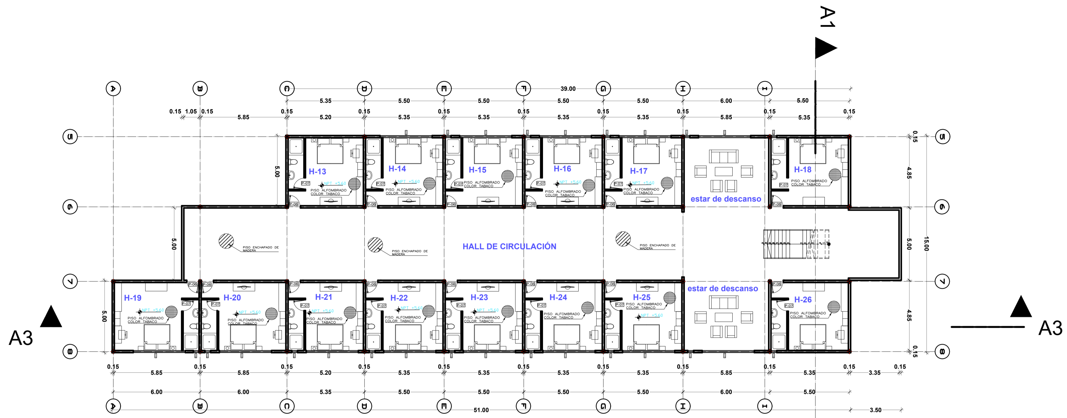
TERCERA PLANTA - RESIDENCIA DE DOCENTES
