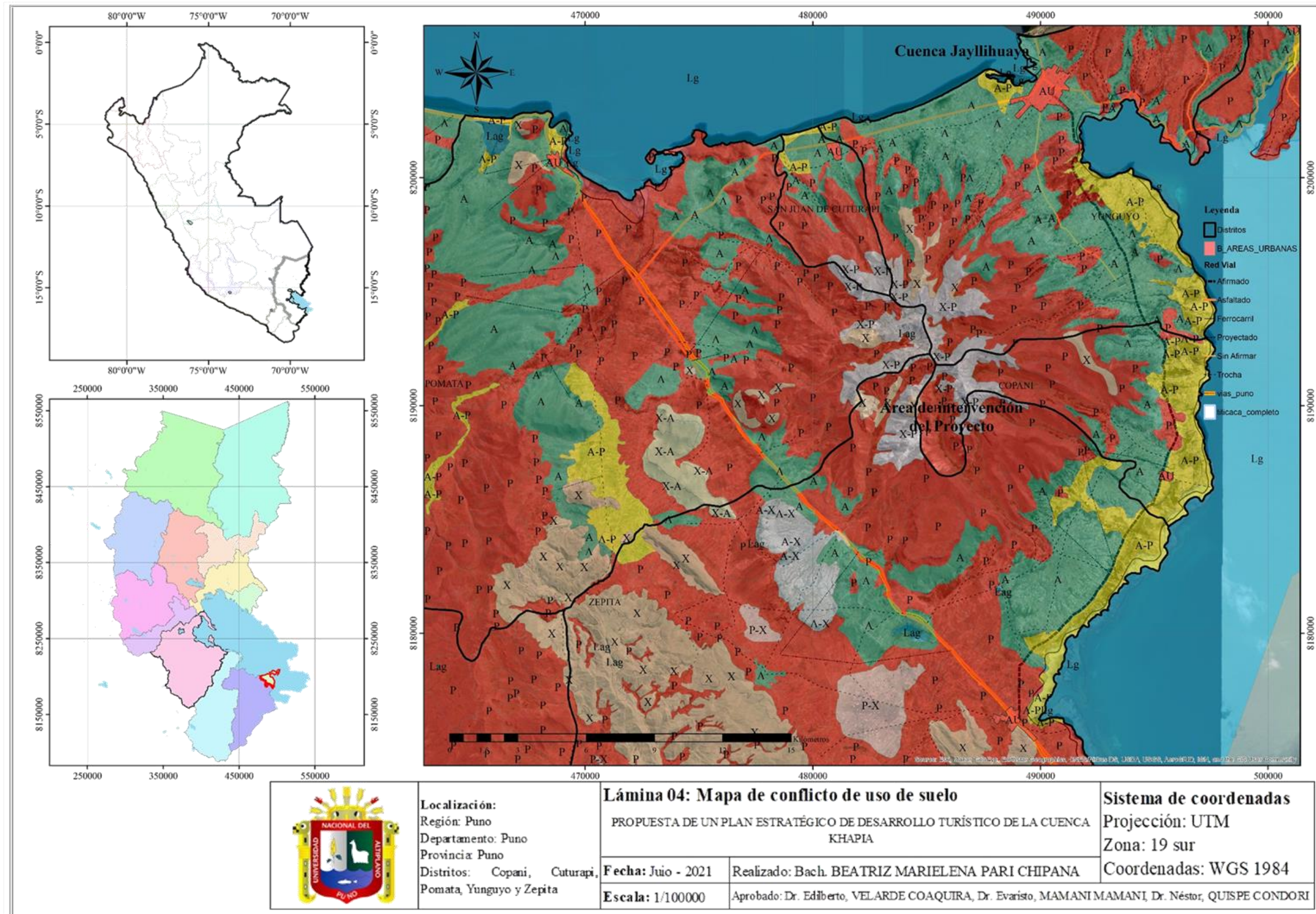
Figura 45. Mapa de conflicto de uso de suelo
