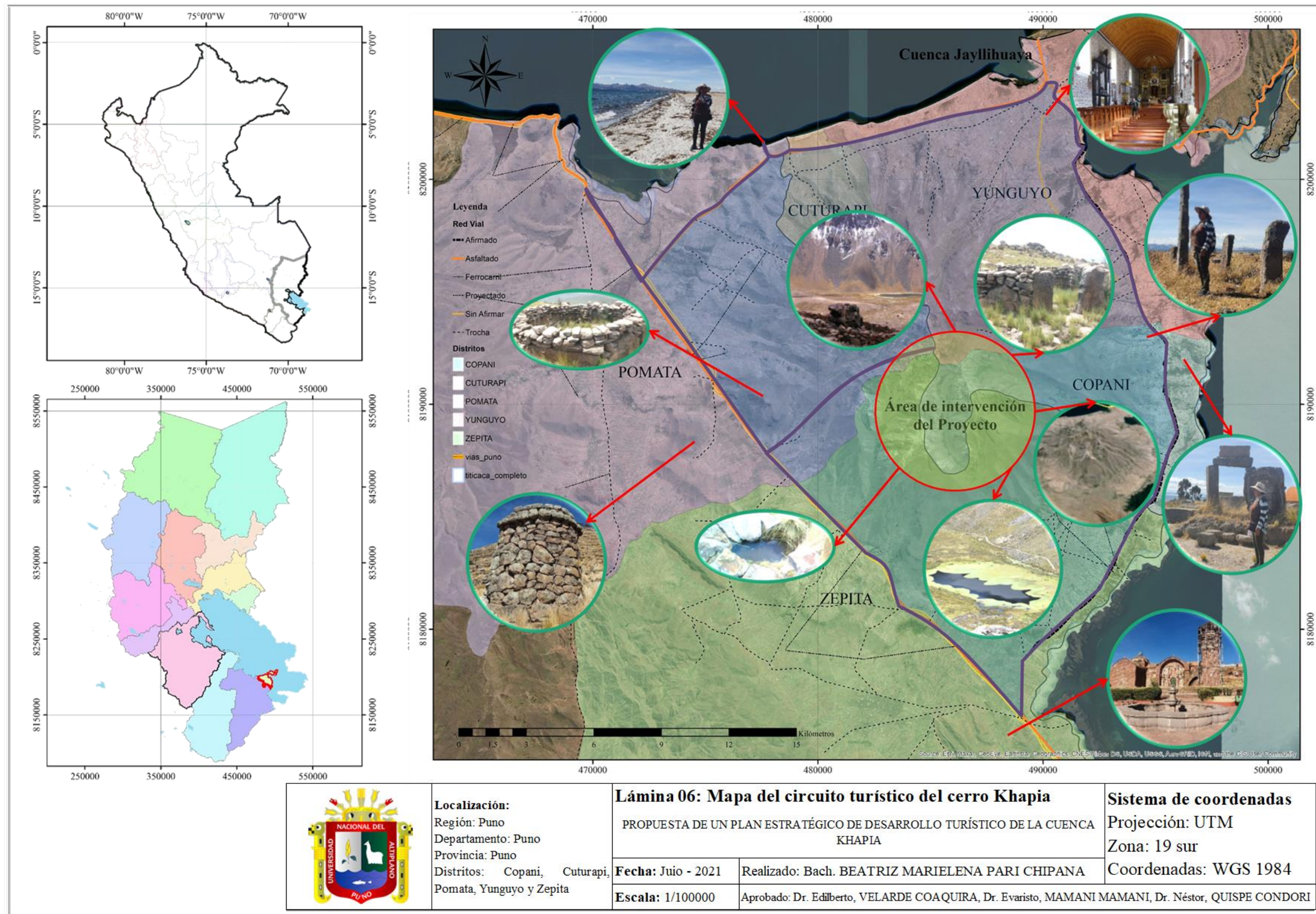
Figura 47. Mapa del circuito turístico del cerro Khapia
