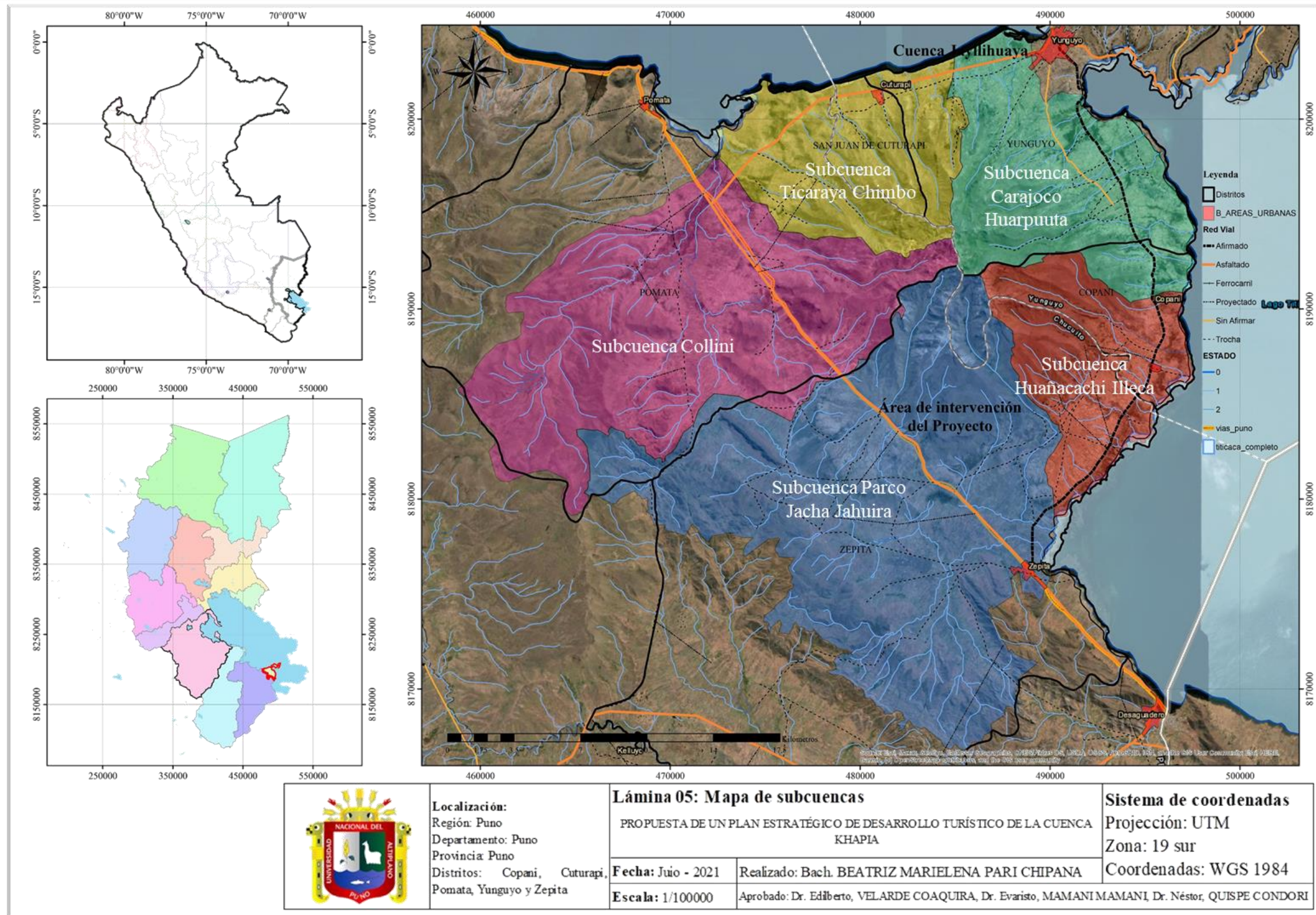
Figura 46. Mapa de las subcuencas
