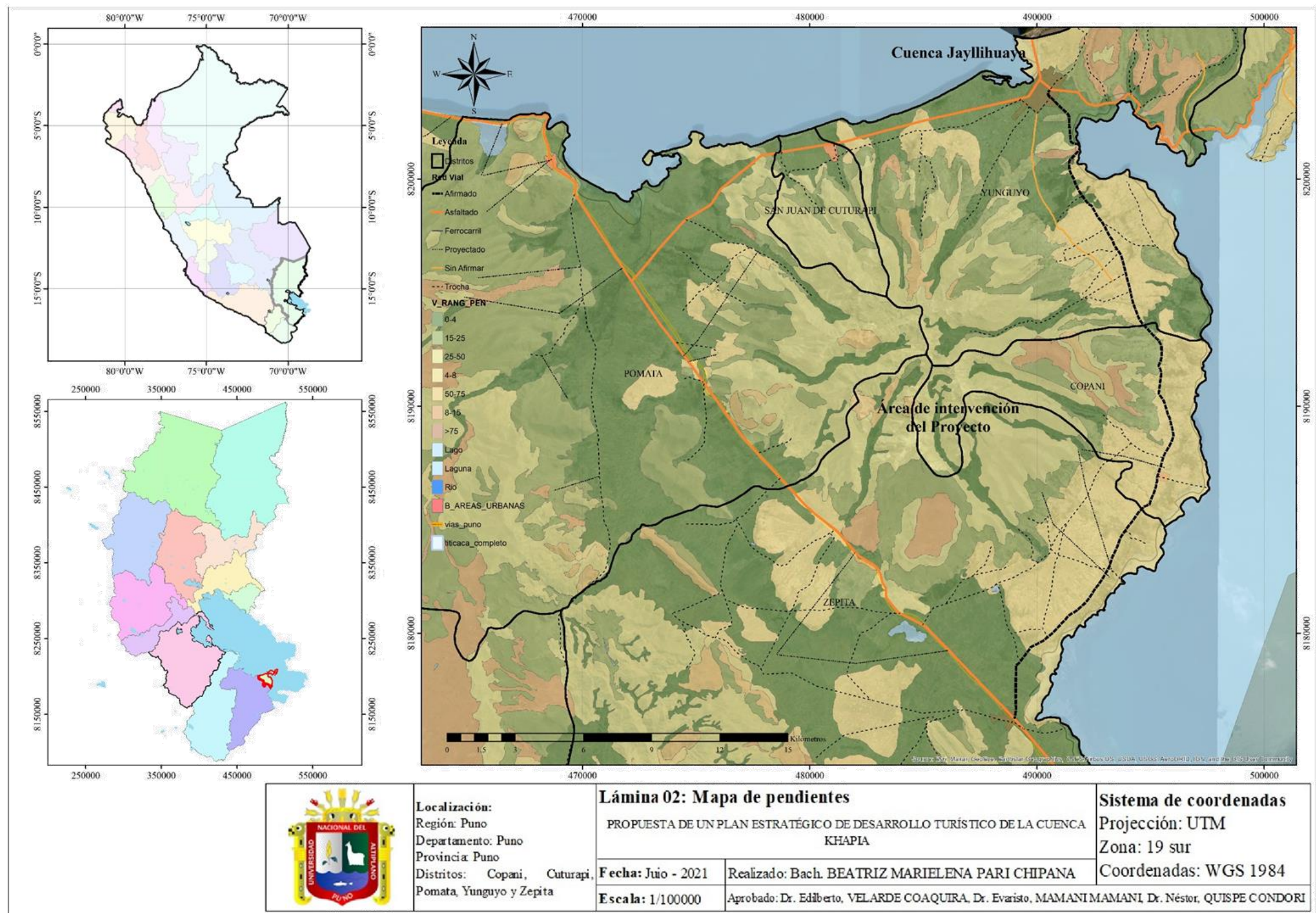
Figura 43. Mapa de pendientes
