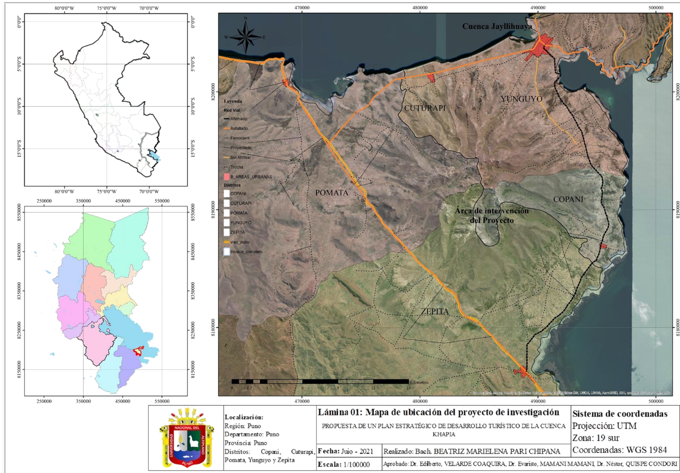
Figura 42. Mapa de ubicación de la zona de estudio
