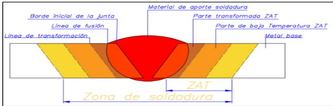
Figura 1. Componentes que se forma y representación de temperaturas en el proceso de soldadura.
