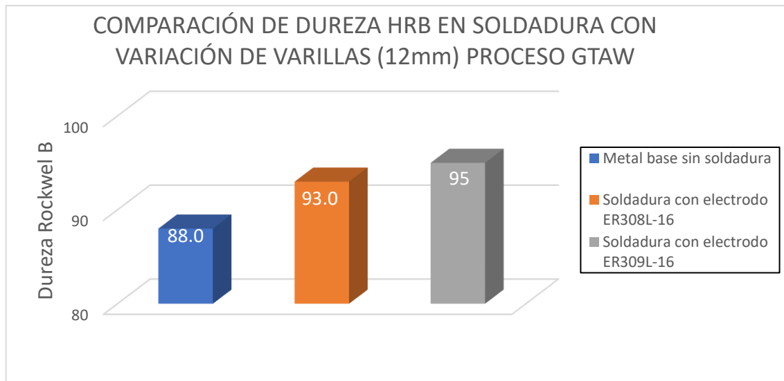
Figura 23. Comparación de dureza (HRB) en soldadura con varilla de 12 mm, proceso GTAW
