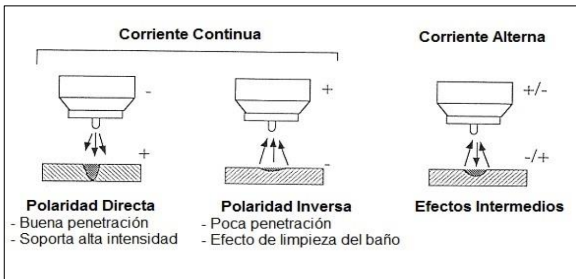
Figura 6. Tipos de corriente en el proceso de soldadura GTAW
