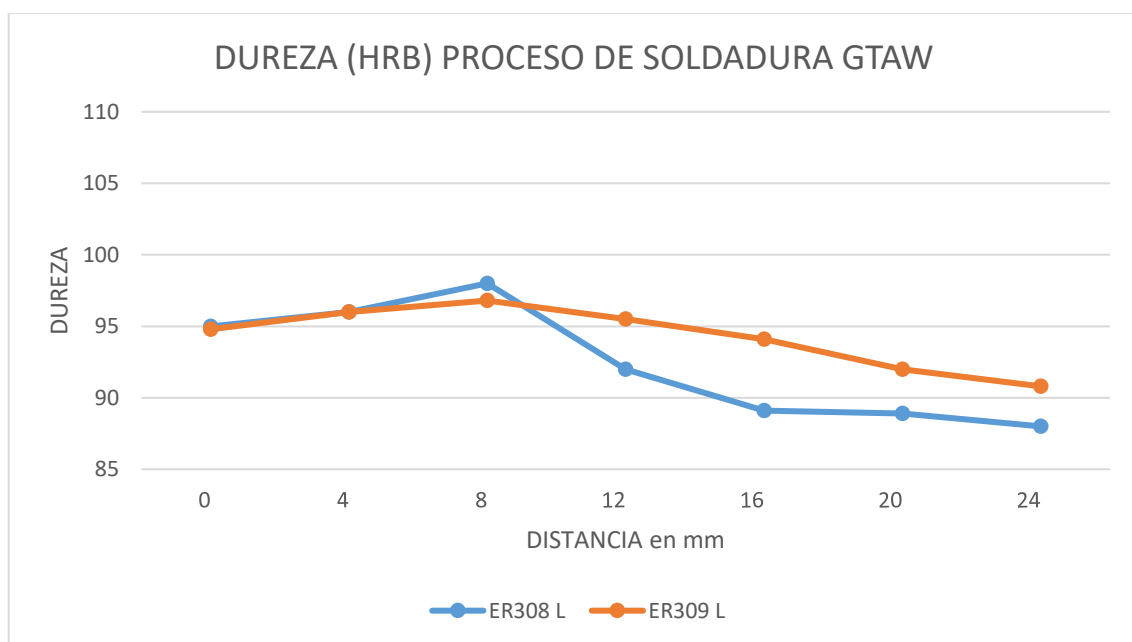
Figura 24. Relación de durezas en juntas soldadas GTAW
