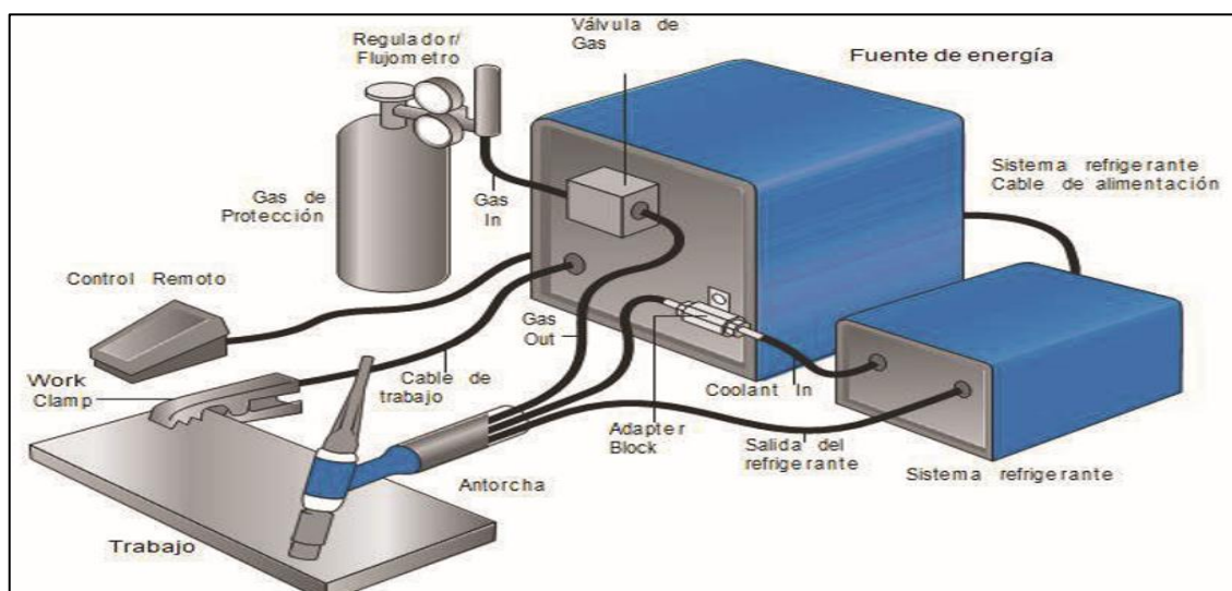
Figura 4. Elementos esenciales de proceso GTAW
