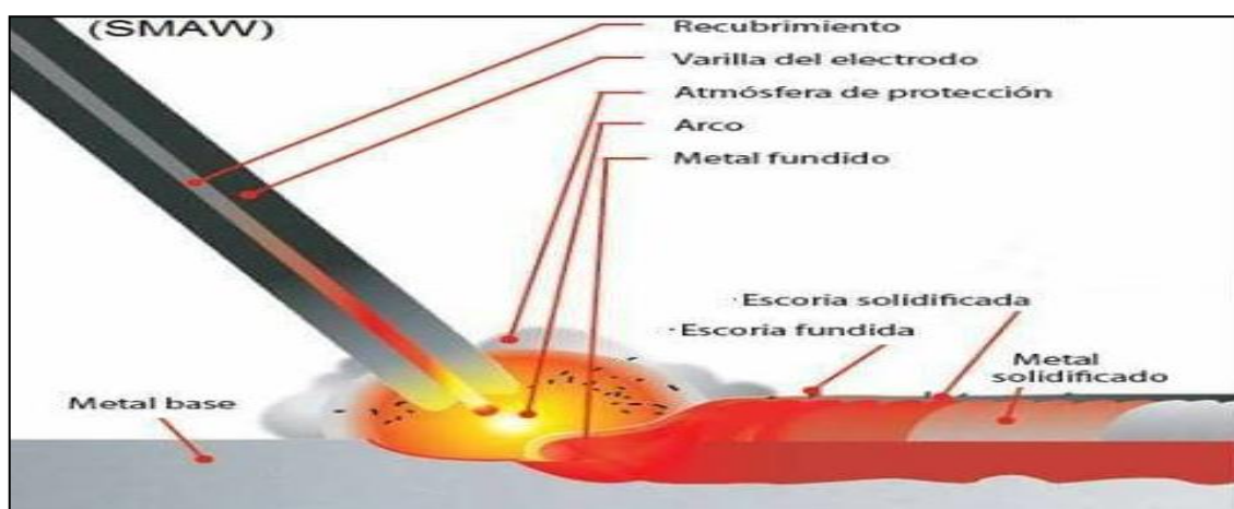
Figura 3. Proceso de la soldadura SMAW
