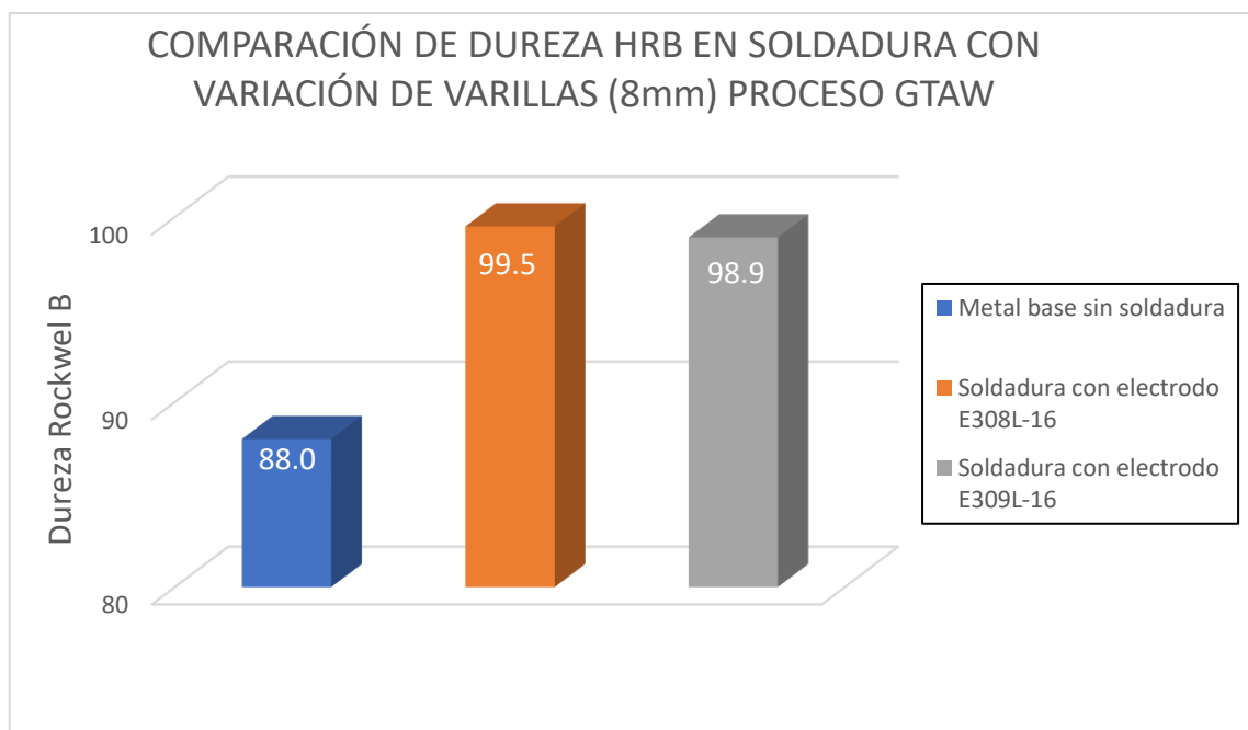
Figura 22. Comparación de dureza (HRB) en soldadura con varilla de 8 mm, proceso GTAW
