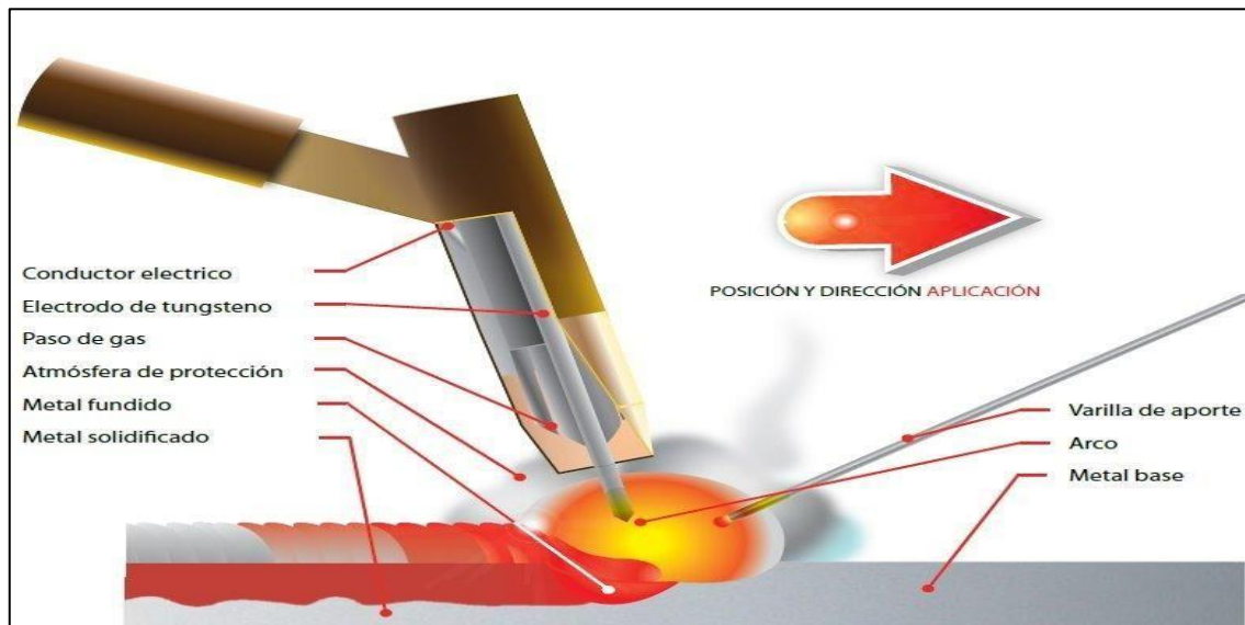
Figura 5. Proceso de la soldadura GTAW
