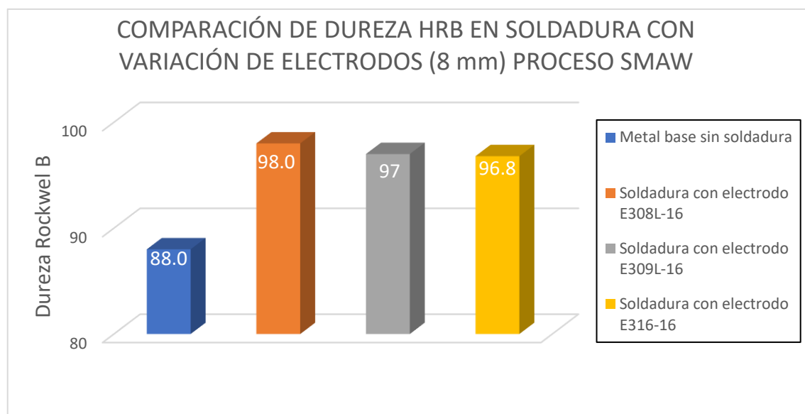
Figura 18. Comparación de Dureza (HRB) con variación de electrodos de 8 mm
