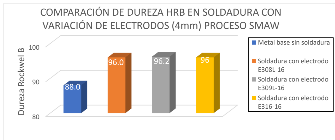
Figura 17. Comparación de Dureza Rockwell (HRB) con variación de 4 mm
