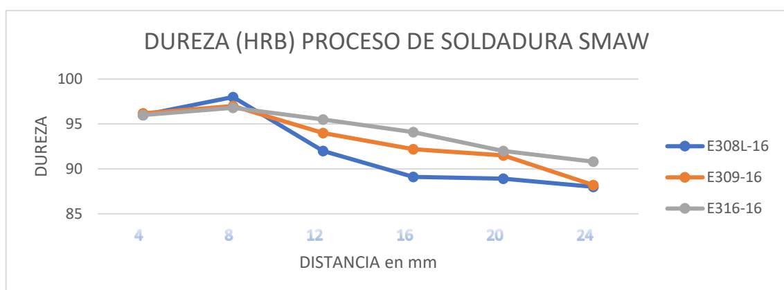
Figura 20. Relación de durezas en juntas soldadas SMAW
