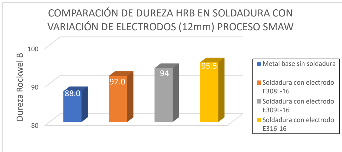
Figura 19. Comparación de Dureza Rockwell (HRB) con variación de 12 mm
