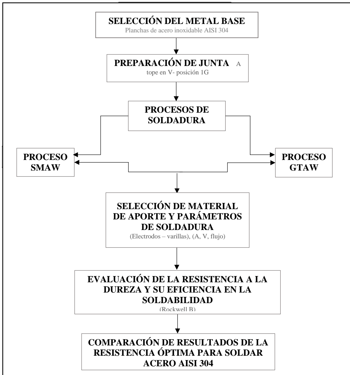
Figura 9. Flujograma del procedimiento experimental
