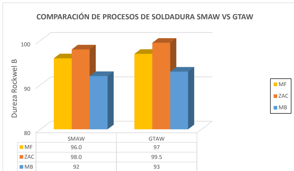
Figura 25. Comparación de Procesos de Soldadura SMAW vs. GTAW
