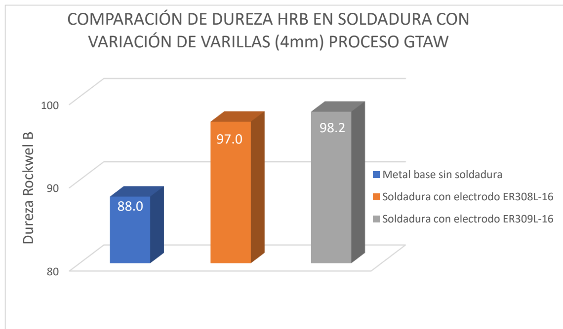
Figura 21. Comparación de dureza (HRB) en soldadura con varilla de 4mm, proceso GTAW
