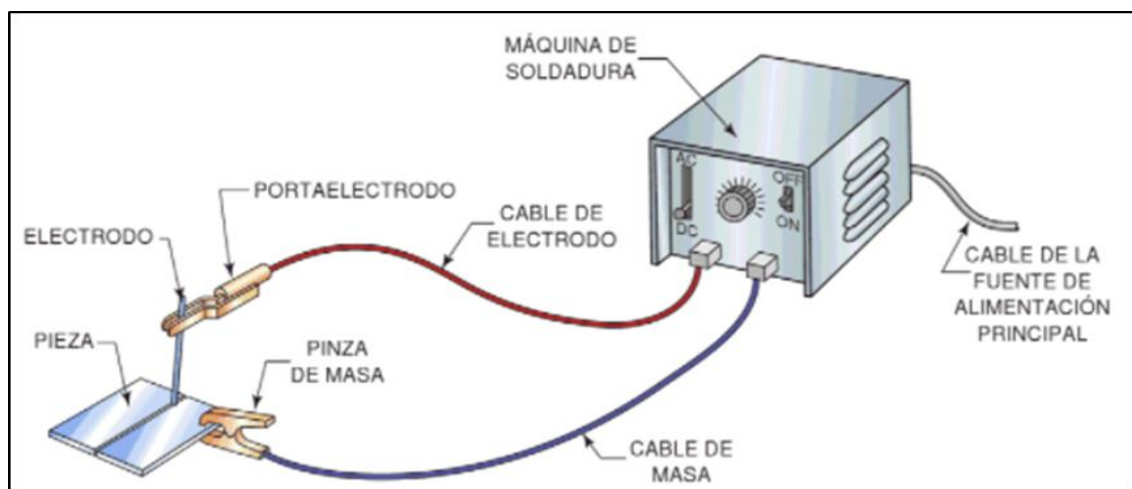
Figura 2. Equipo Proceso de soldadura SMAW
