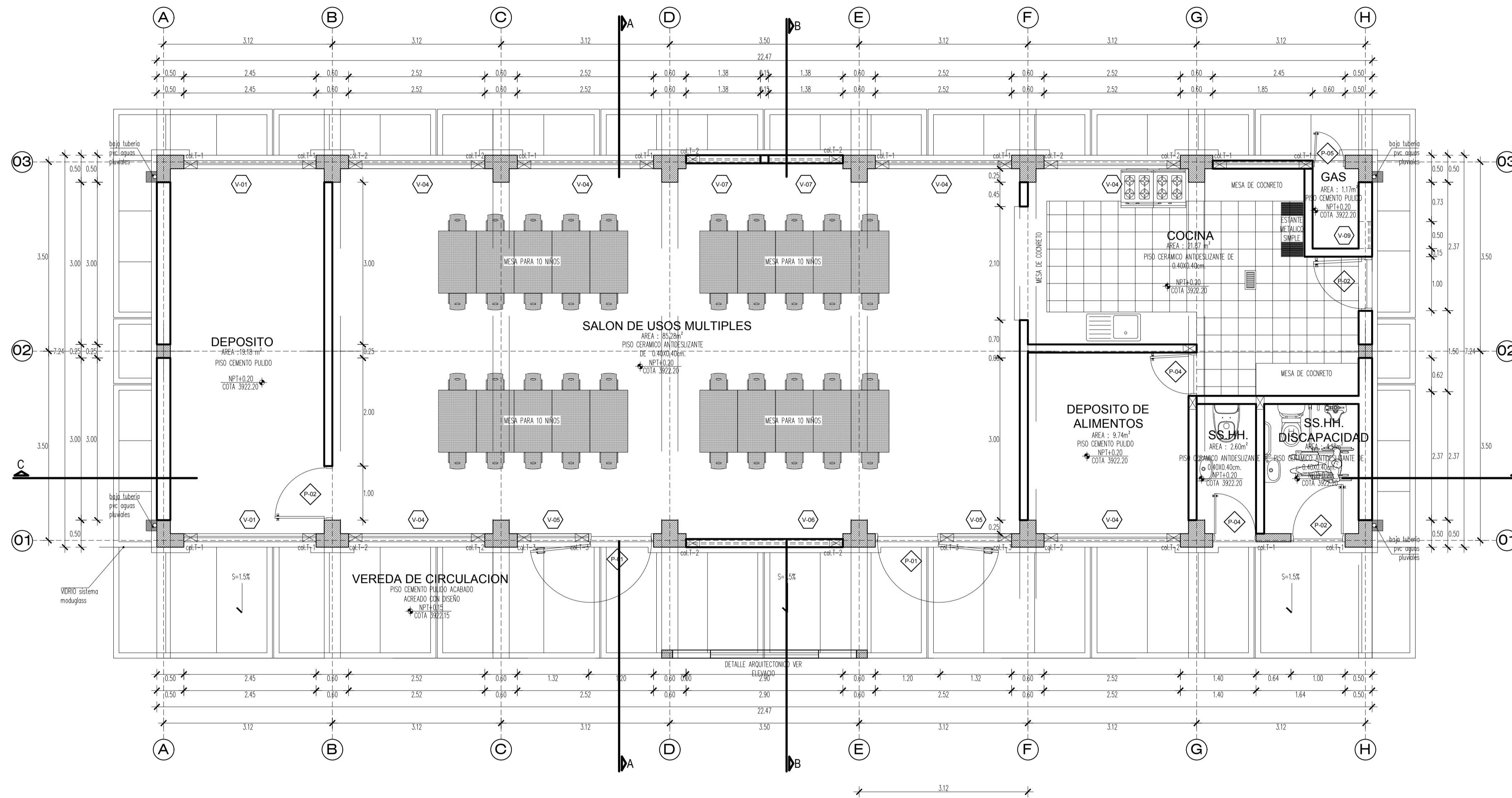
PLANO DISTRIBUCION 1ER NIVEL MODULO 04 Esc 1:50
