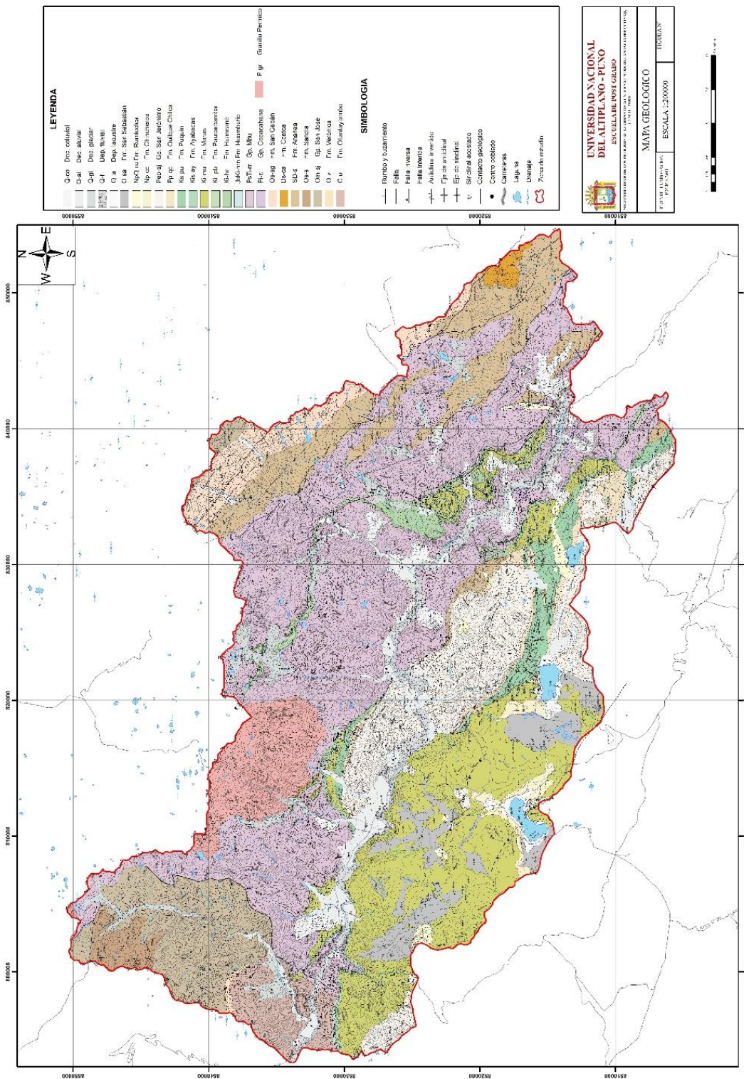
Figura 3. Mapa geológico
