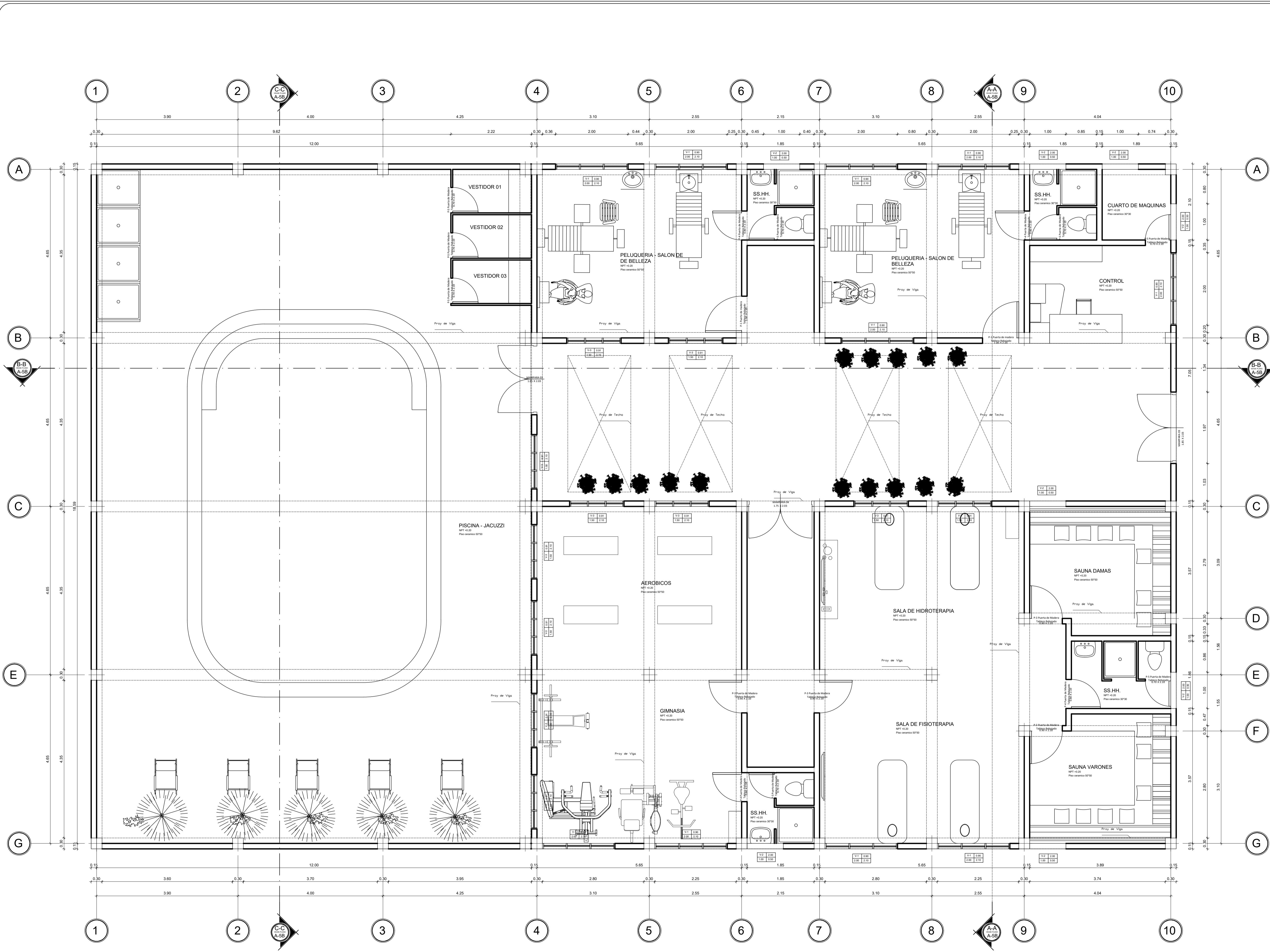
DISTRIBUCION PRIMER NIVEL Esc: 1/50
