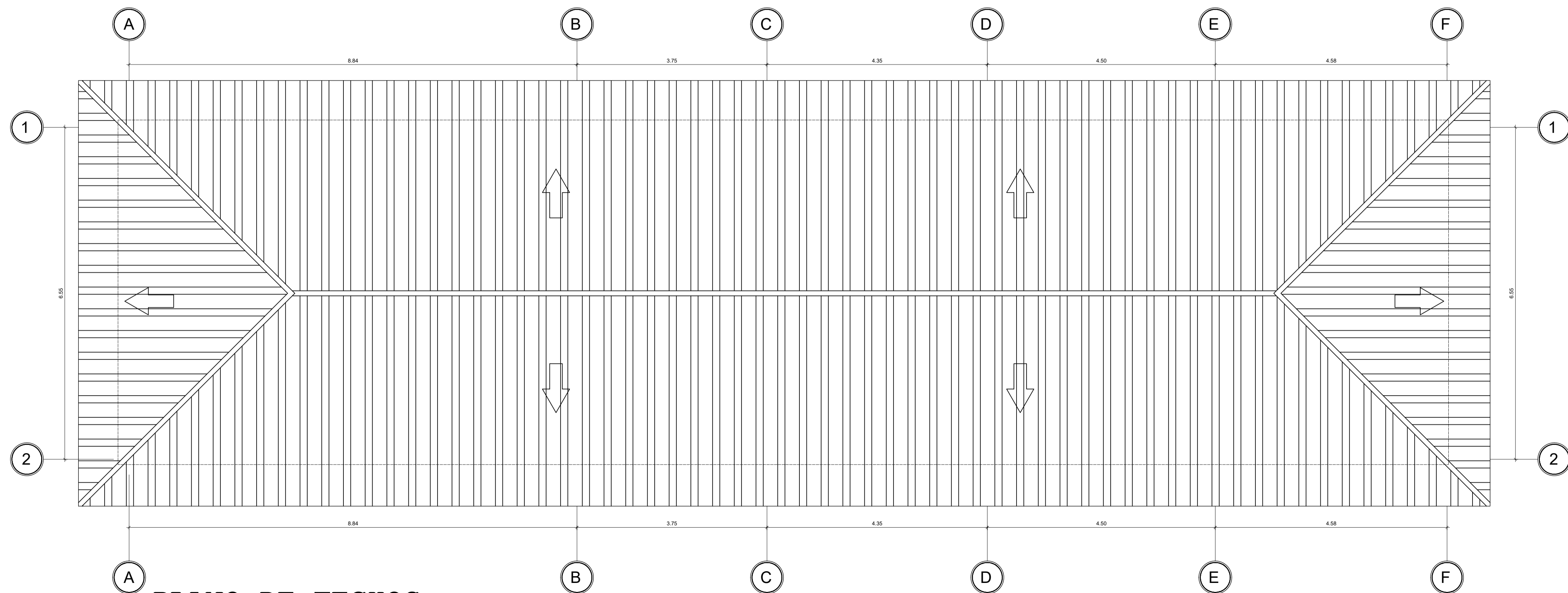
PLANO DE TECHOS PRIMER NIVEL Esc: 1/50
