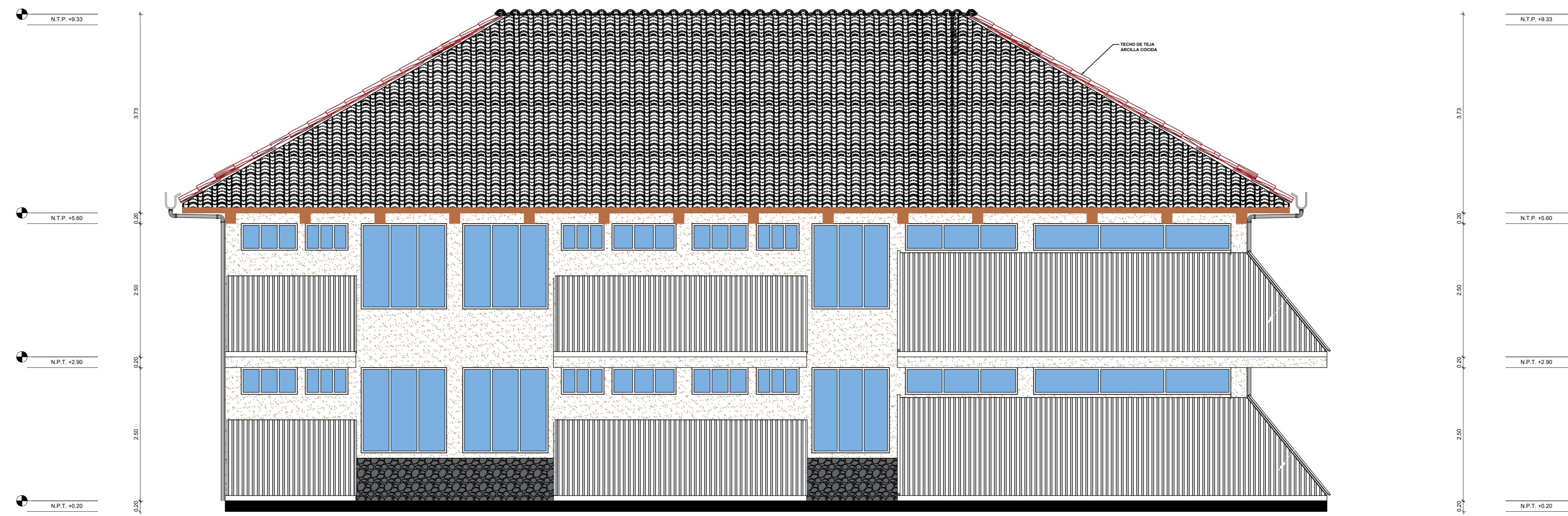
ELEVACIÓN LATERAL Esc: 1/50
