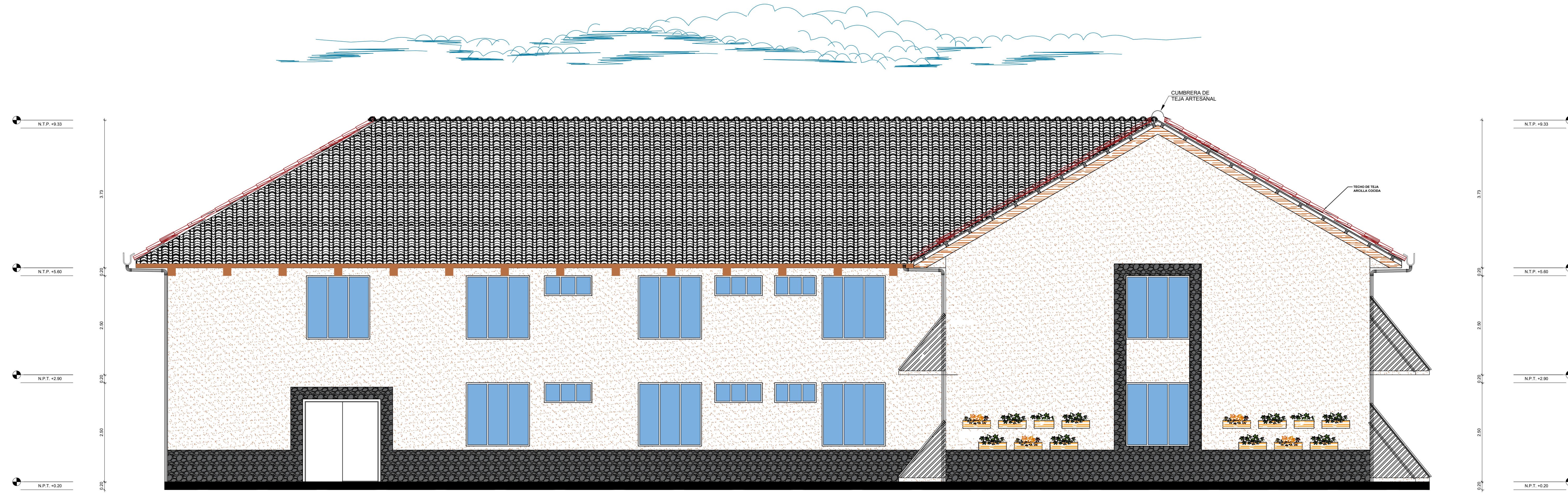
ELEVACIÓN FRONTAL Esc: 1/50
