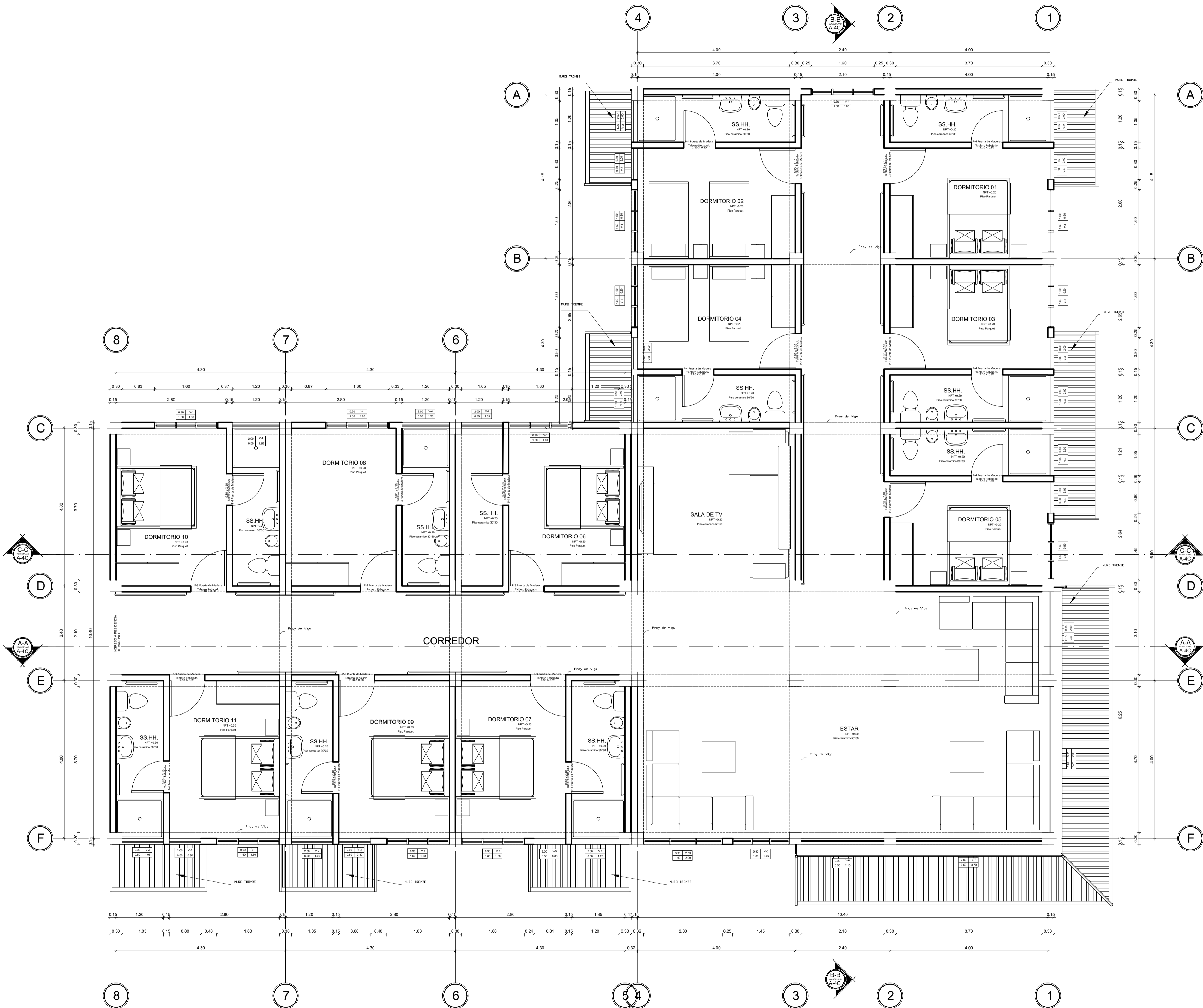
DISTRIBUCION PRIMER NIVEL Esc: 1/50
