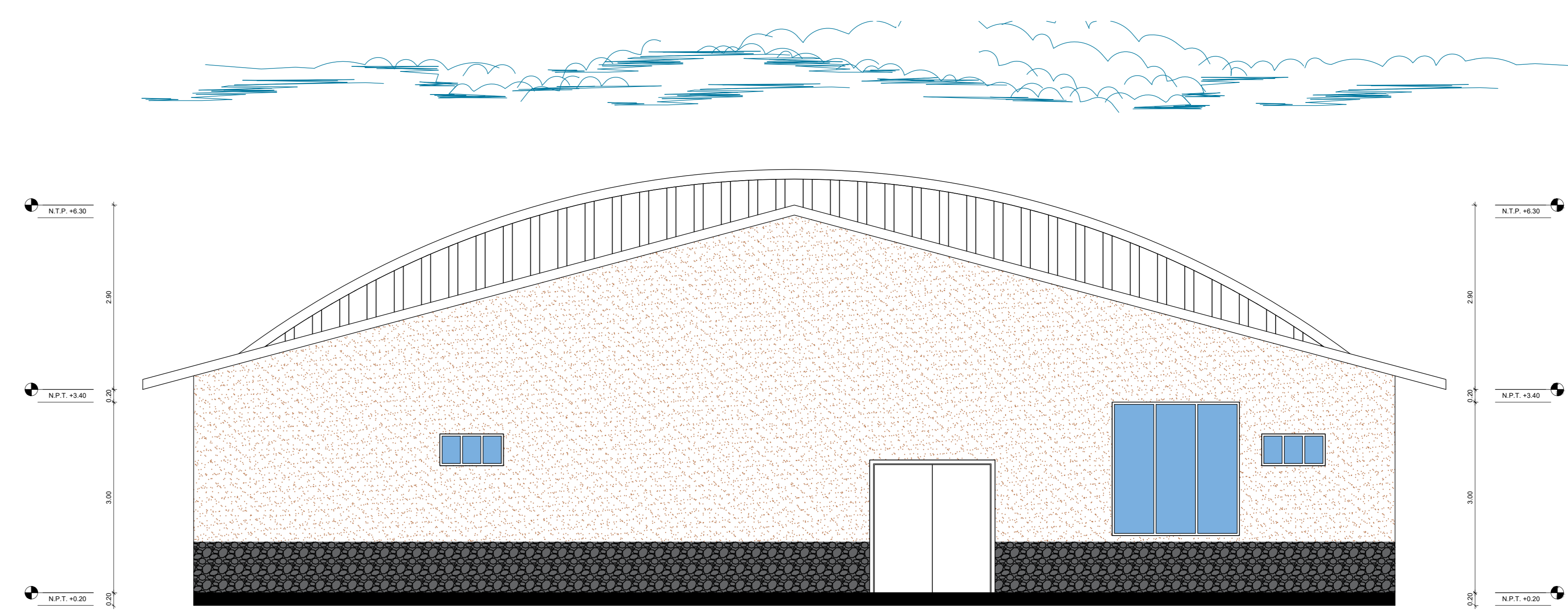
ELEVACIÓN FRONTAL Escala: 1/50
