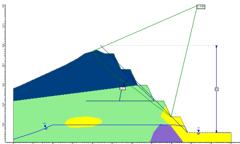
SECCIÓN 10
