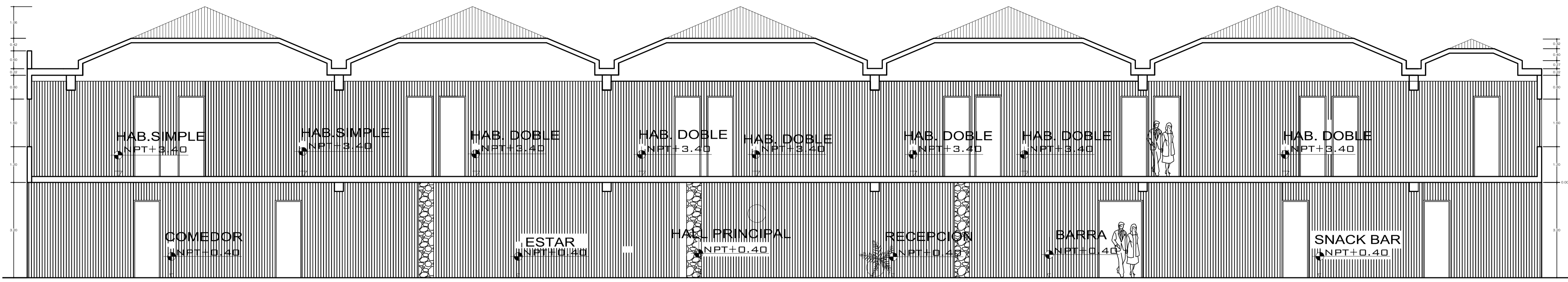
SECCION A-A PRIMER - SEGUNDO NIVEL HOSPEDAJE ESC: 1/75
