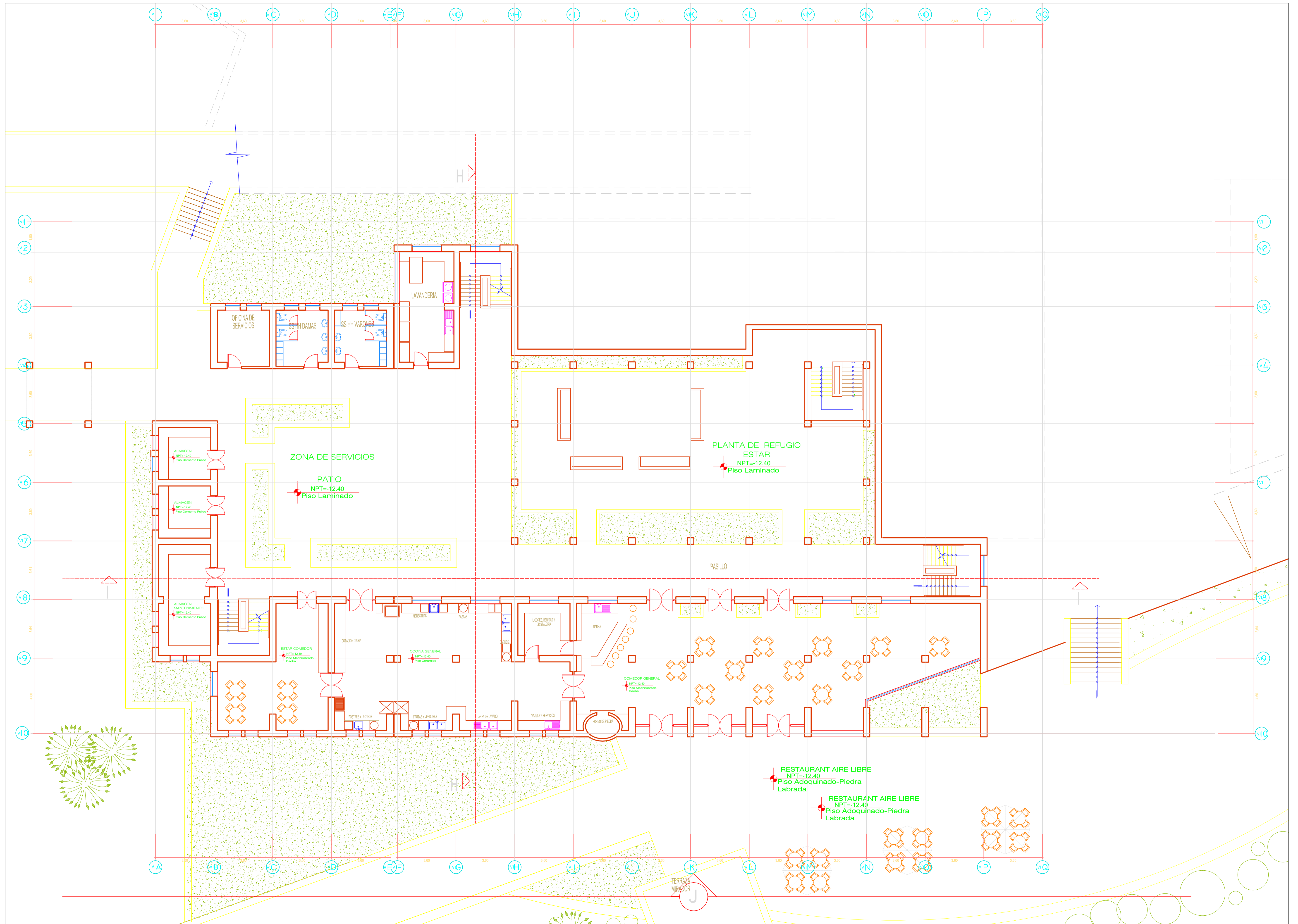
PLANTA MODULO DE HOTEL (Nivel -12.40)
