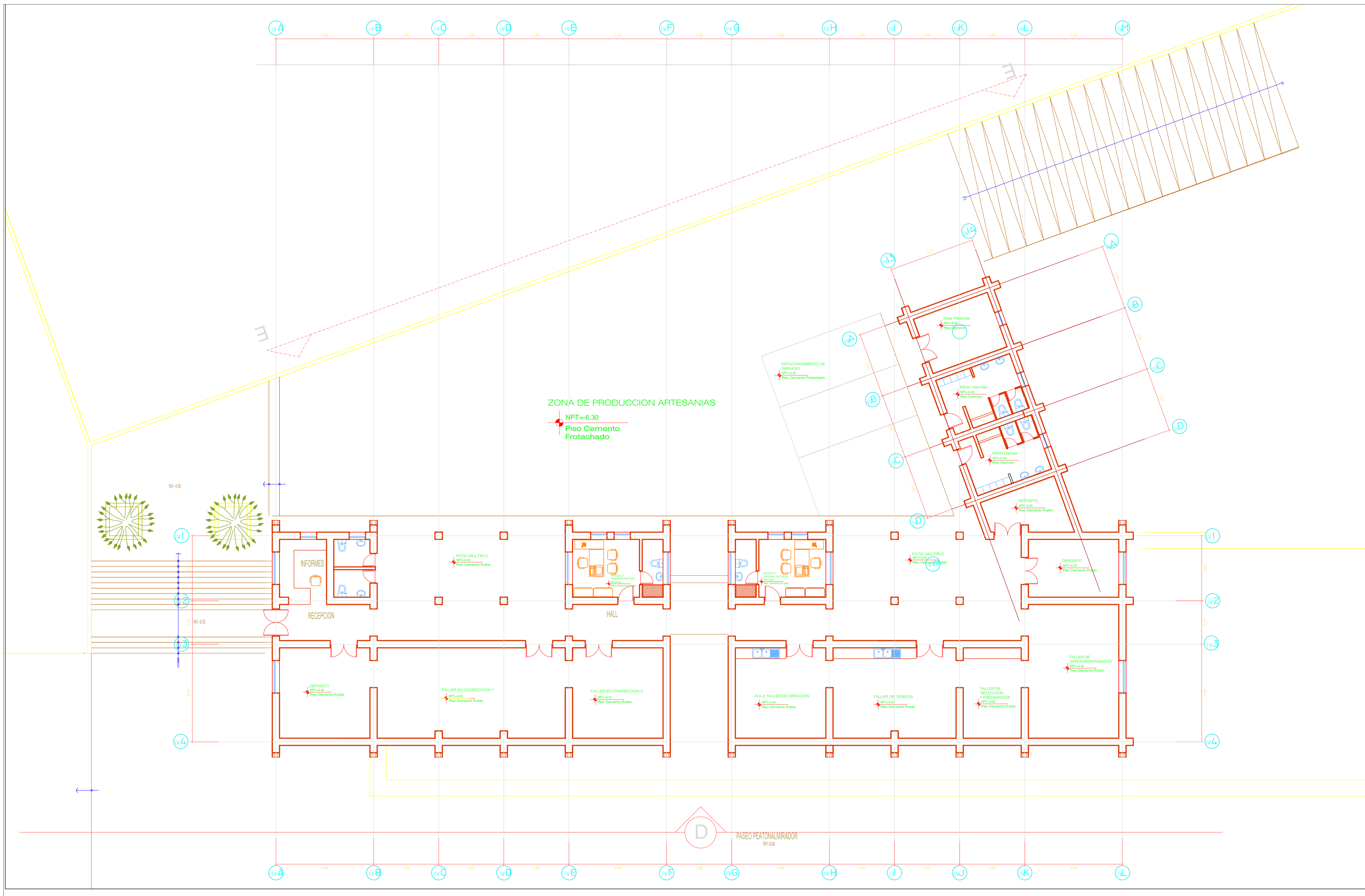
PLANTA MODULO DE CABALLERIZAS (Nivel -12.00)
