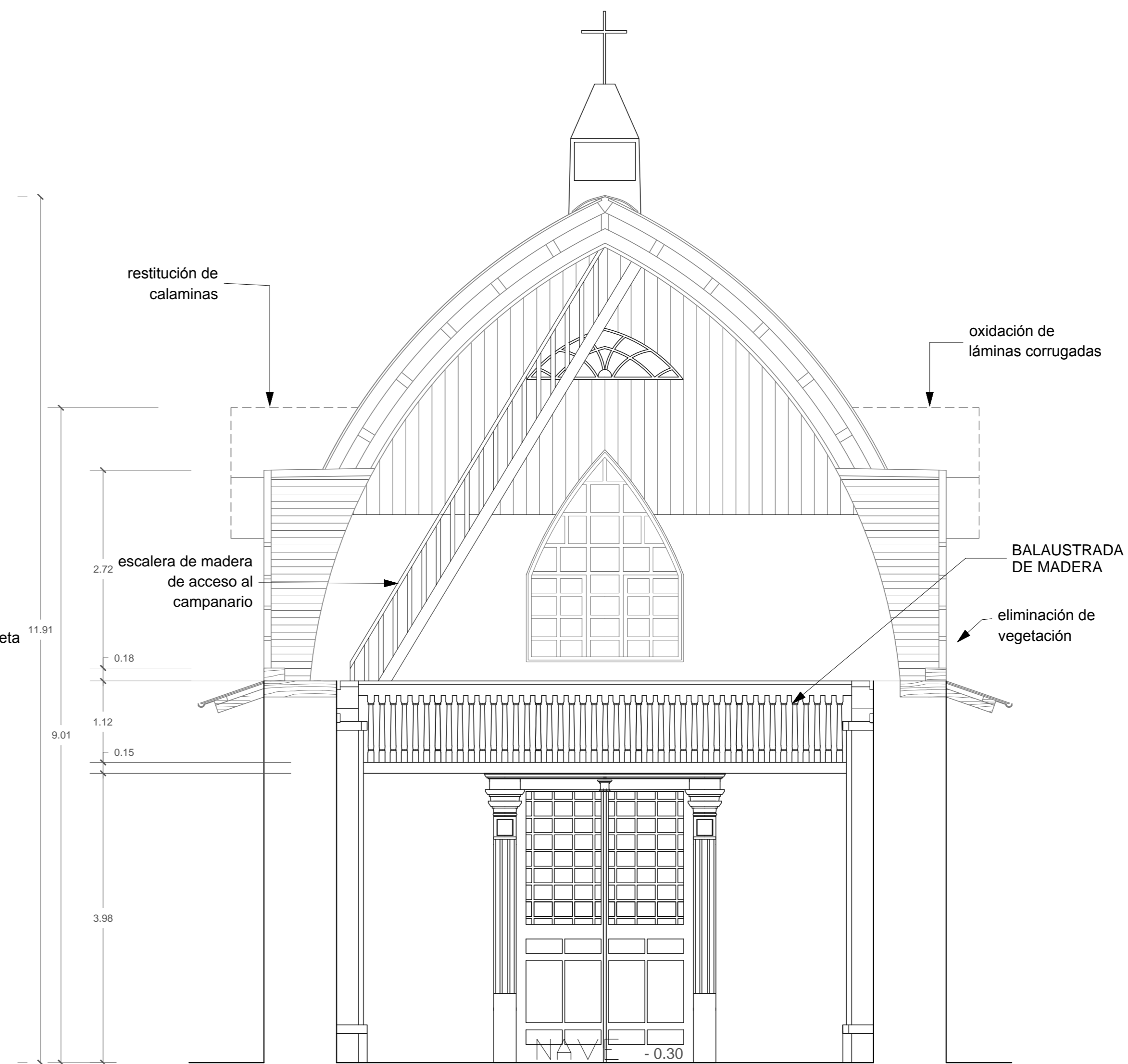
CORTE D - D PROPUESTA DE RESTAURACION ESC 1/50
