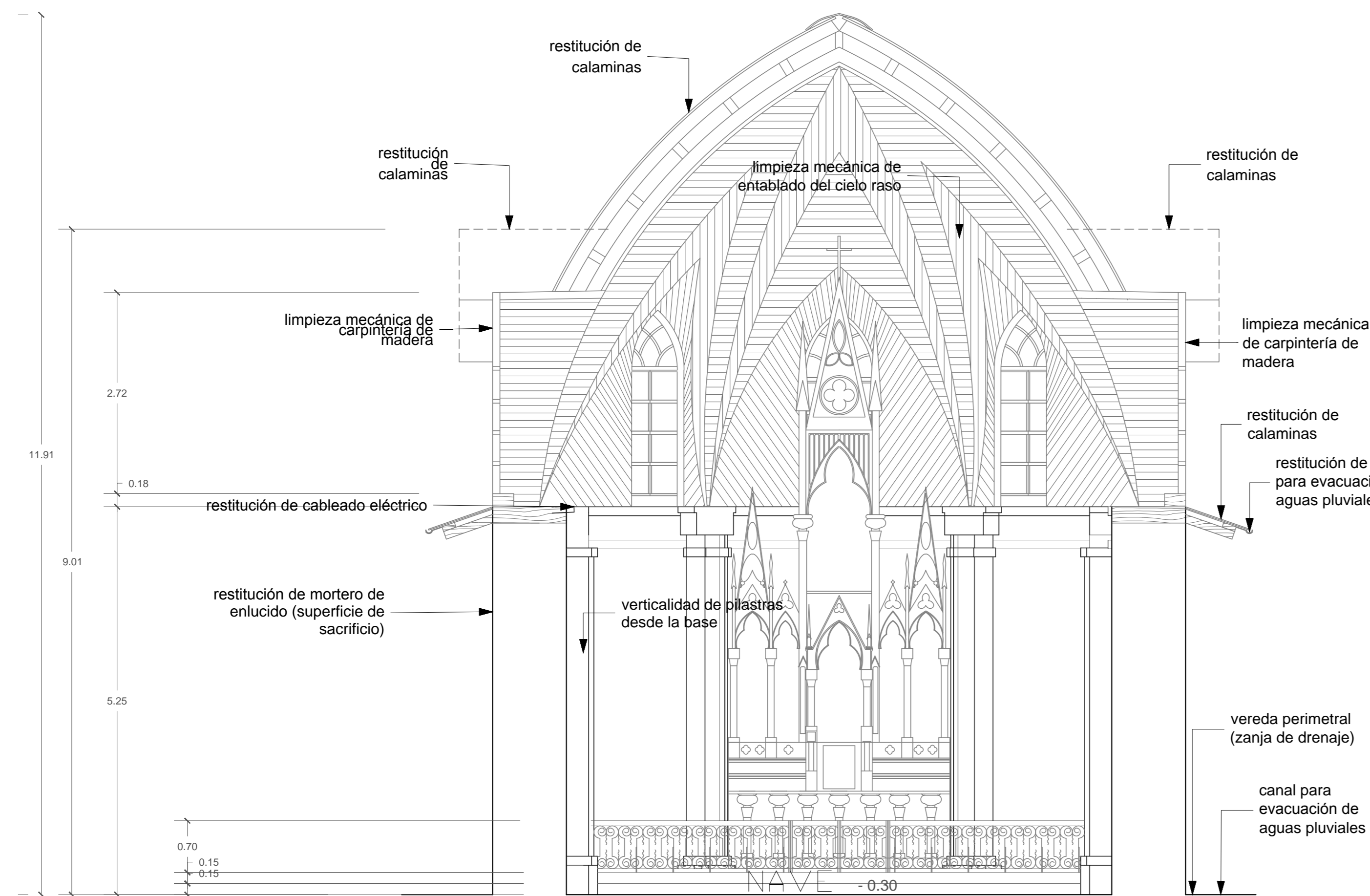
CORTE C - C PROPUESTA DE RESTAURACION ESC 1/50
