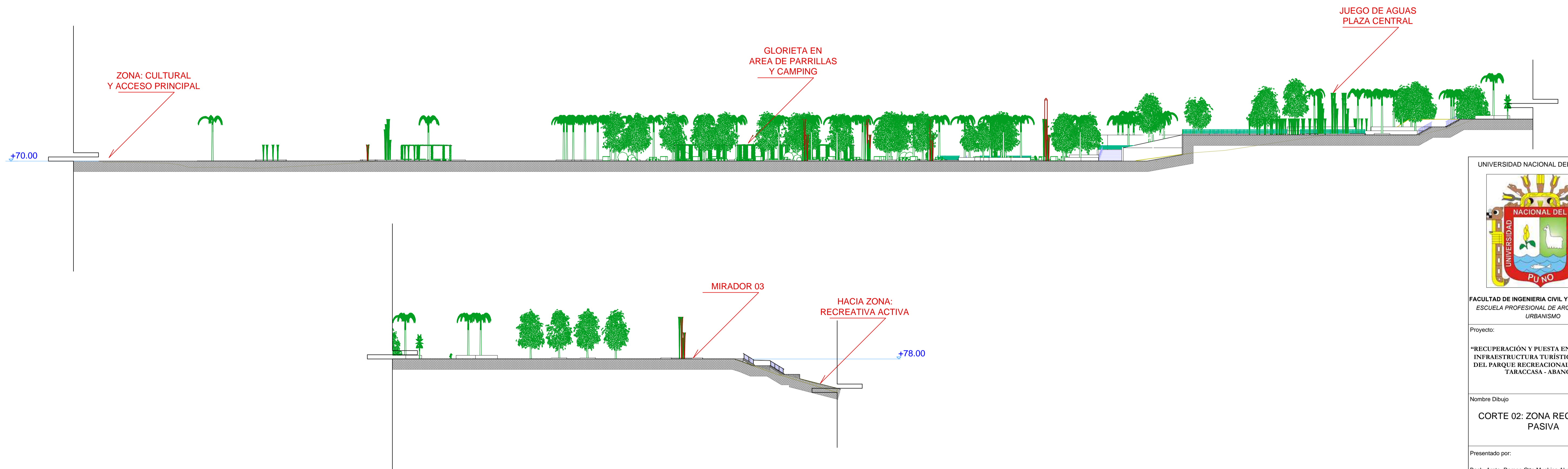
CORTE 02 - ZONA RECREATIVA PASIVA ESC: 1/500
