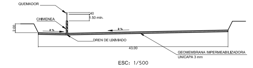
DETALLE DE SECCIÓN A-A
