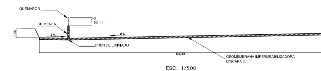
DETALLE DE SECCIÓN C-C
