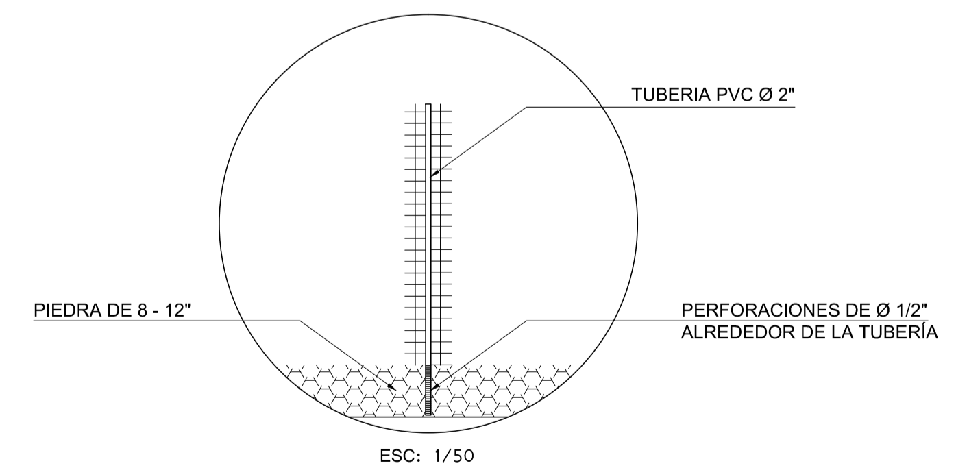
DETALLE 1 DE TUBERÍA DE MONITOREO
