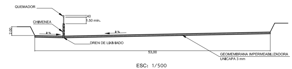
DETALLE DE SECCIÓN B-B
