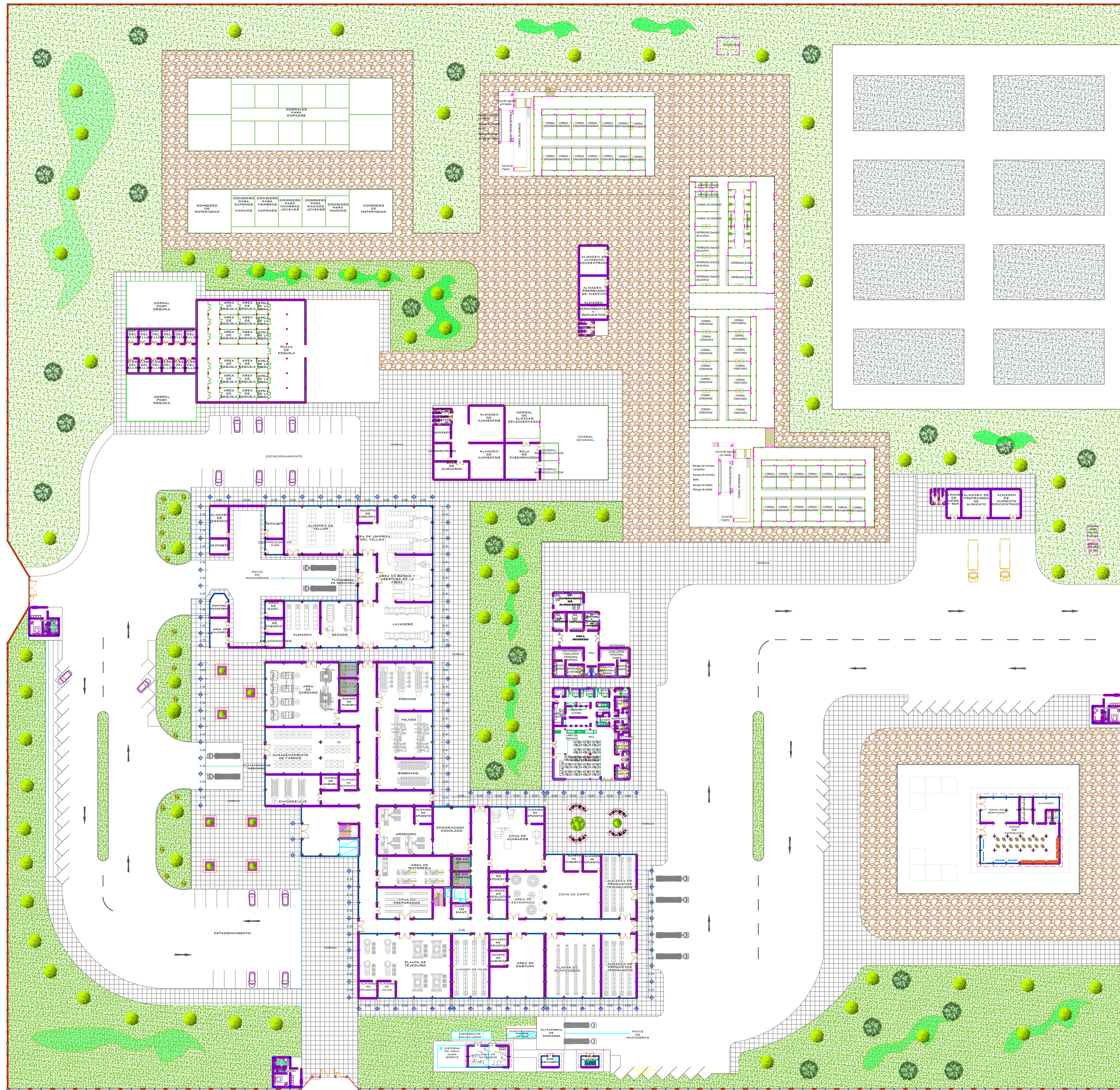
PLANIMETRÍA GENERAL
