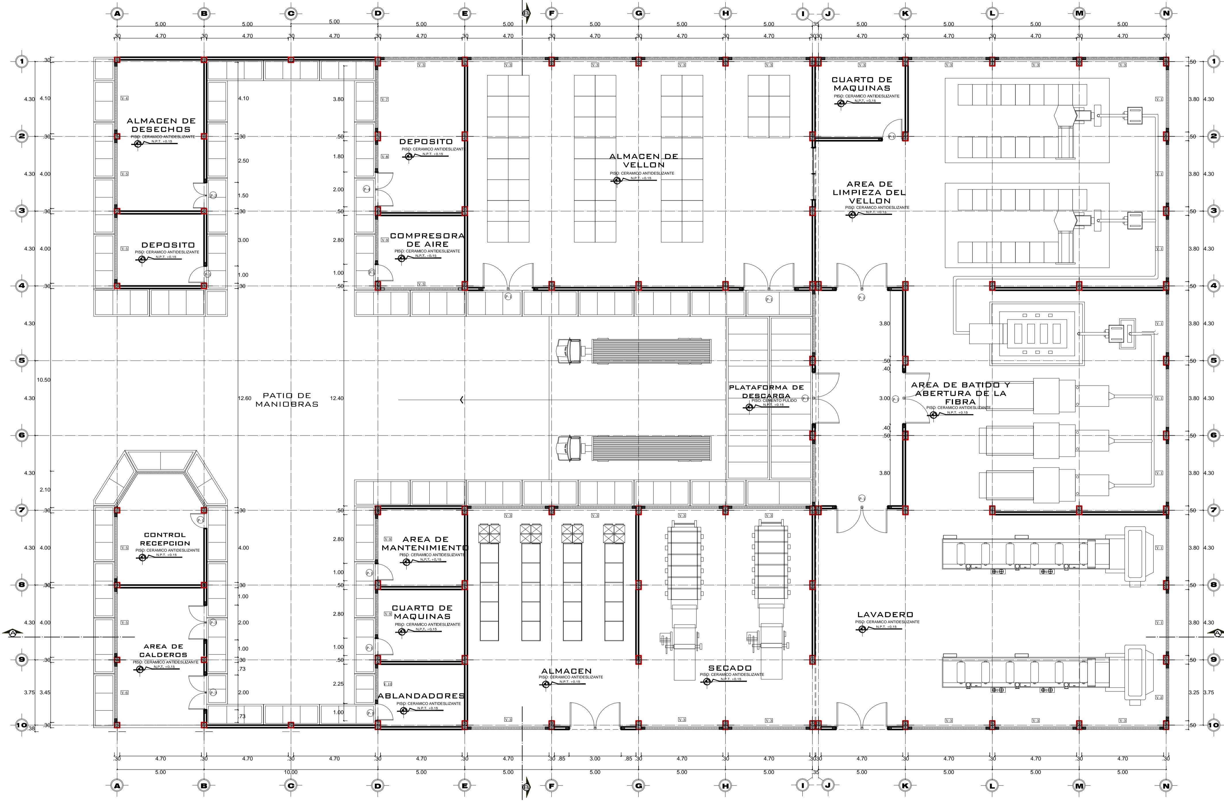
ZONA DE LAVADO PLANTA GENERAL ESC: 1/125
