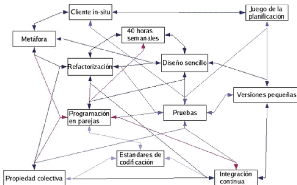
Figura 02: Prácticas XP
