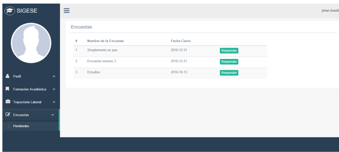
Figura 15: Pantalla Encuestas
