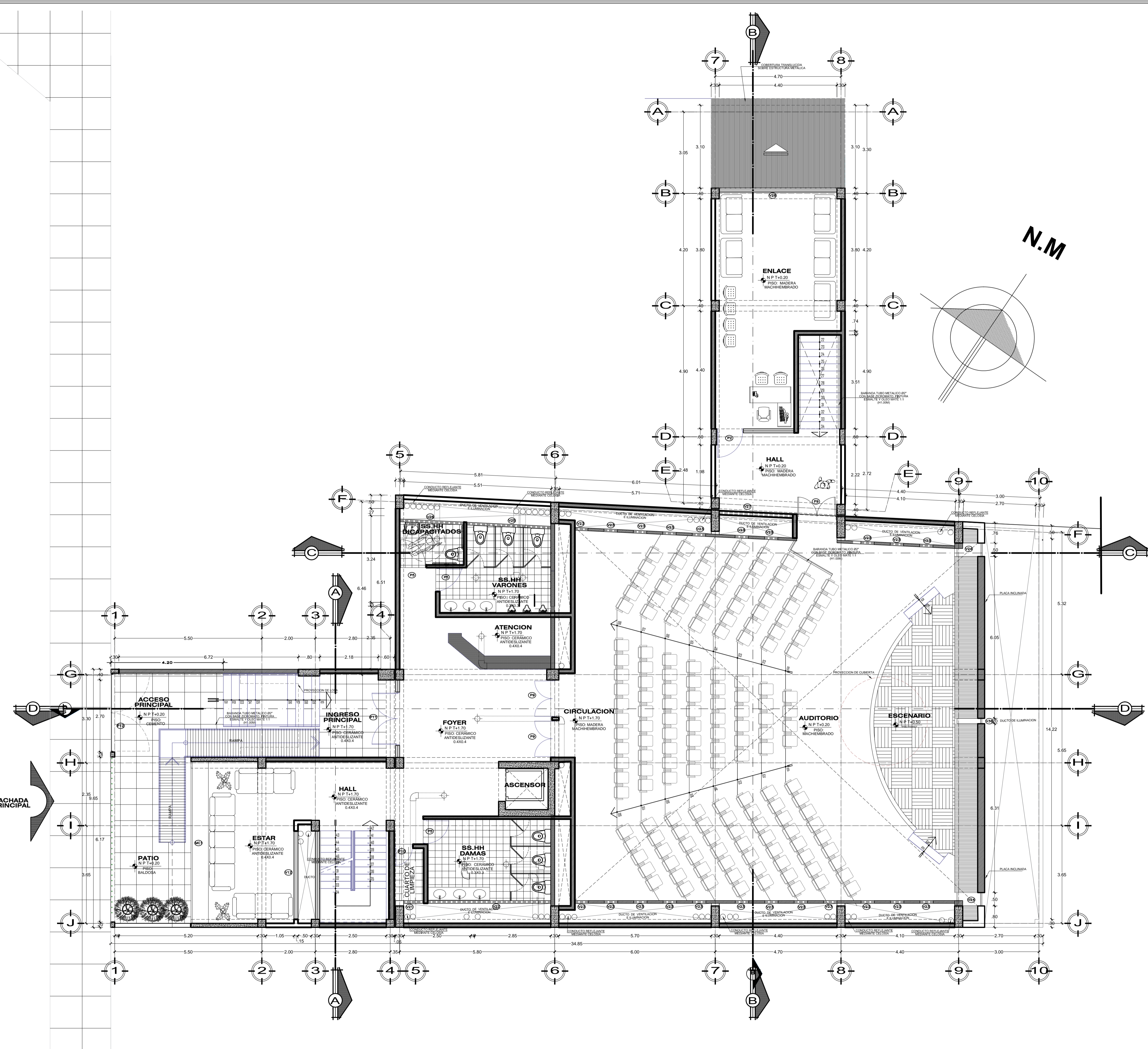
PLANTA DE DISTRIBUCION 1° NIVEL AV. LAYKAKOTA "TEMPLO PARA LA IGLESIA MARANATA PUNO" ESC. 1/75
