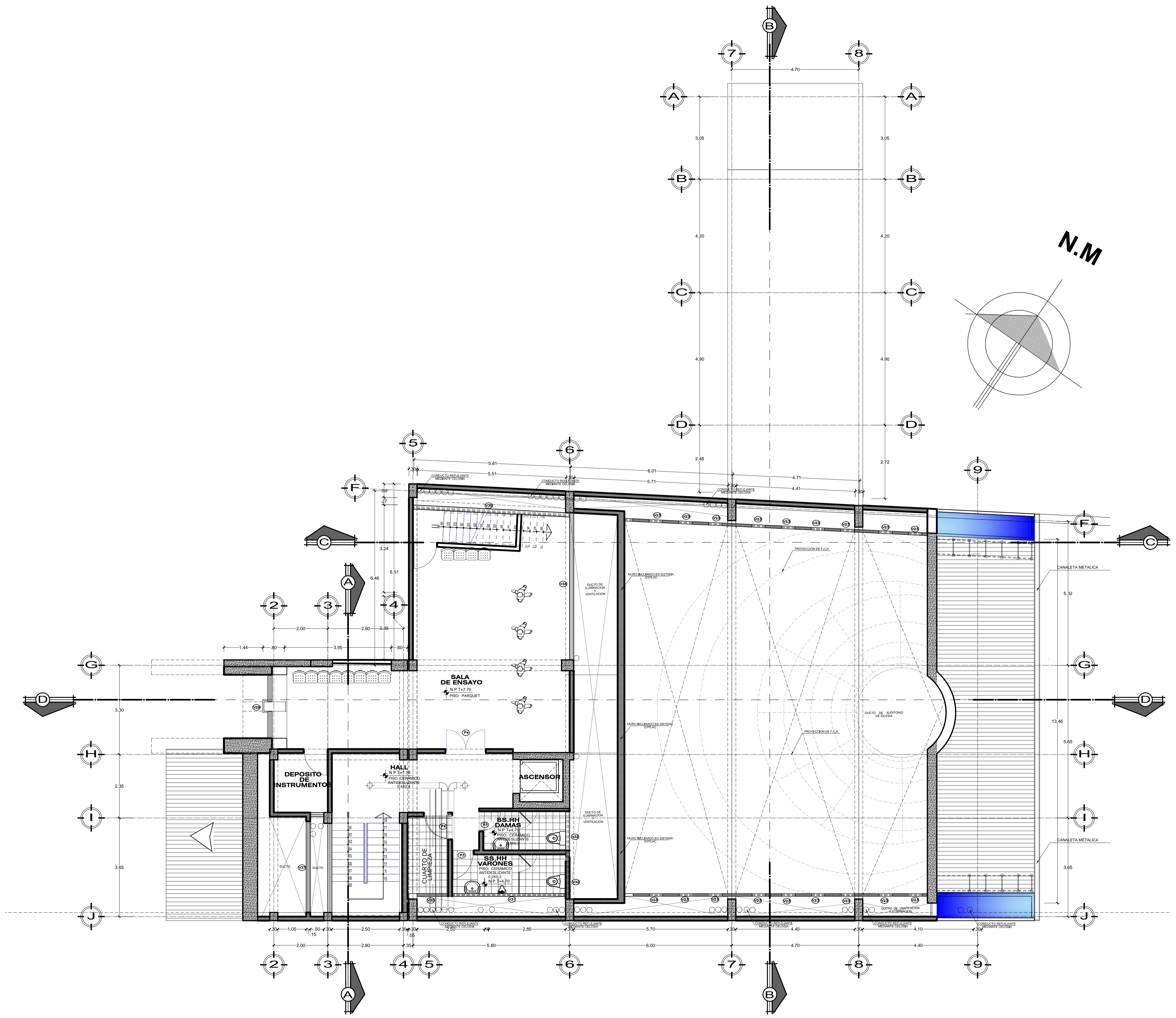
PLANTA DE DISTRIBUCION TERCER NIVEL AV. LAYKAKOTA "TEMPLO PARA LA IGLESIA MARANATA PUNO"
