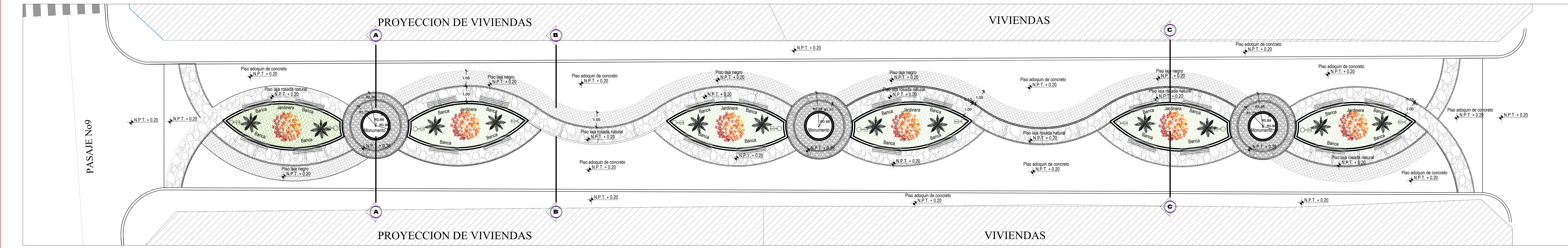
PLANTA - JR. TUPAC YUPANQUI ESCALA 1:100
