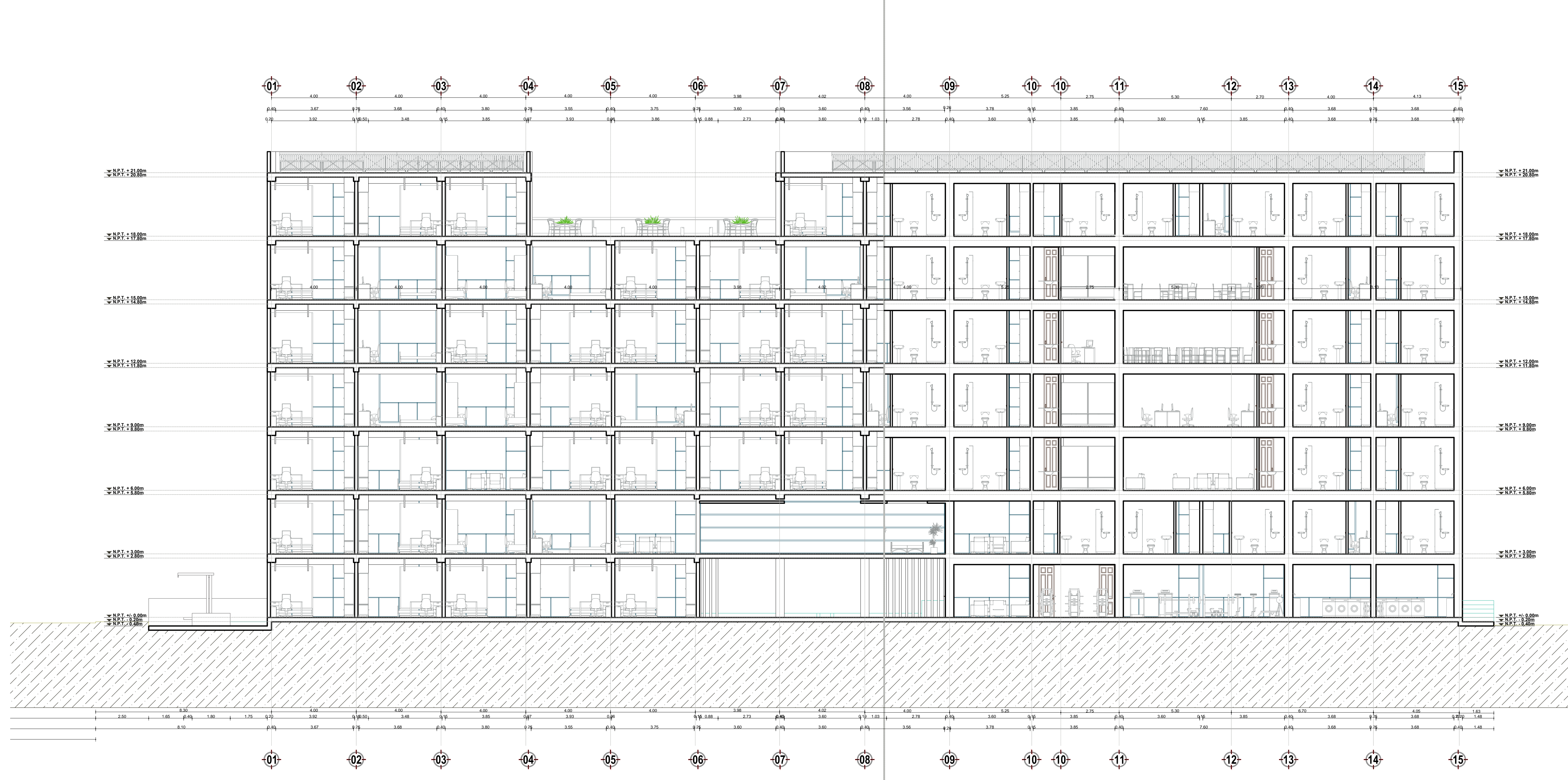
PLANO DE SECCION B-B VISTA DEL - BLOQUE DAMAS ESC: 1/100
