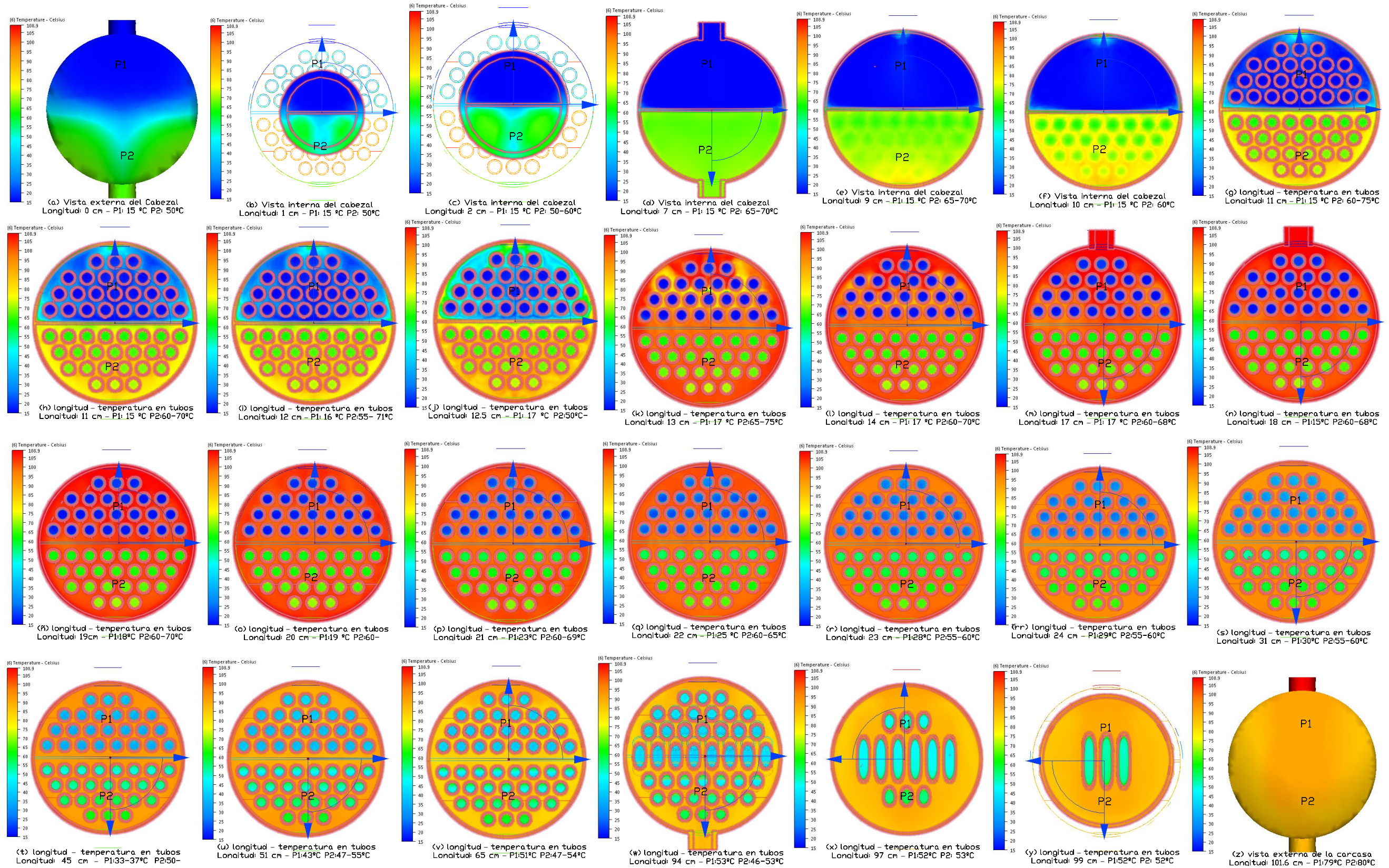
Figura 38: Corte transversal del intercambiador de calor de tubos y carcasa. Donde podemos diferenciar la parte del cabezal desde la figura (a) hasta la (j), y de la (k) a la (z) el resto de la carcasa. P1: primer paso (24 tubos), P2: segundo paso (24 tubos). Longitud de extremo a extremo 101.6 cm (Fuente: propia).
