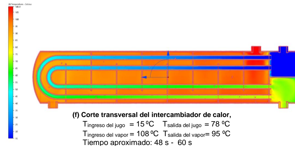
Figura 37: Avance térmico aproximado de los fluidos dentro del intercambiador de calor de tubos y carcasa 1-2 (Fuente: propia).
