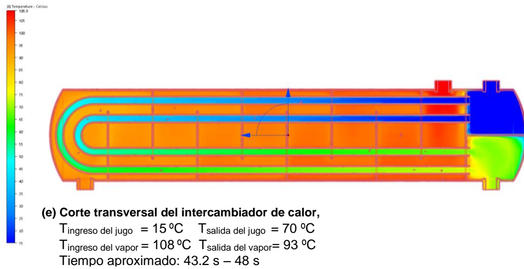
Figura 37: Avance térmico aproximado de los fluidos dentro del intercambiador de calor de tubos y carcasa 1-2 (Fuente: propia).
