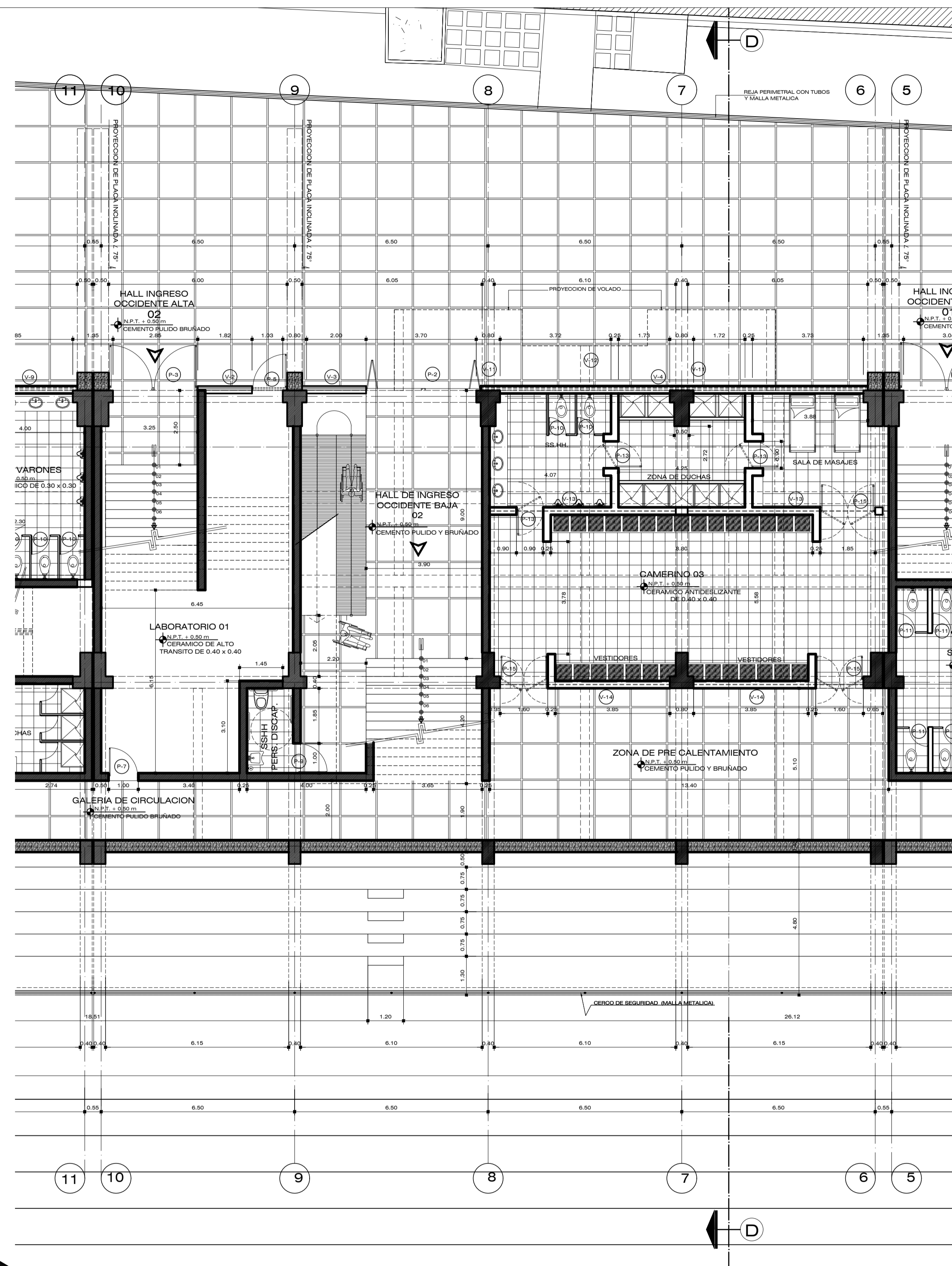
PLANTA DE DISTRIBUCION PRIMER NIVEL - TRIBUNA OCCIDENTE BOLQUE II
