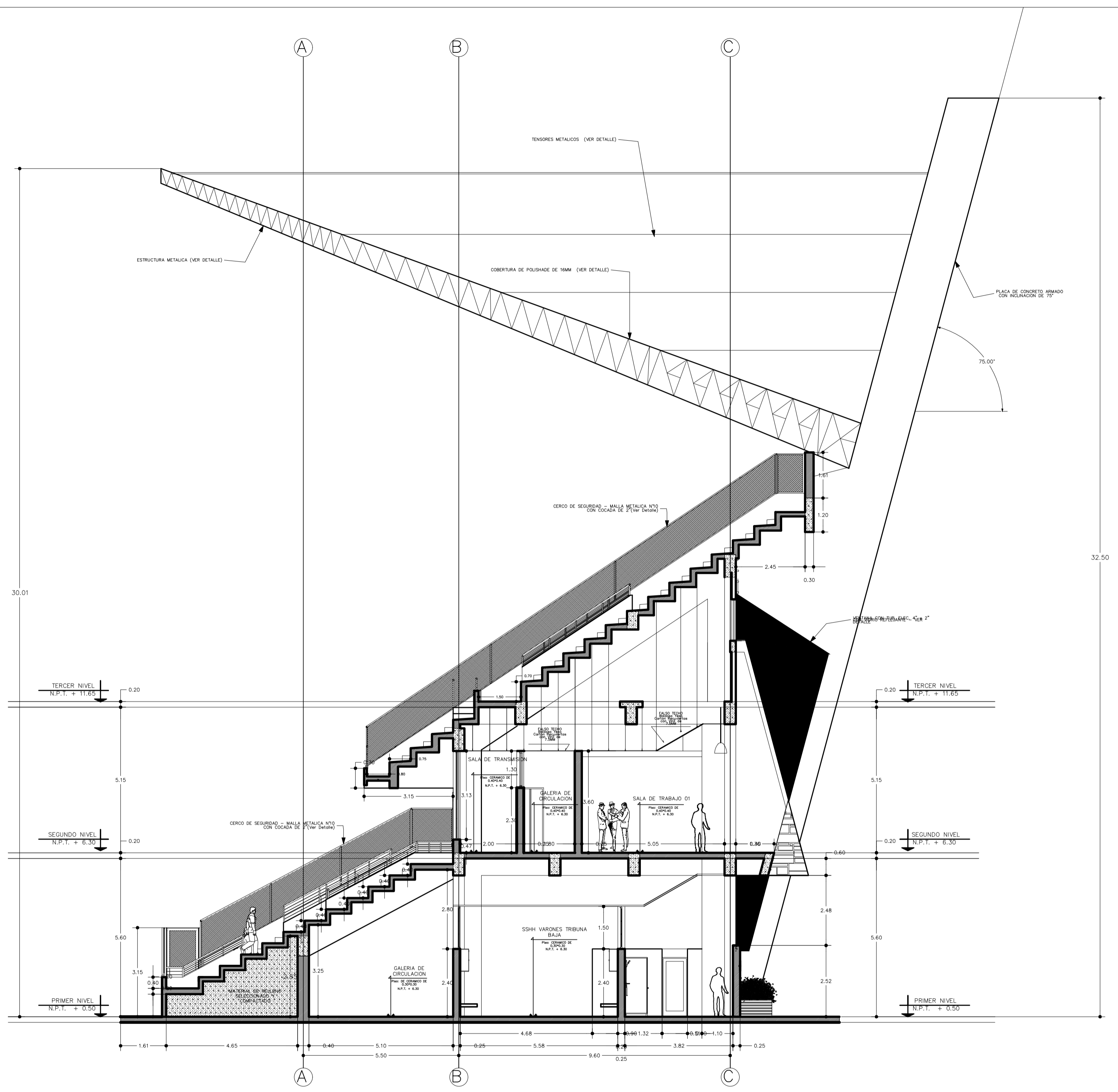
CORTE D-D
