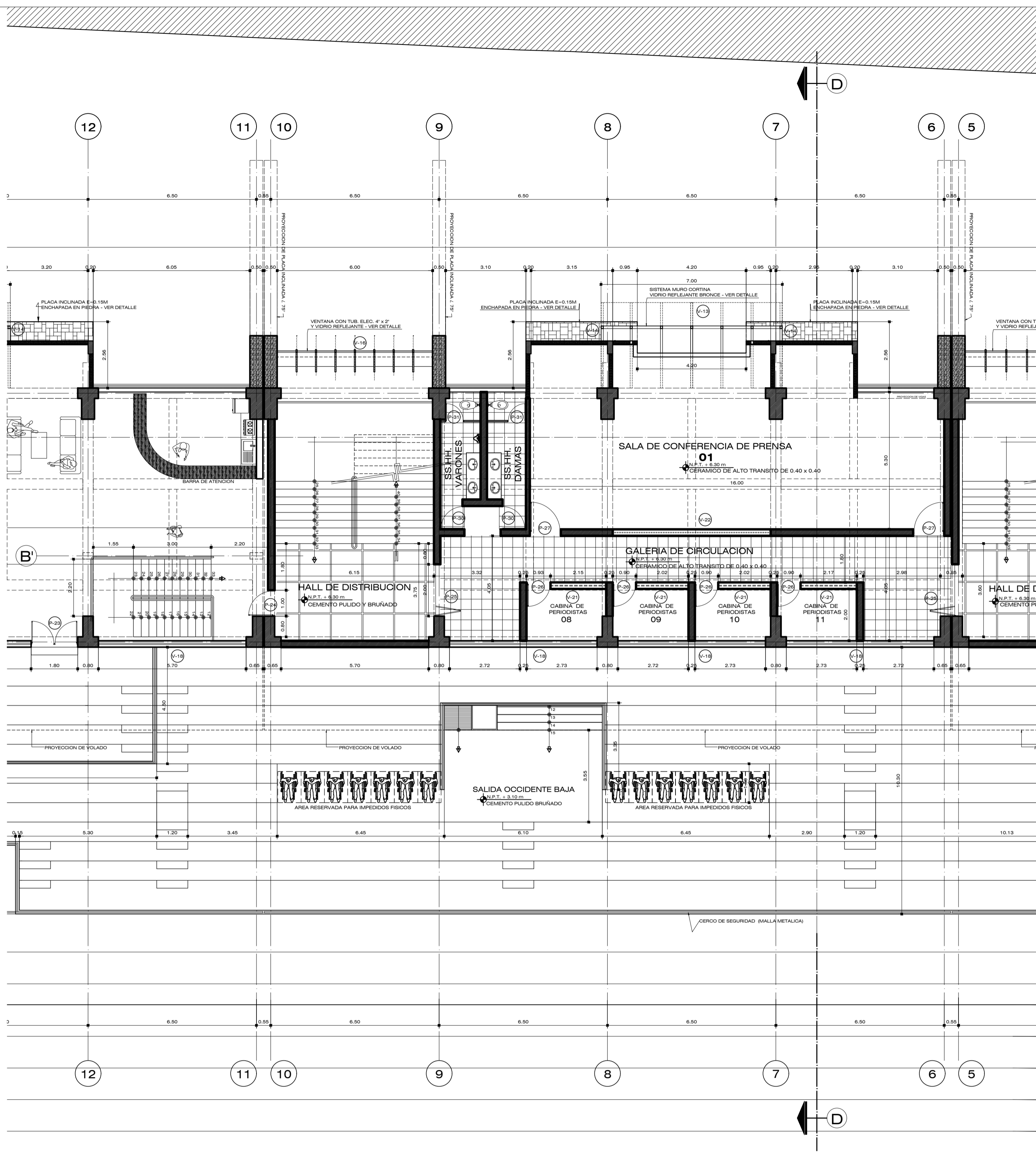
PLANTA DE DISTRIBUCION SEGUNDO NIVEL - TRIBUNA OCCIDENTE BOLQUE II
