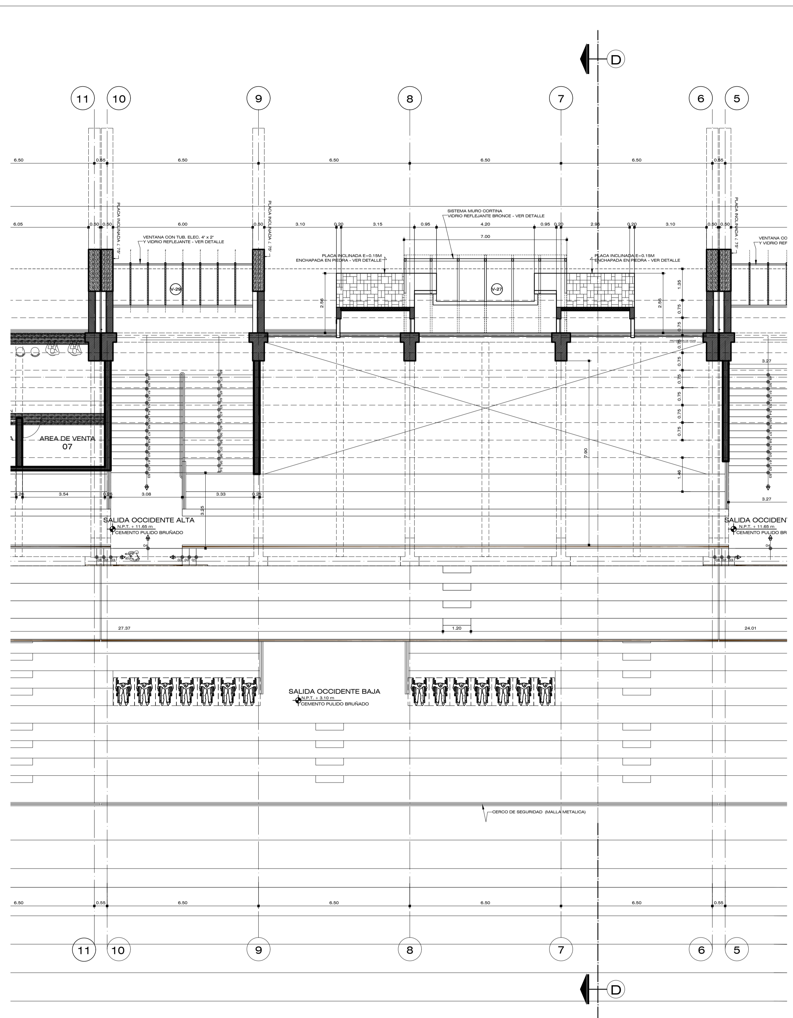
PLANTA DE DISTRIBUCION TERCER NIVEL - TRIBUNA OCCIDENTE BOLQUE II
