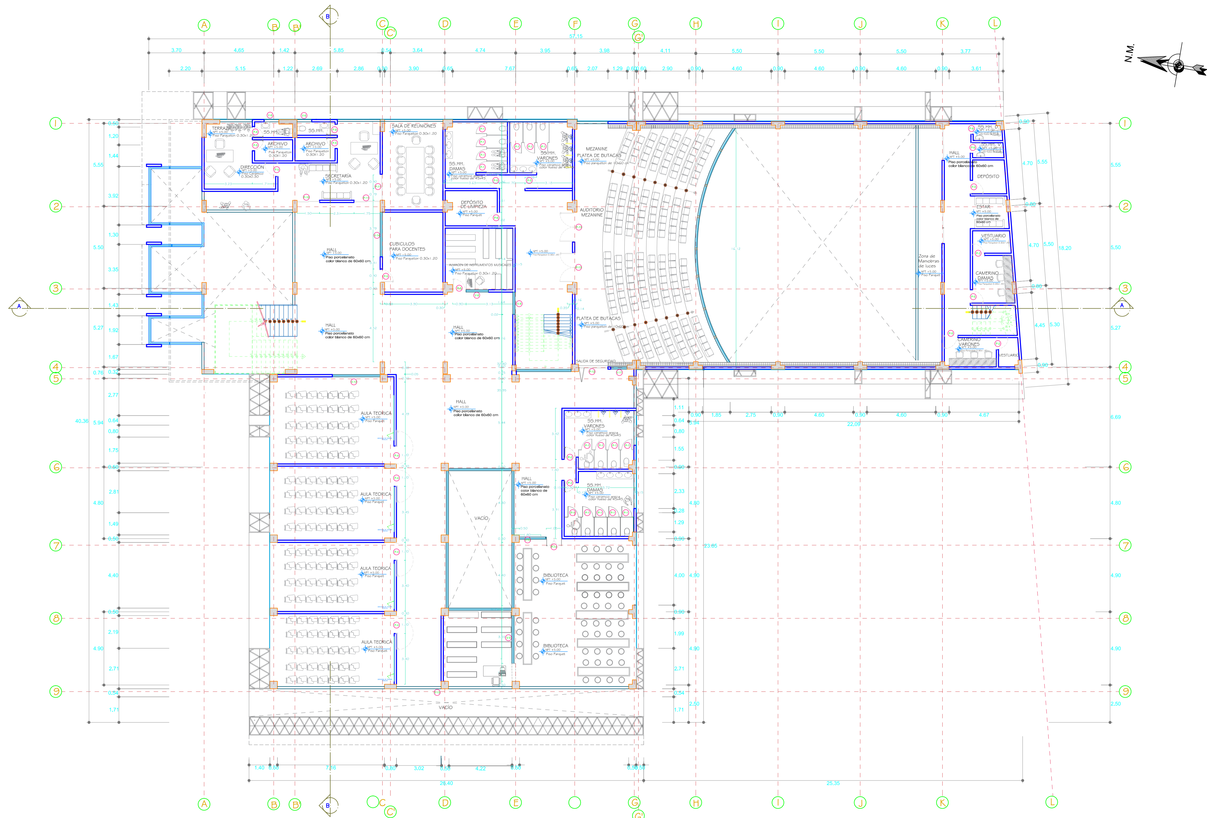
SEGUNDO NIVEL - PLANO EN PLANTA Esc: 1 / 200
