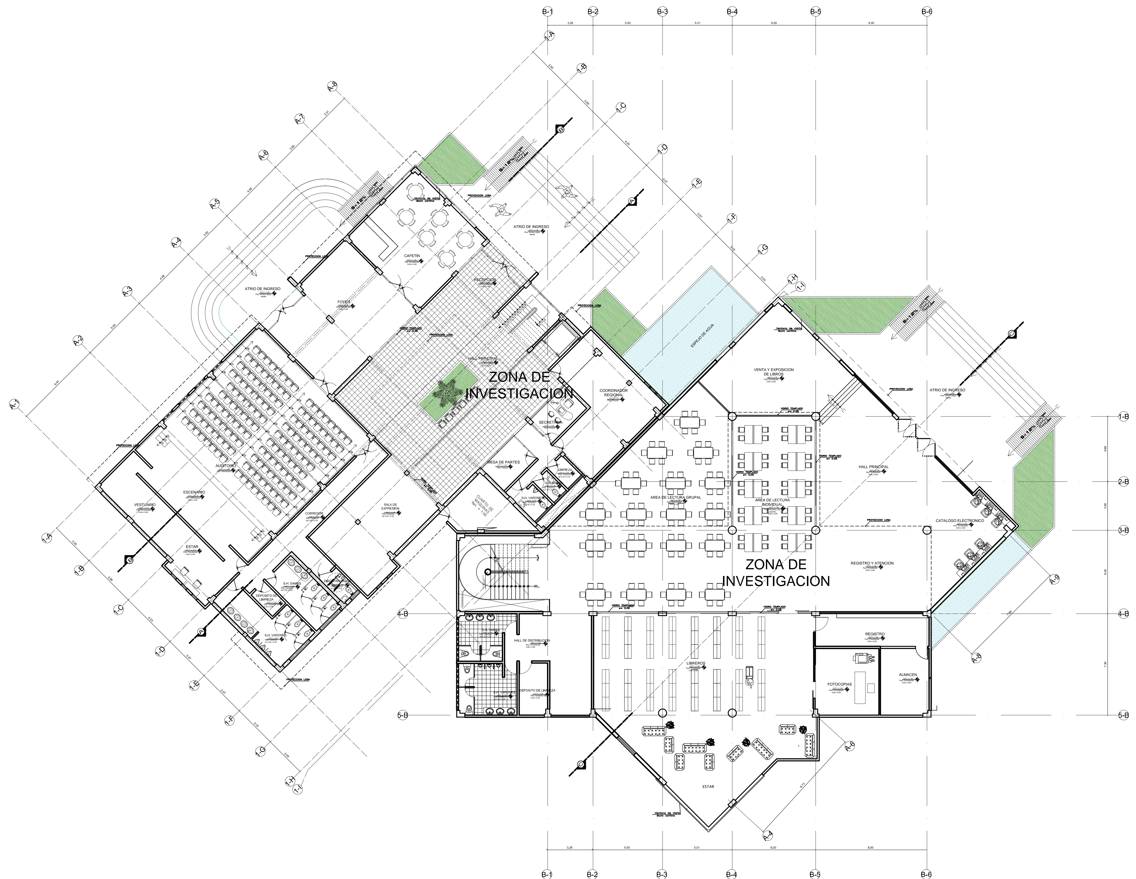
DISTRIBUCCION ARQUITECTONICA PRIMER NIVEL ZONA DE REVALORACION Y ADMINISTRATIVA
