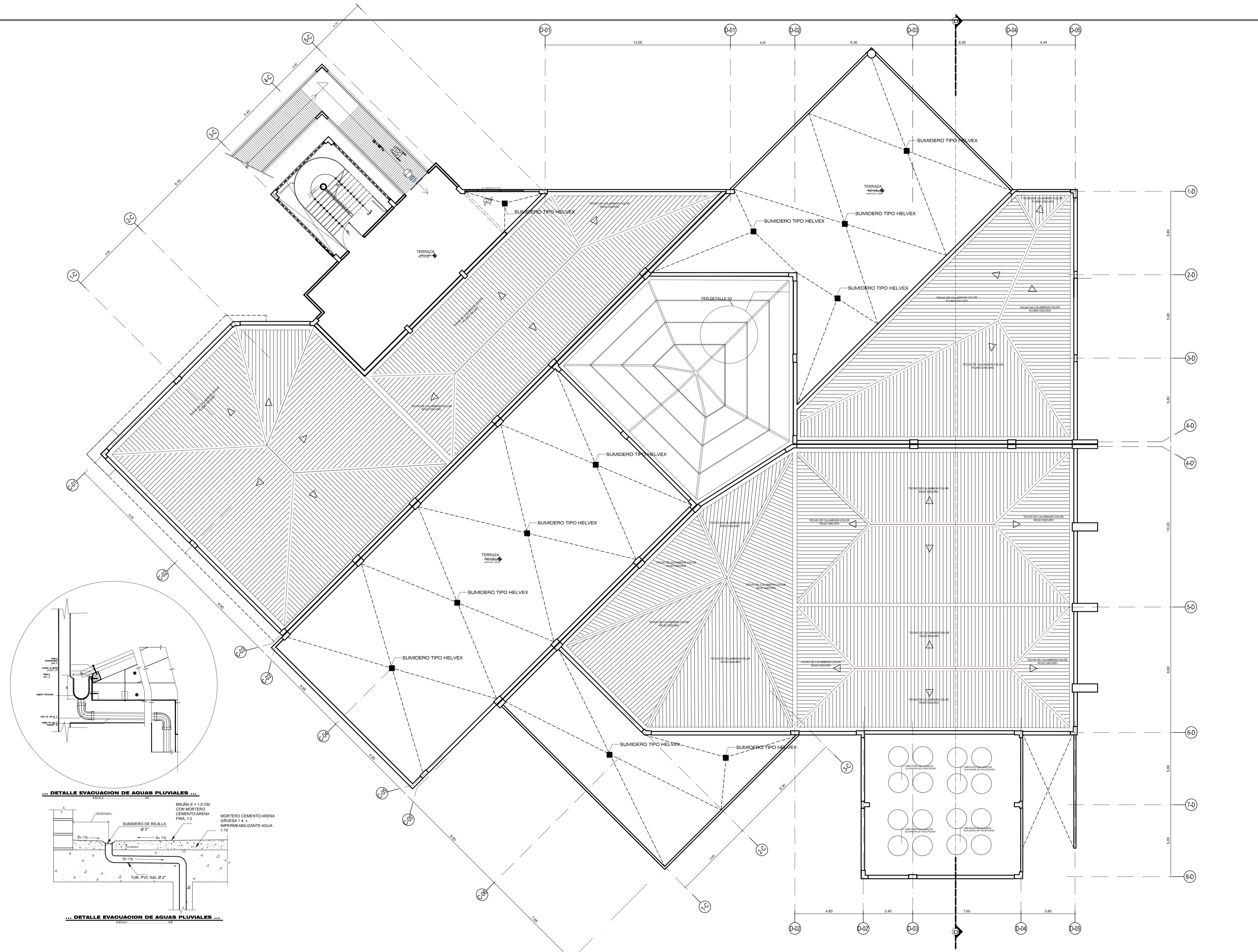
DISTRIBUCCION ARQUITECTONICA NIVEL BLOQUE D (EXHIBICION) ESCALA 1:125
