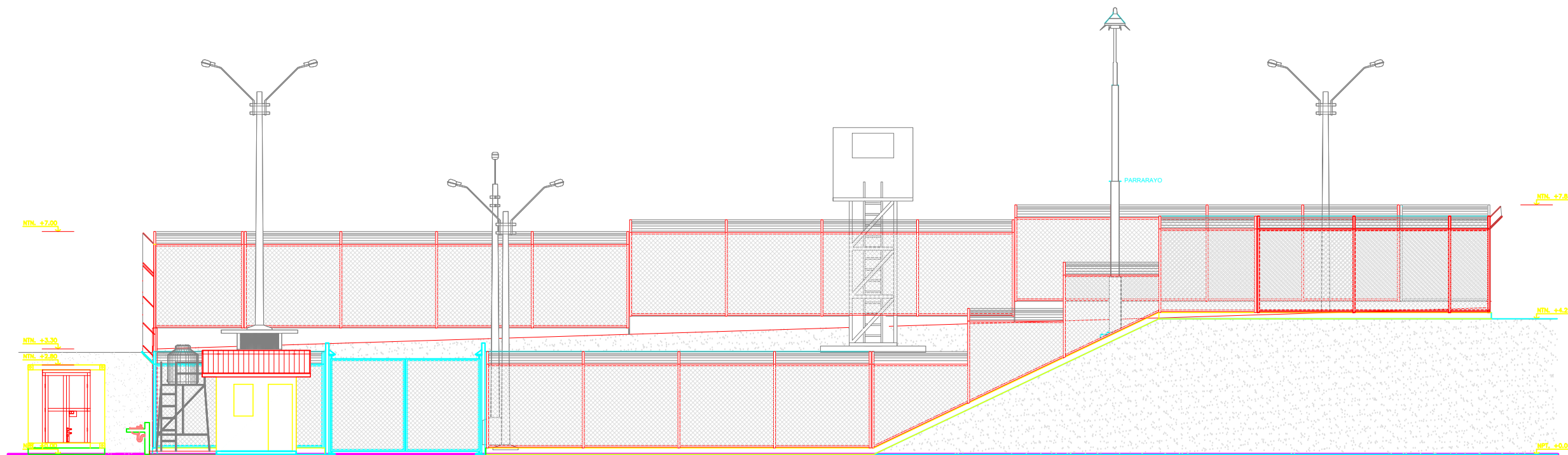
ELEVACION A-A
