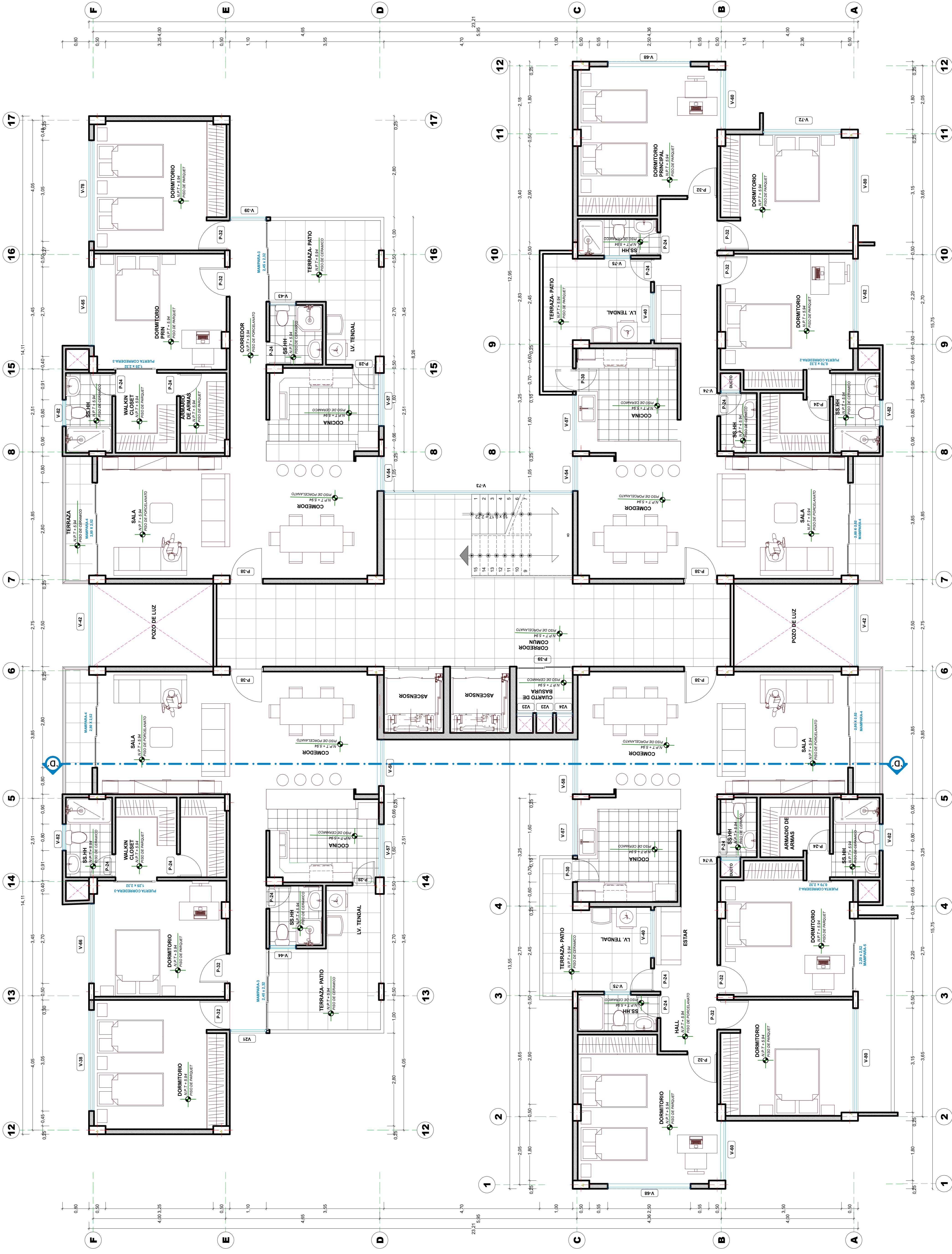
PLANTA DE DISTRIBUCION DEL 10ER AL DECIMO CUARTO NIVEL
