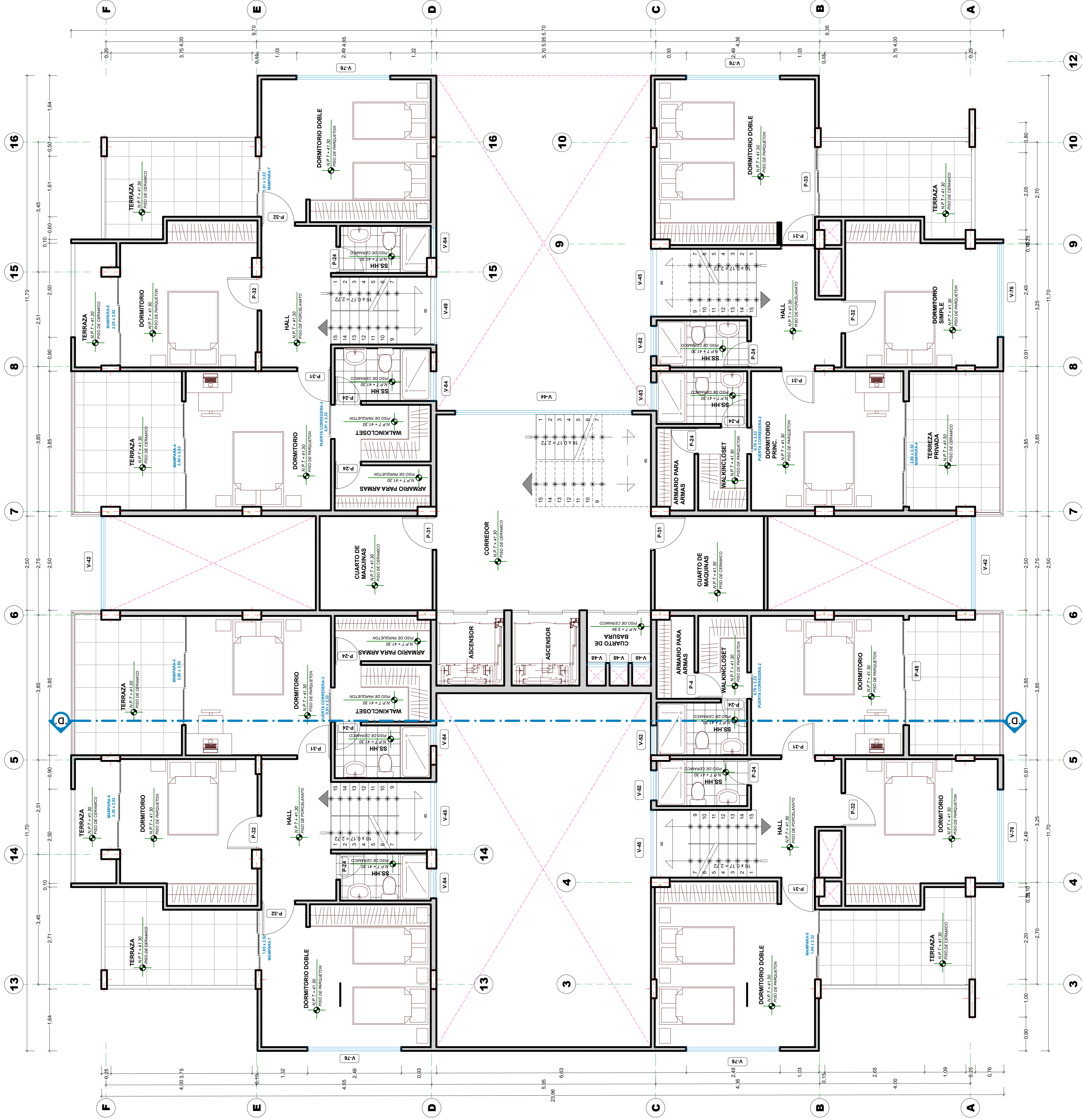
PLANTA DE DISTRIBUCION DECIMO SEXTO NIVEL ESC. 1/50
