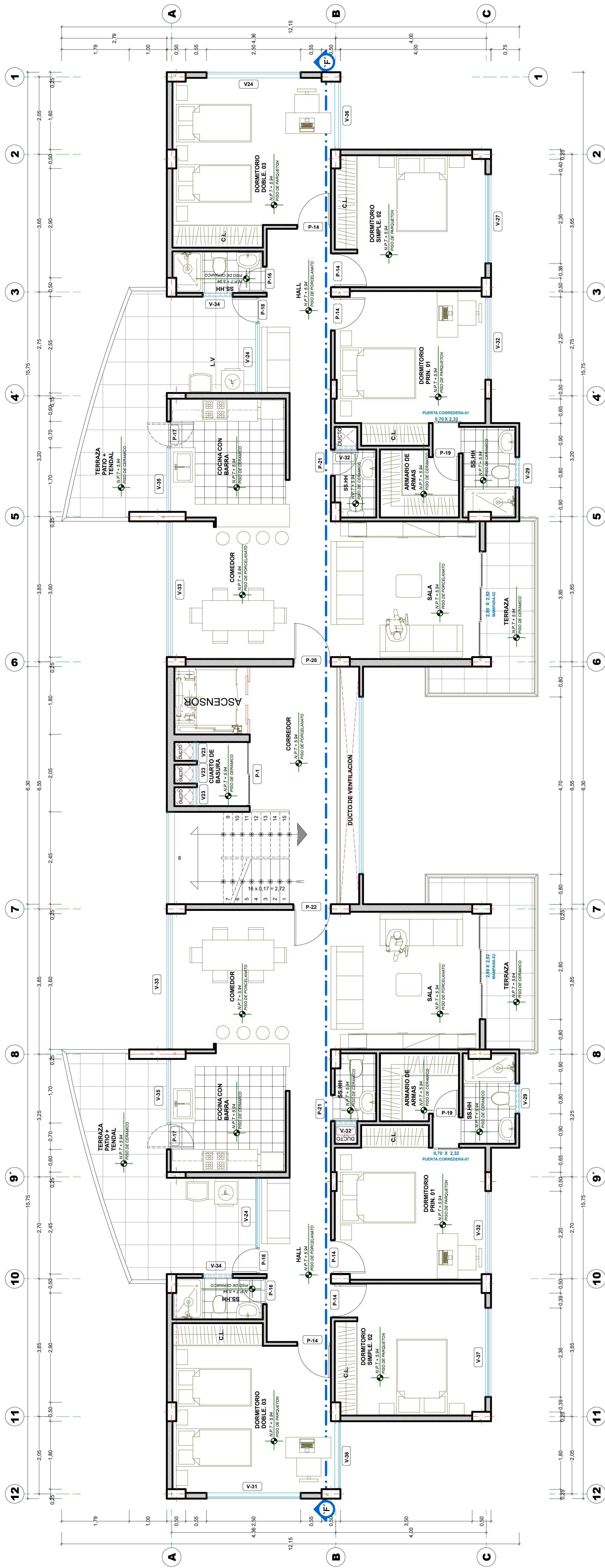
PLANTA DE DISTRIBUCION TIPICA (MODULO DE VIVIENDA TIPO FLATS) ESC: 1/30
