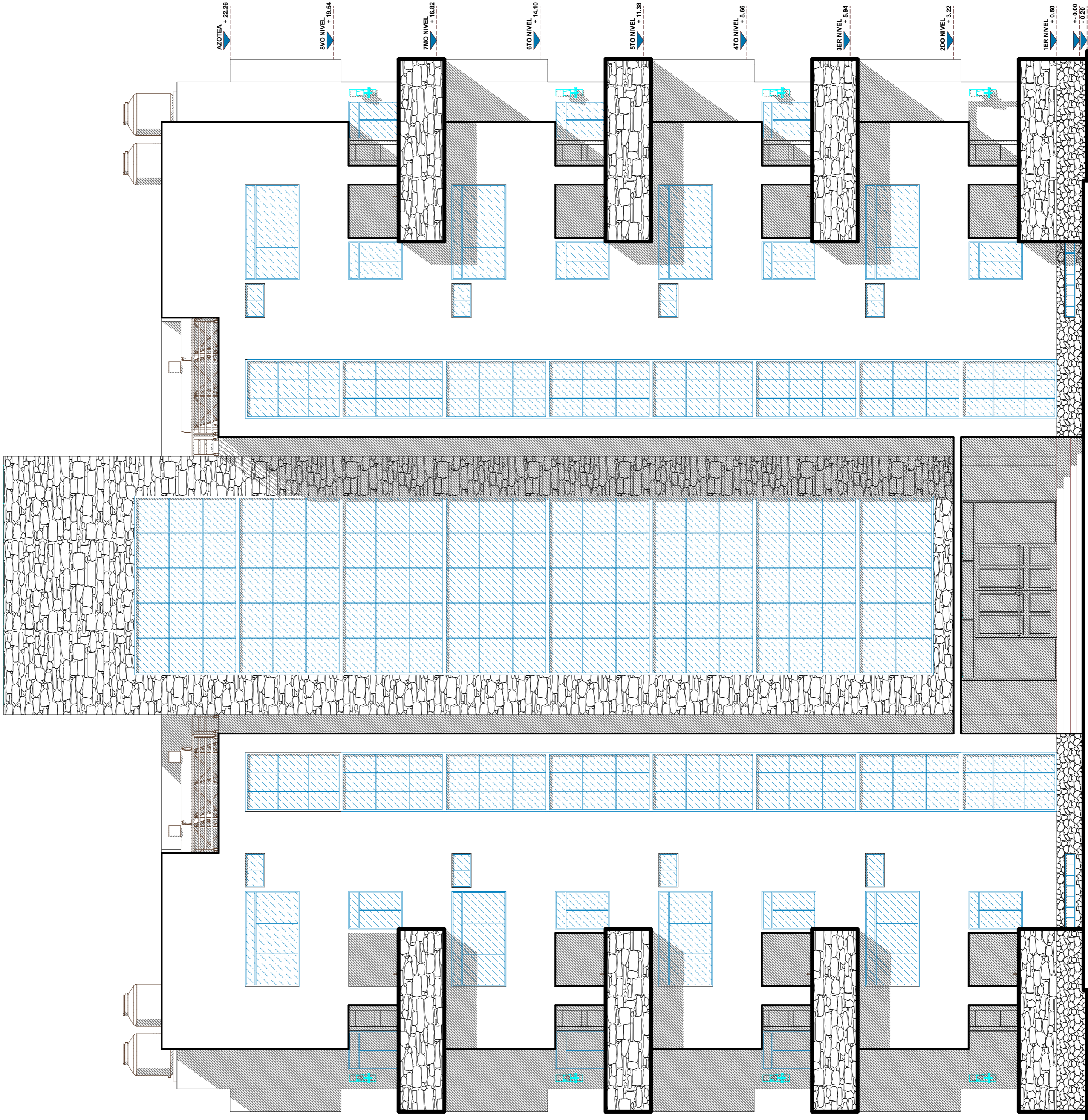
FACHADA PRINCIPAL ESC. 1/75
