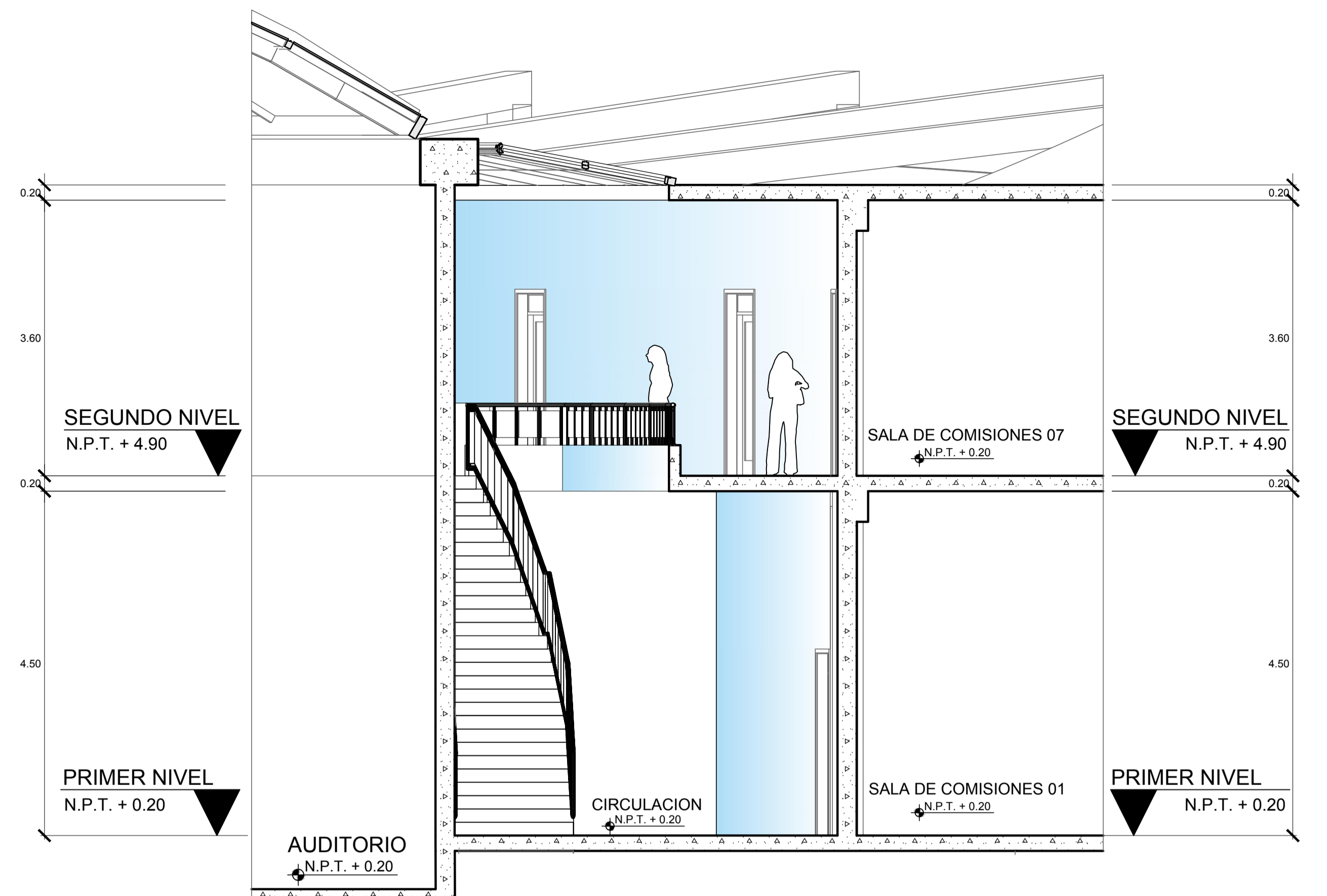
CORTE E-E SC: 1/50
