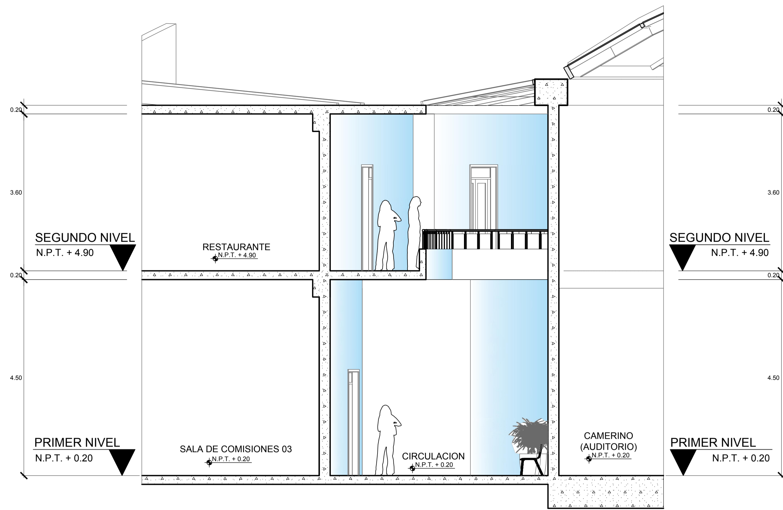
CORTE D-D SC: 1/50
