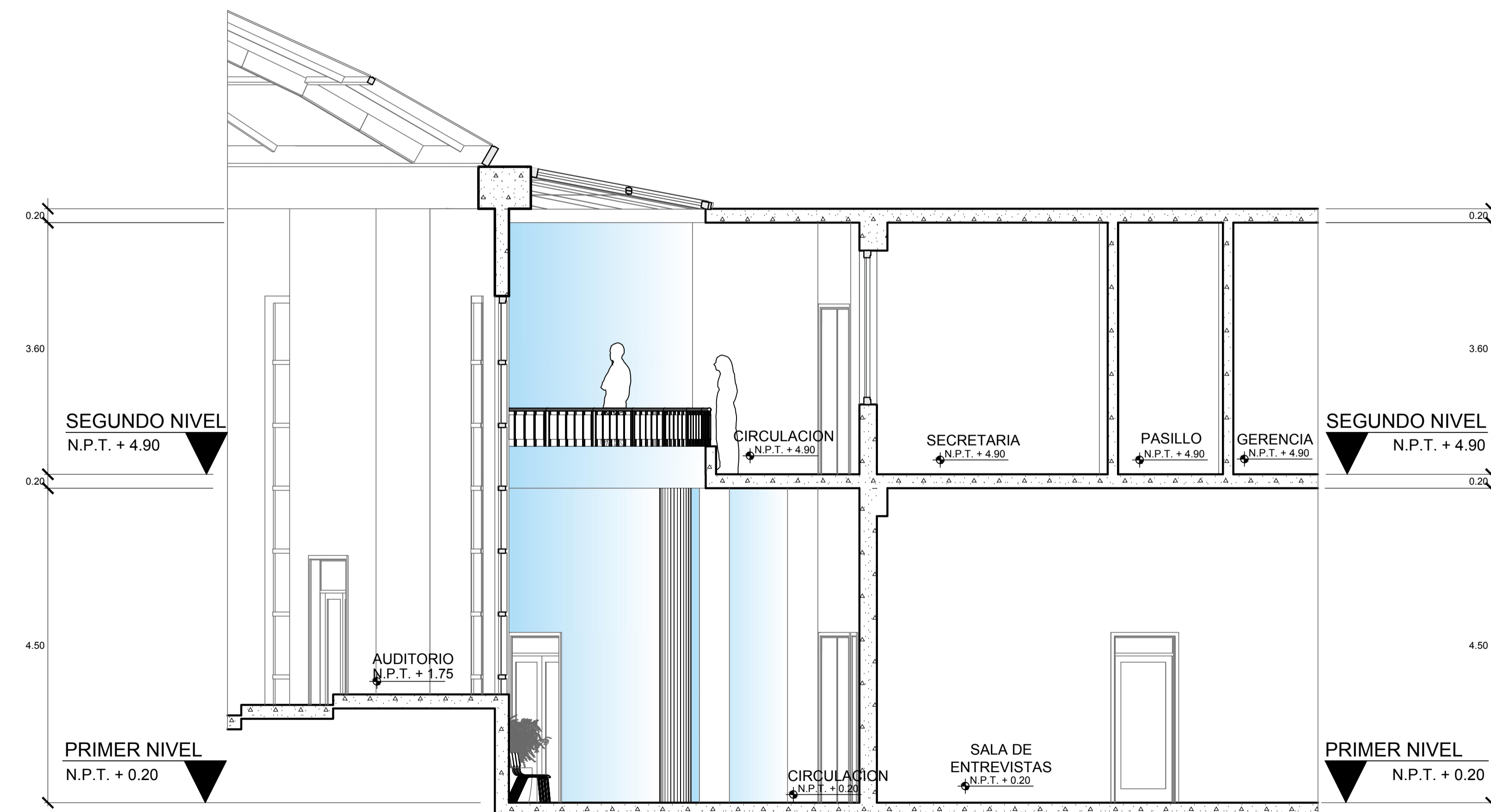
CORTE F-F SC: 1/50
