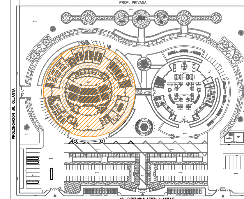
PLANIMETRIA ZONA DE CONVENCIONES
