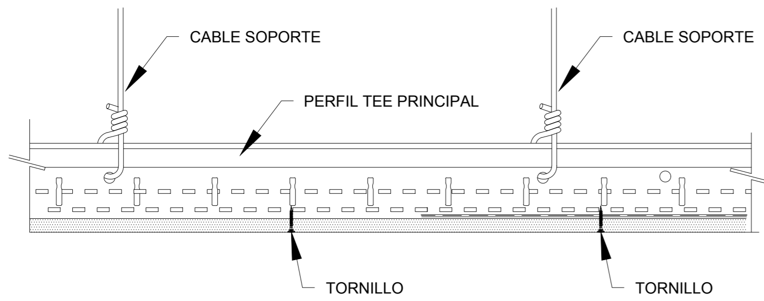
DETALLE 4 - CIELO RASO
