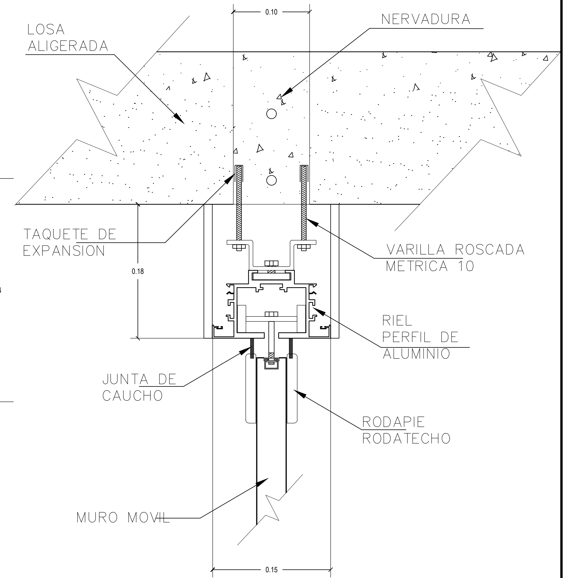
SECCION A - RIEL DE SUJECION SC: 1/5
