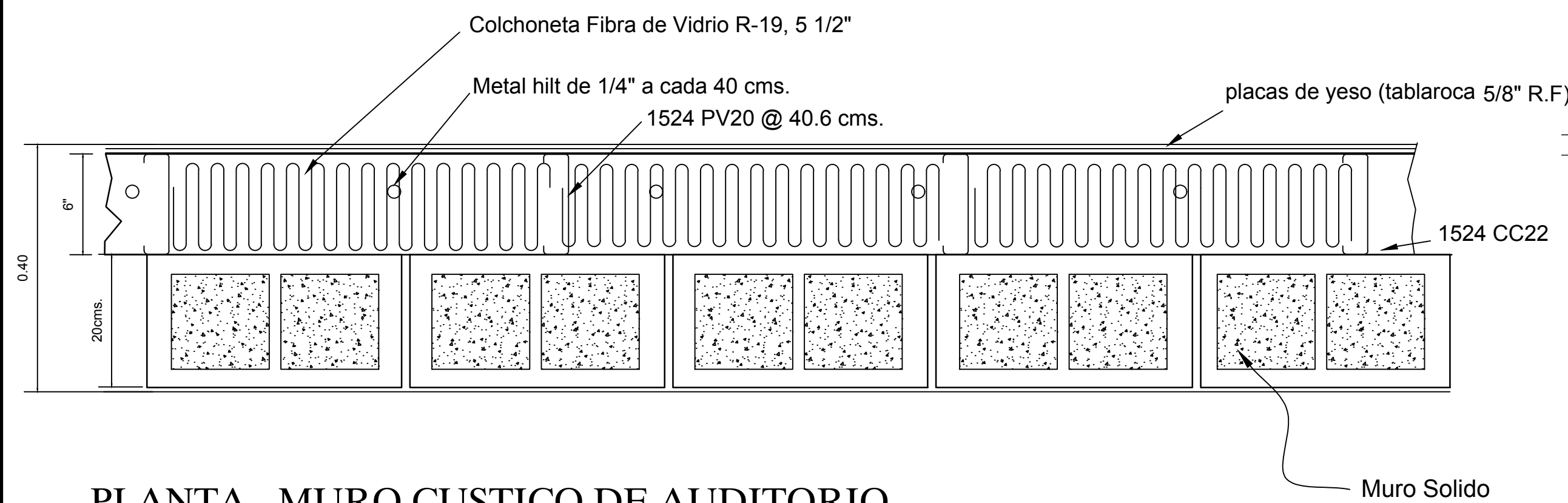
PLANTA - MURO CUSTICO DE AUDITORIO SC: 1/25
