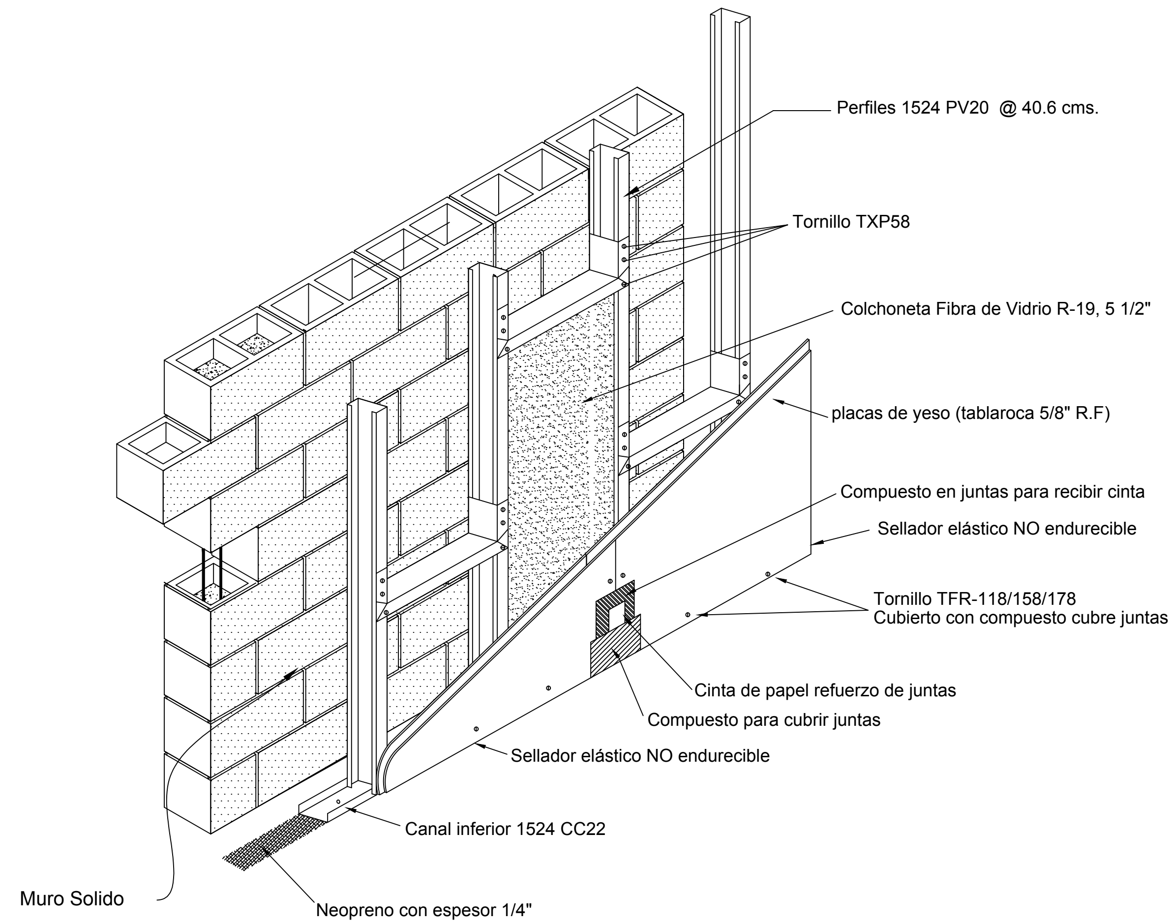
ISOMETRICO - MURO CUSTICO DE AUDITORIO
