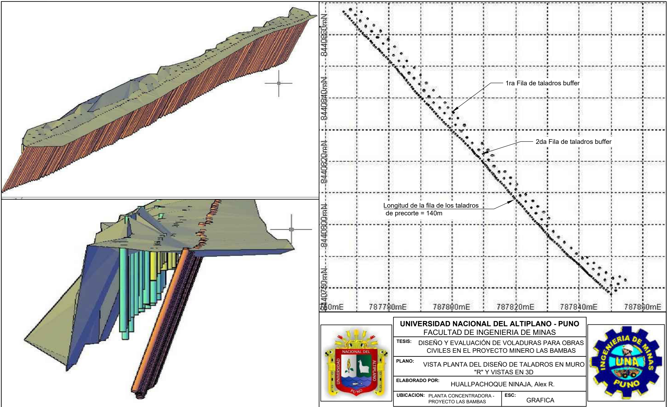
Figura N° 27: Vista planta del diseño de taladros en el muro "R" y vistas en 3D
