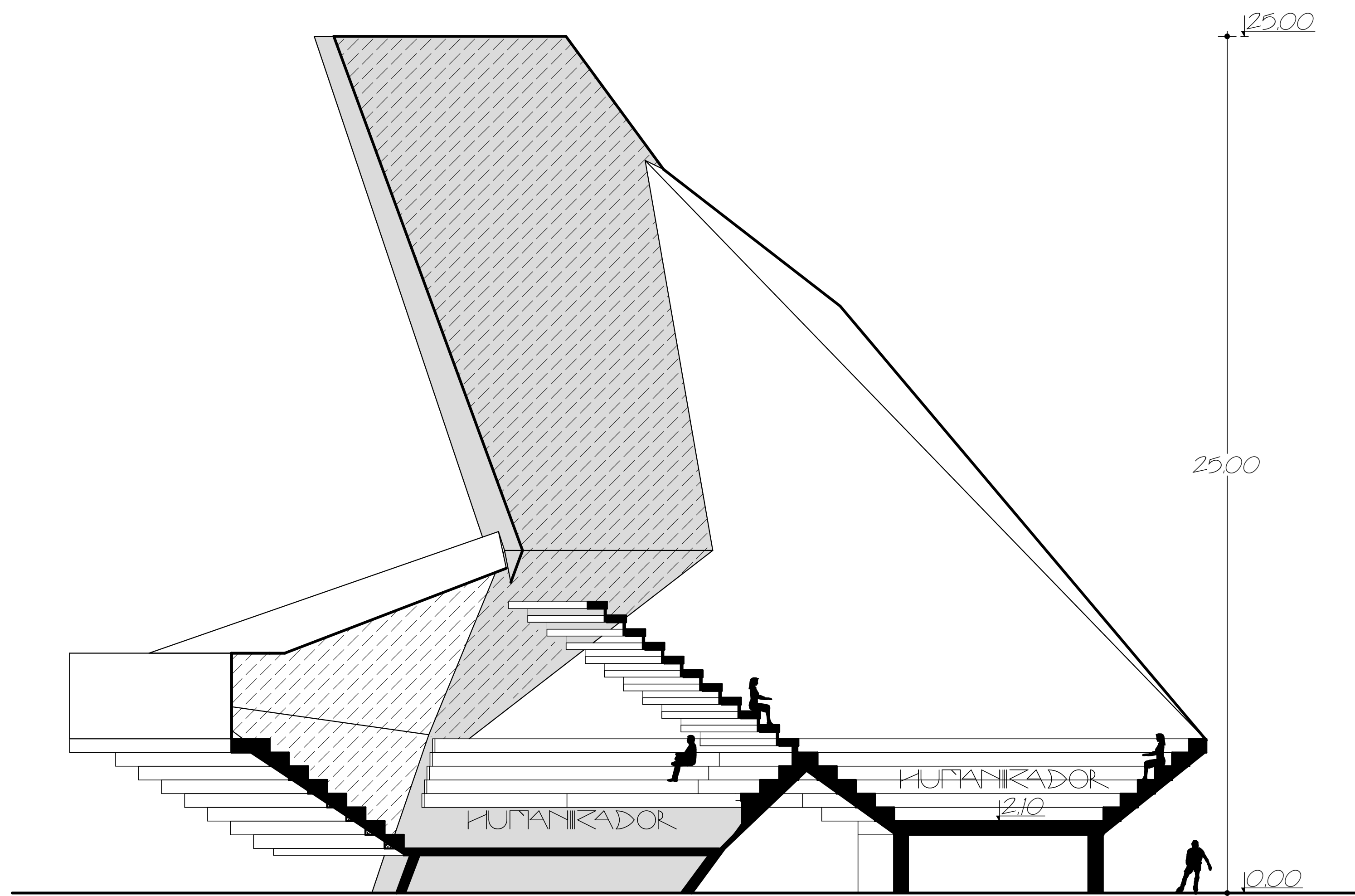
CORTE-2 E:1/100
