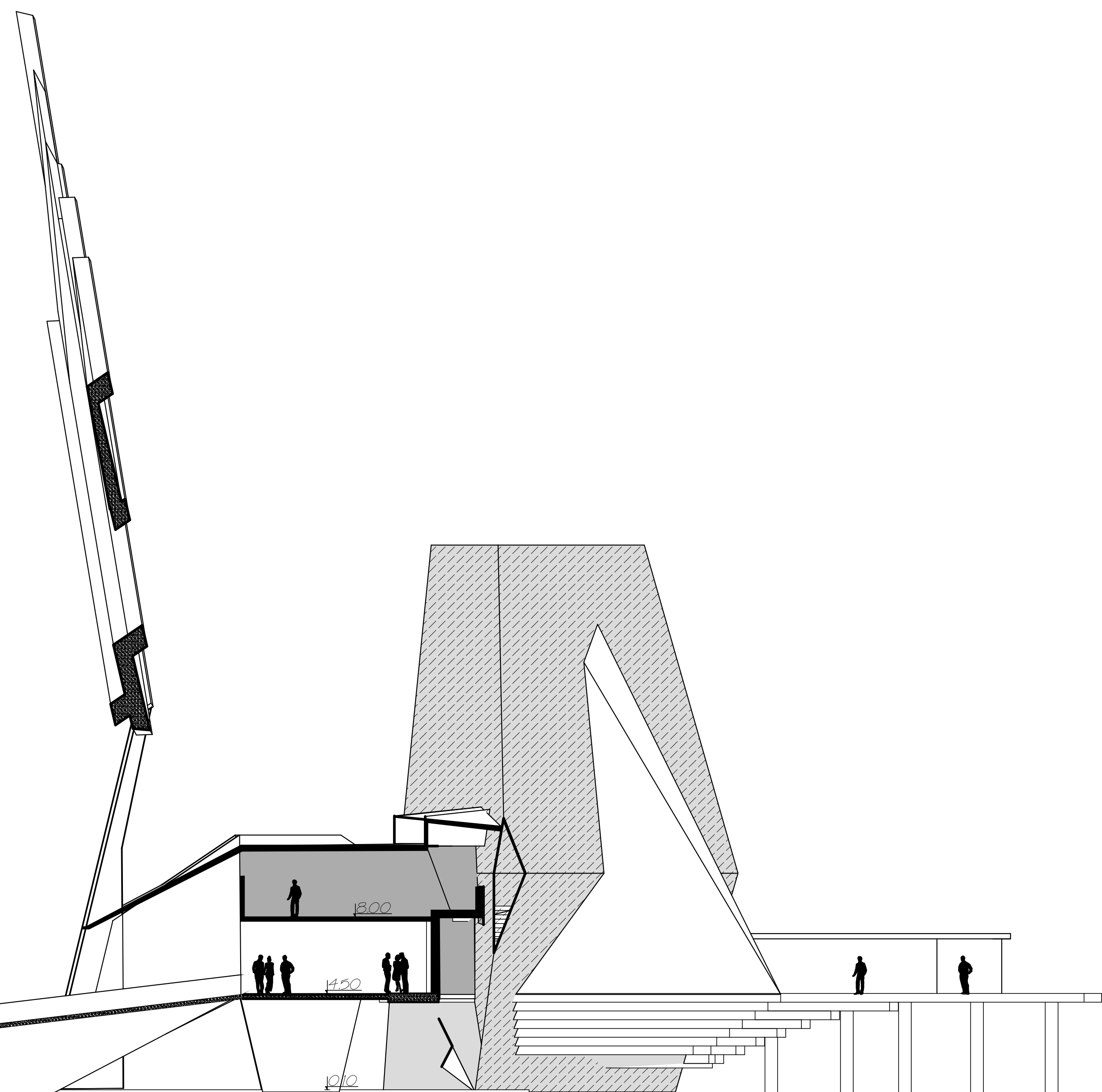
CORTE-1 E:1/150
