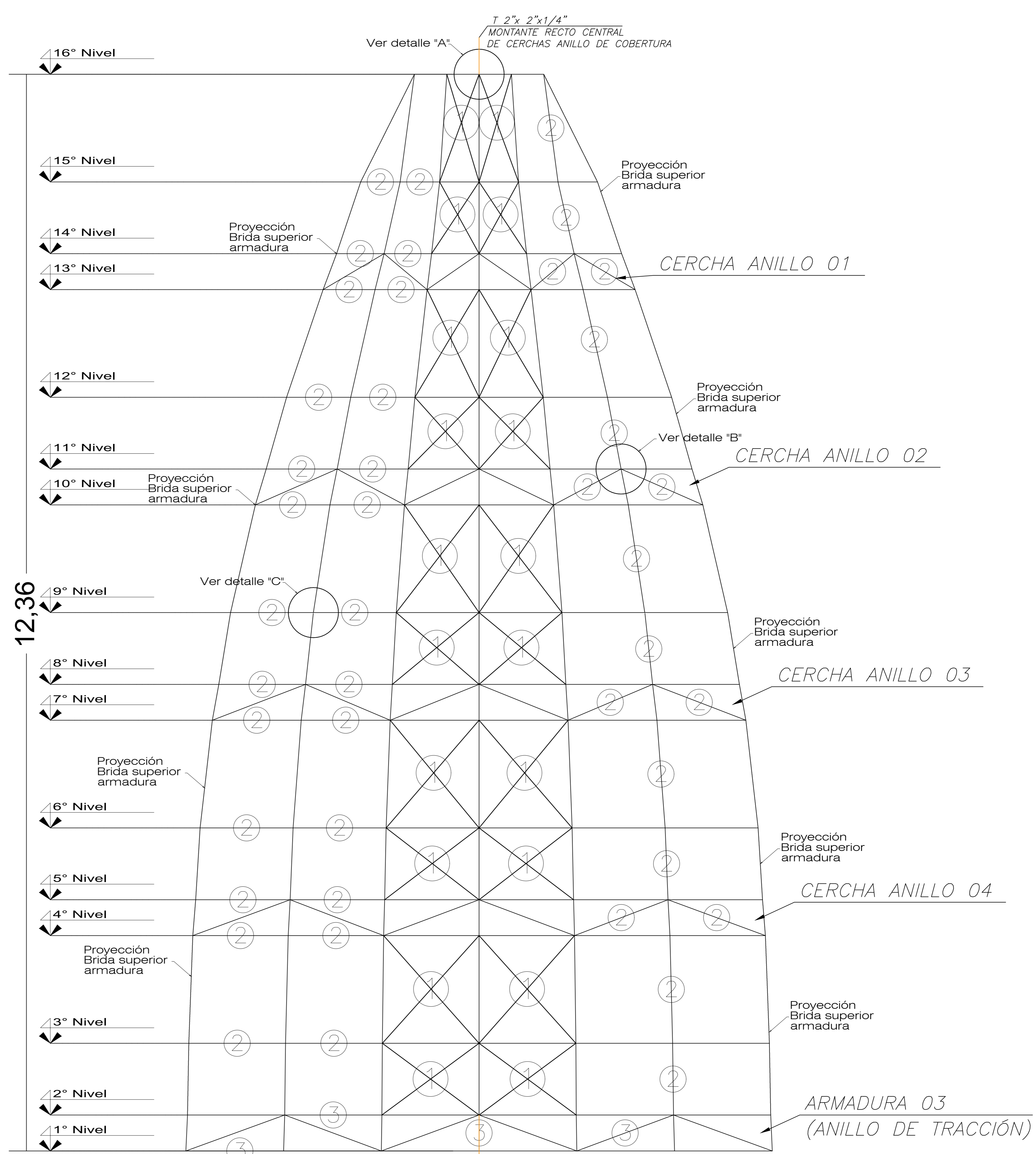
GAJO ESTRUCTURAL TIPO 1 C-I COMPOSICIÓN DE CERCHAS DE CERRAMIENTO C-CI-01
