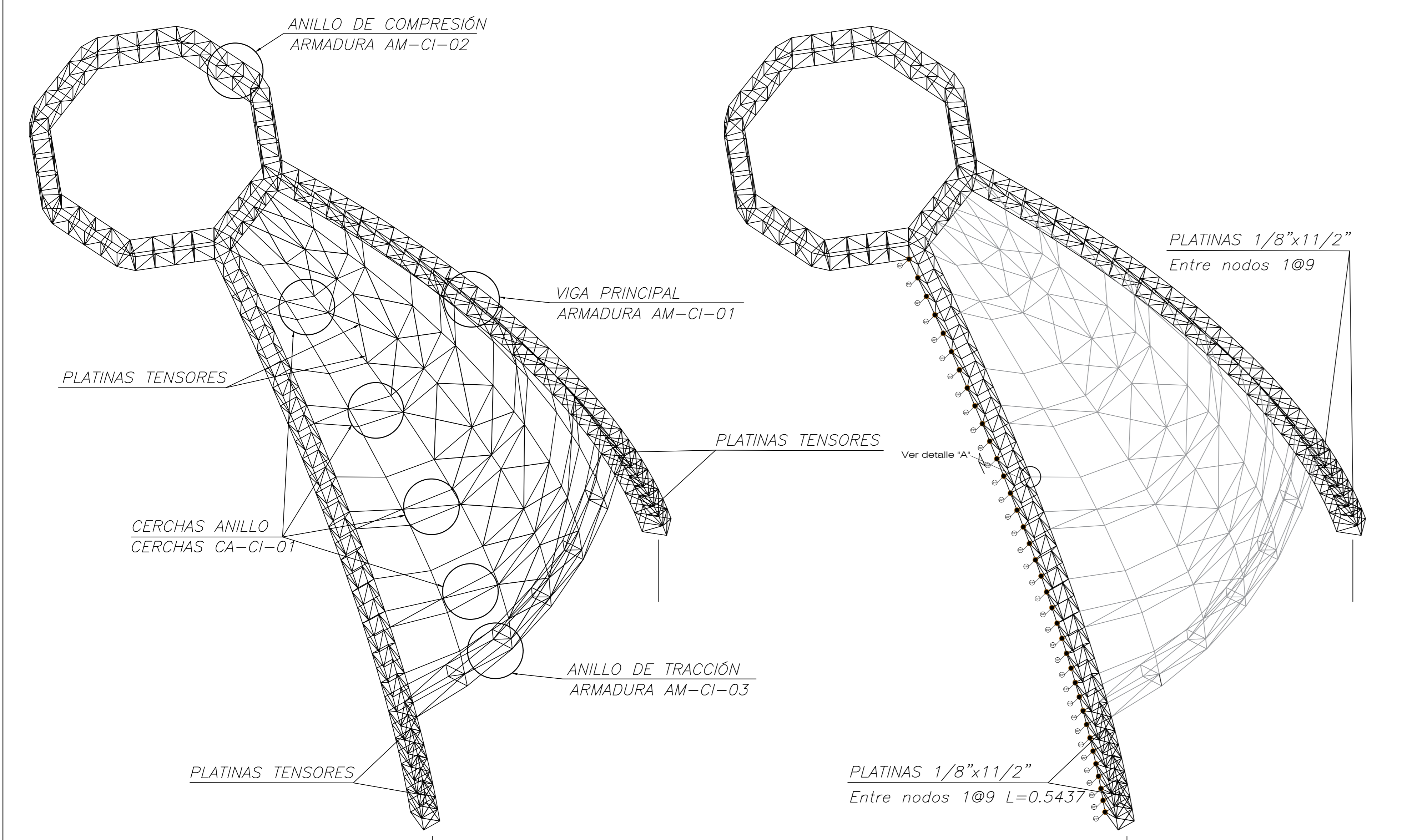
GAJO ESTRUCTURAL TIPO 1 CASCARÓN INTERNO COMPONENTES ESTRUCTURALES EN VISTA ISOMÉTRICA, NUMERACIÓN DE NODOS DE ARMADURA AM-CI-01
