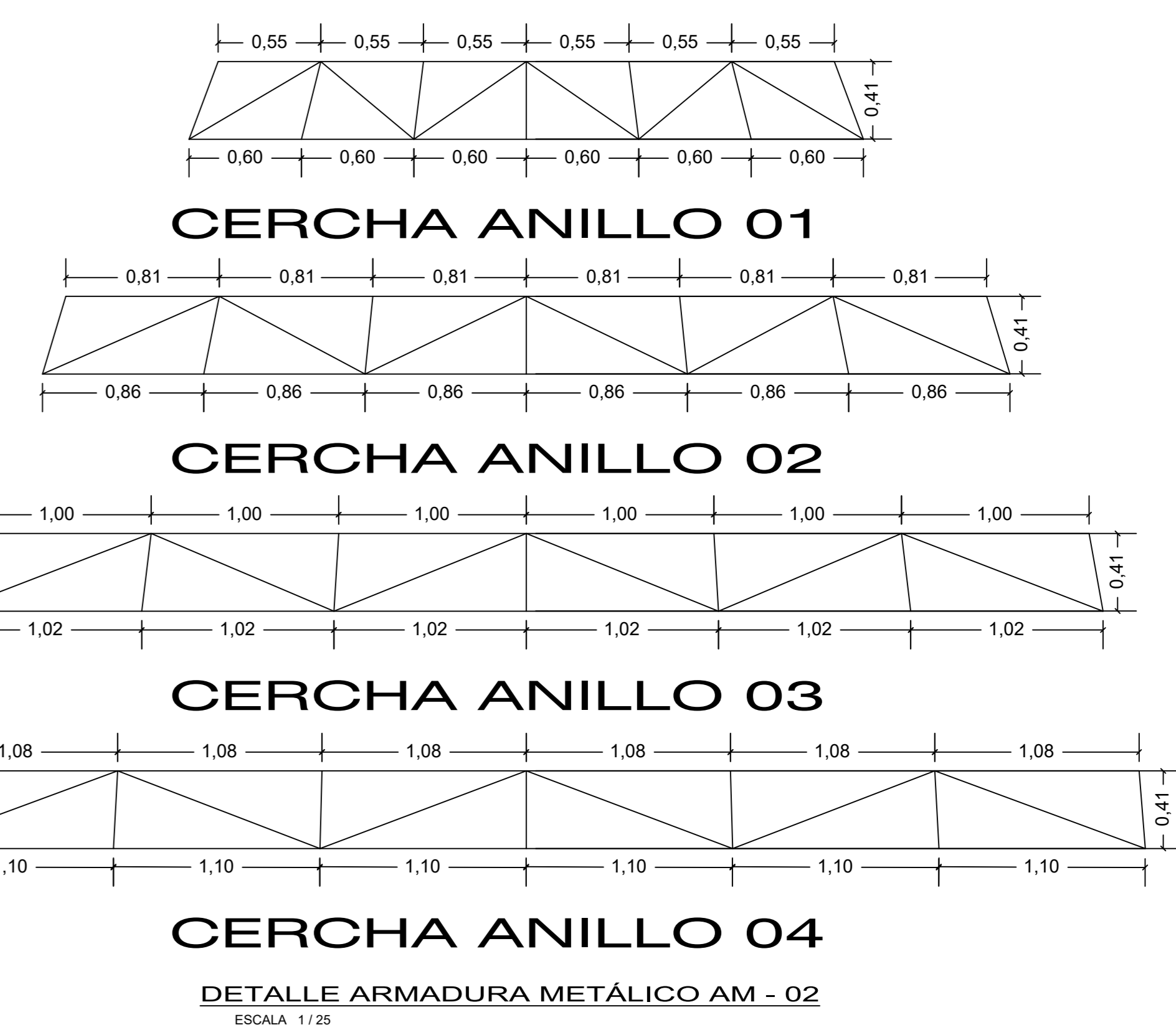
GAJO ESTRUCTURAL TIPO 1 C-I COMPOSICIÓN DE CERCHAS DE CERRAMIENTO C-CI-01
