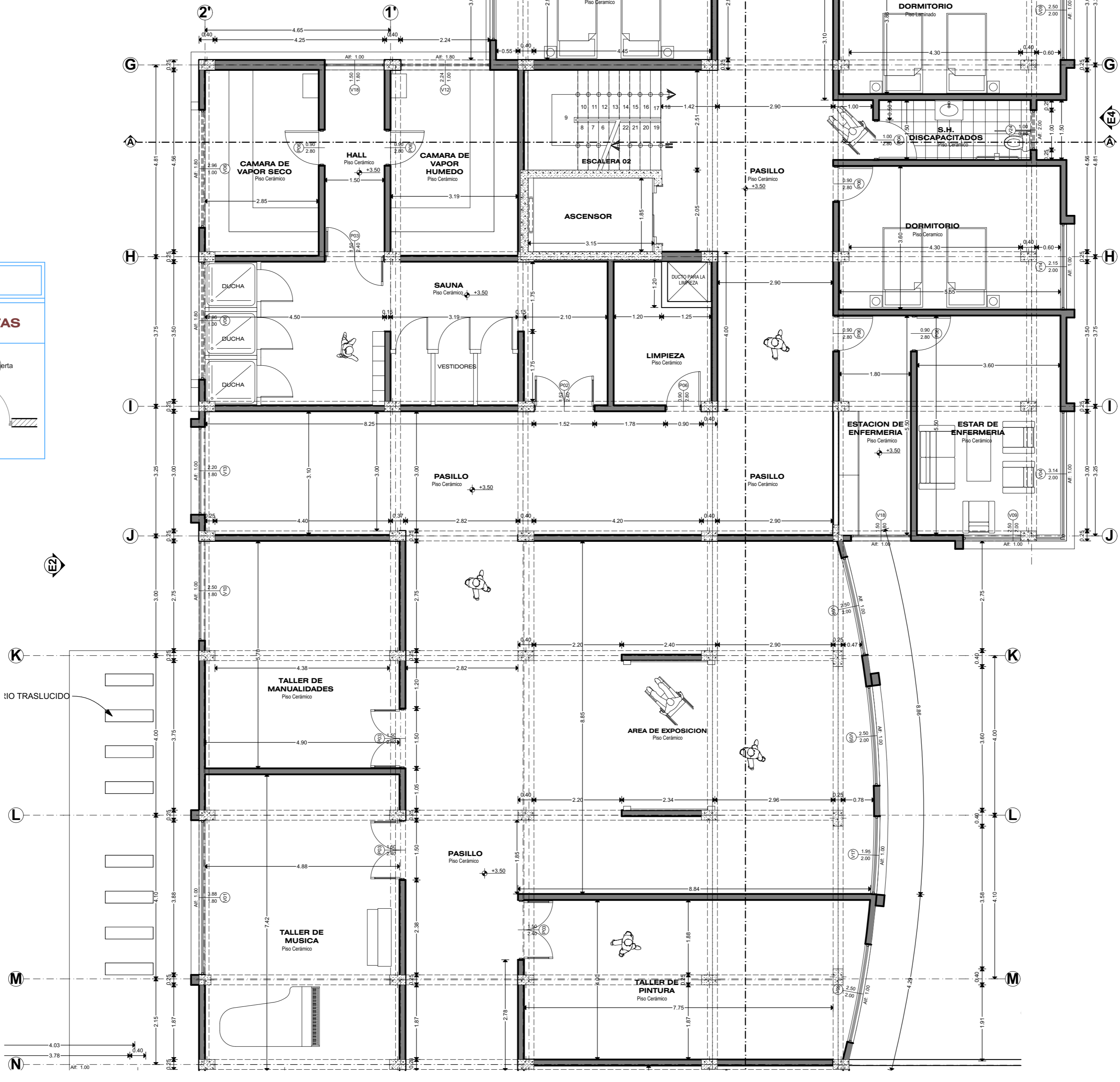
SEGUNDO NIVEL Esc: 1:75 ZONA DE SERVICIOS COMPLEMENTARIOS
